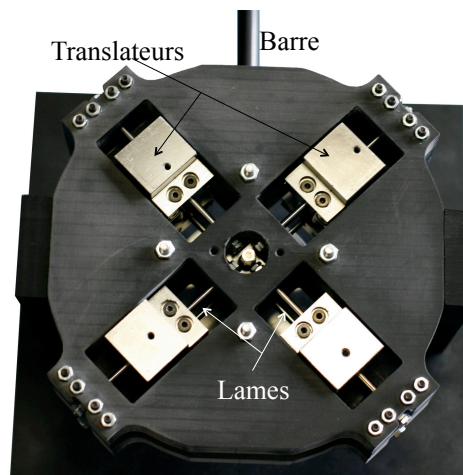
FIGURE 3.15 – Zoom sur la partie centrale, sans la spirale d'actionnement.
