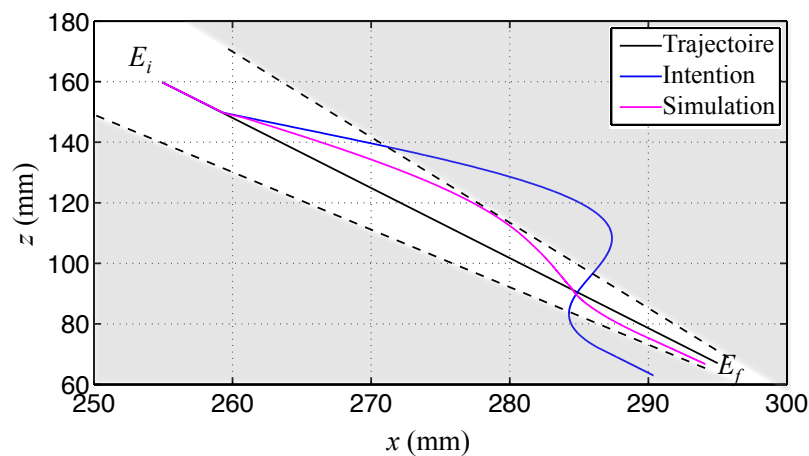
FIGURE 4.23 – Suivi de trajectoire guidé pour un cône d'effort donné.
