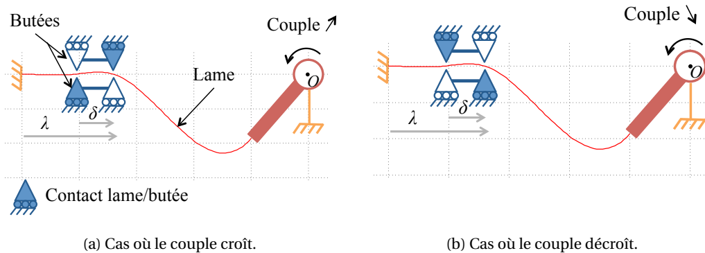
FIGURE 3.8 – Positionnement des butées et conditions de contact en fonction du couple extérieur.
