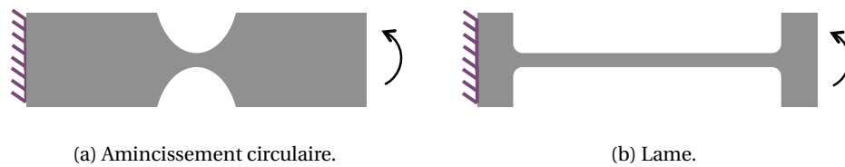
FIGURE 3.4 – Réductions de section usuelles pour la réalisation de mécanismes compliants.
