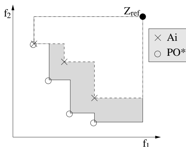
FIGURE 6.3 – Exemple en deux dimensions d’une différence d’hypervolume entre un ensemble de référence \text{PO}^* et une approximation \text{A}_i (zone grisée).
