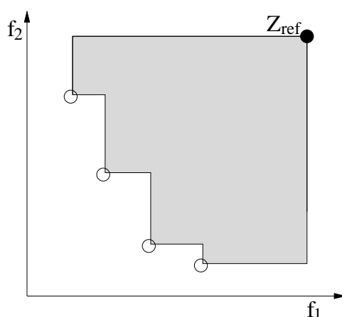
FIGURE 6.2 – Exemple en deux dimensions d’hypervolume entre un ensemble de référence \mathbf{PO}^* et un point de référence Z_{ref} (zone grisée).
