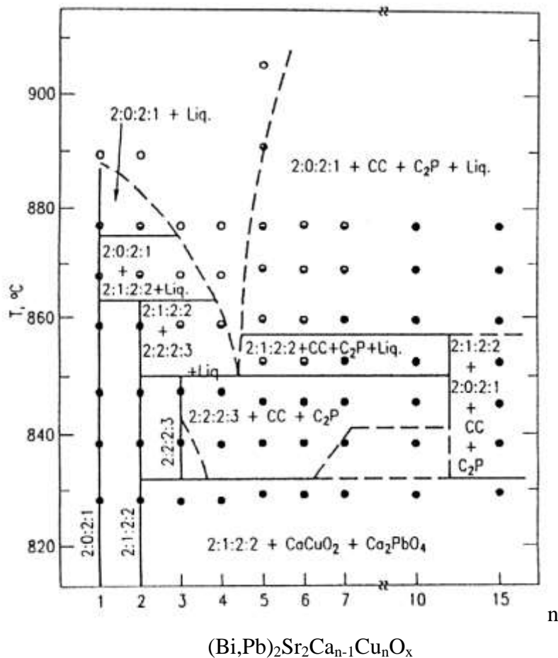
Figure 2.10 — Diagramme de phase de la famille (\text{Bi,Pb})_2\text{Sr}_2\text{Ca}_{n-1}\text{Cu}_n\text{O}_x en fonction de n , établi par Strobel et coll. [35][36] . 2:0:2:1 = (\text{Bi,Pb})_2\text{Sr}_2\text{CuO}_6 ; 2:1:2:2 = (\text{Bi,Pb})_2\text{Sr}_2\text{CaCu}_2\text{O}_6 ; CC = \text{Sr}_x\text{Ca}_{2-x}\text{CuO}_3 ; C 2 P = \text{Ca}_2\text{PbO}_4 .
