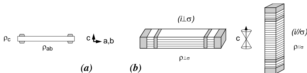
Figure 5.41 — (a) Position des contacts pour la mesure de l'anisotropie de résistivité intrinsèque des monocristaux de phases 2201 et 2212 (Montgomery) et (b) position des contacts (en grisé) sur barreaux massifs texturés 2223.
