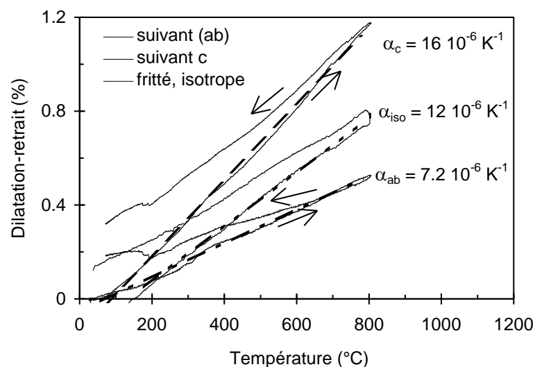
Figure 4.4 — Courbes de dilatation - retrait de deux céramiques de (\text{Bi,Pb})_2\text{Sr}_2\text{Ca}_2\text{Cu}_3\text{O}_y , l'une isotrope et l'autre texturée.
