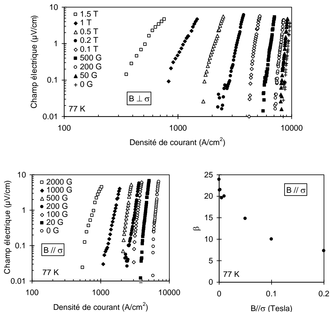
Figure 5.32 — Courbes E - J à 77\text{ K} en fonction du champ magnétique B \perp \sigma (haut) et B \parallel \sigma (gauche); Dépendance en champ B \parallel \sigma de l'exposant \beta de E = \alpha.J^\beta (droite).
