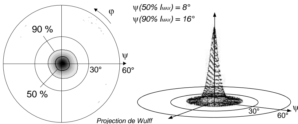
Figure 3.18 — Visualisation de l'alignement des grains en figure de pôle en diffraction des rayons X au cœur d'un disque forgé à 845°C pendant 24 heures sous 600 kg ; plans (0 0 10).
