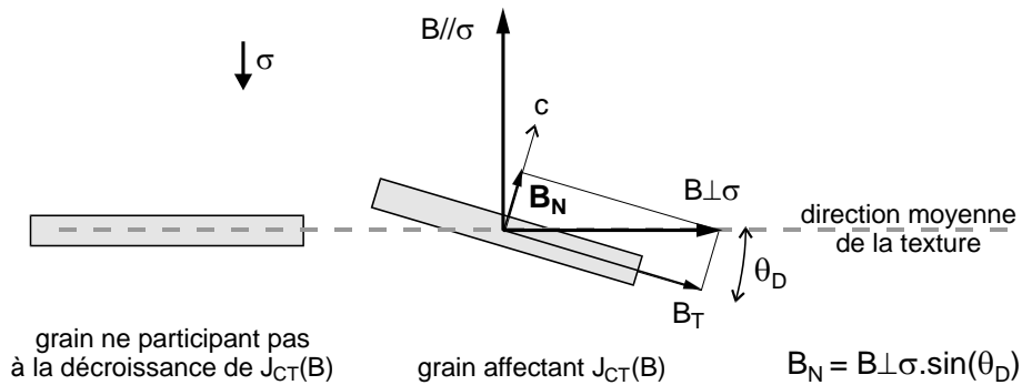
Figure 5.29 — Comparaison entre le champ magnétique global B_{\perp\sigma} appliqué et le champ magnétique B_N vu par un grain légèrement désorienté de \theta_D , responsable de la valeur de J_{CT} .
