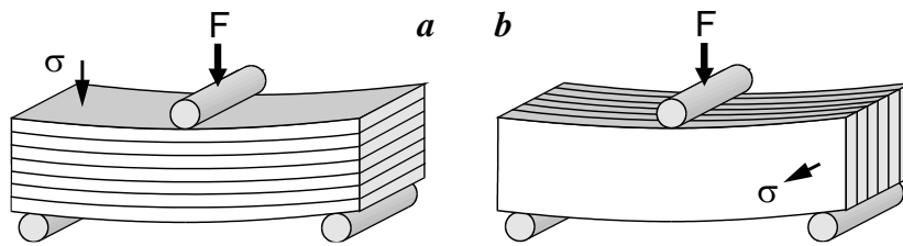
Figure 4.18 — Deux types de chargement en flexion 3 points « F \perp \sigma courant » : (a) F // \sigma dit « à plat » et (b) F \perp \sigma dit « sur chant ».
