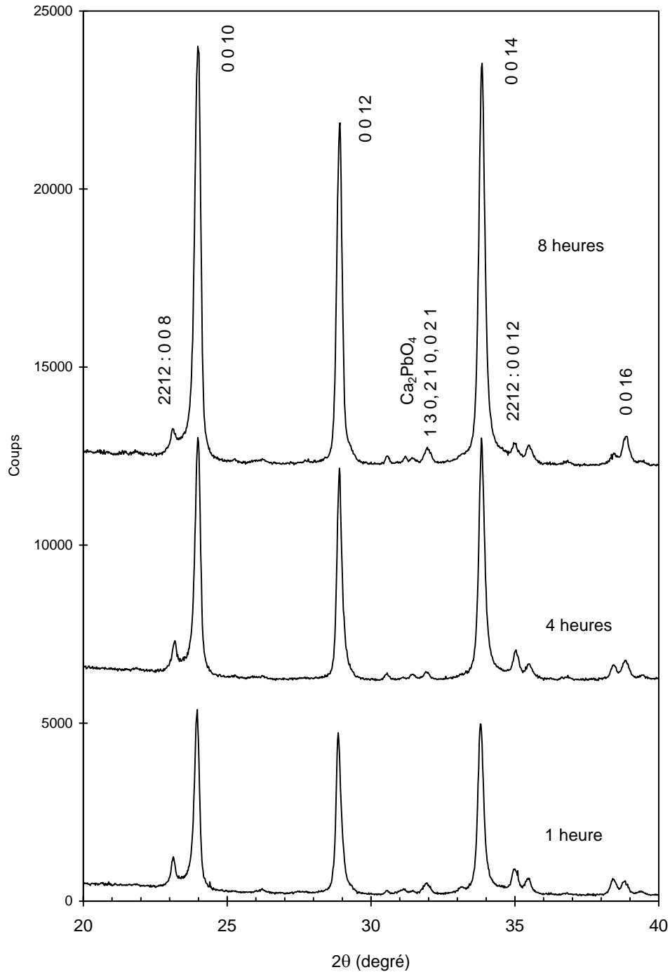
Figure 3.17 — Diffractogrammes X sur surface polie à cœur (Figure 3.16) de disques forgés à 845°C sous une charge de 600 kg pendant 1 heure, 4 heures et 8 heures.
