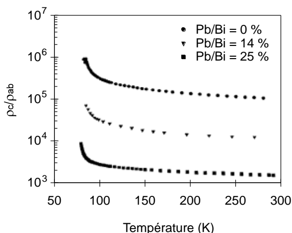
Figure 1.11 — Rapport d'anisotropie de résistivité \Gamma = \rho_c/\rho_{ab} d'un monocristal d'oxyde (Bi,Pb)_2Sr_2CaCu_2O_{8+x} suivant le dopage en plomb, d'après Régi et coll. [26] .
