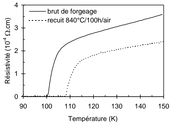
Figure 5.7 — Résistivité en fonction de la température d'un barreau non recuit.
