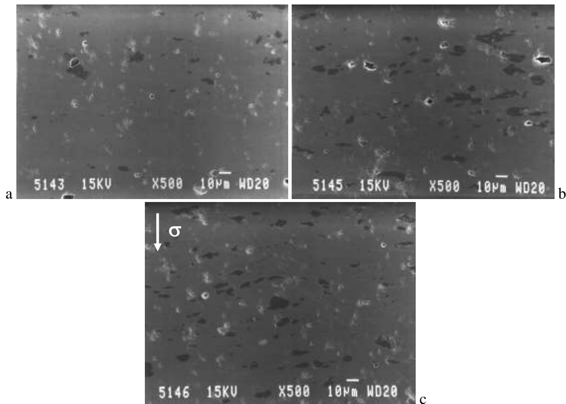
Figure 3.14 — Micrographies MEB sur sections polies de disques forgés à 850^\circ\text{C} sous 600\ \text{kg} pendant 15 minutes (a), 2 heures (b) et 4 heures (c) ; taux de phases secondaires respectifs : 1.0 % (a), 2.3 % (b) et 5.2 % (c). Notez qu'après 8 heures, la porosité – estimée à 1-2 % – diminue encore progressivement en cours de forgeage.
