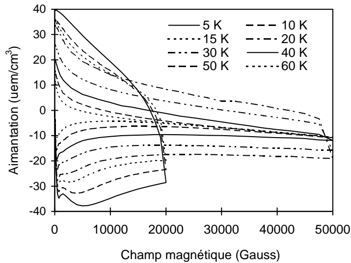
Figure 5.37 — Cycles d'aimantation en fonction de la température ( B//\sigma ). Notez le léger effet « papillon » au-dessous de 30 K (échantillon recuit sous 7,5 % \text{O}_2 )
