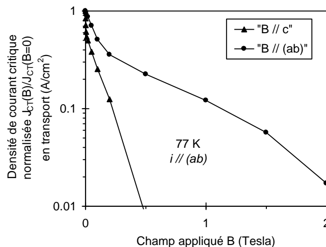
Figure 1.12 — Densité de courant critique en fonction de l'intensité du champ magnétique appliqué dans une céramique Bi-2223 à grains orientés.
