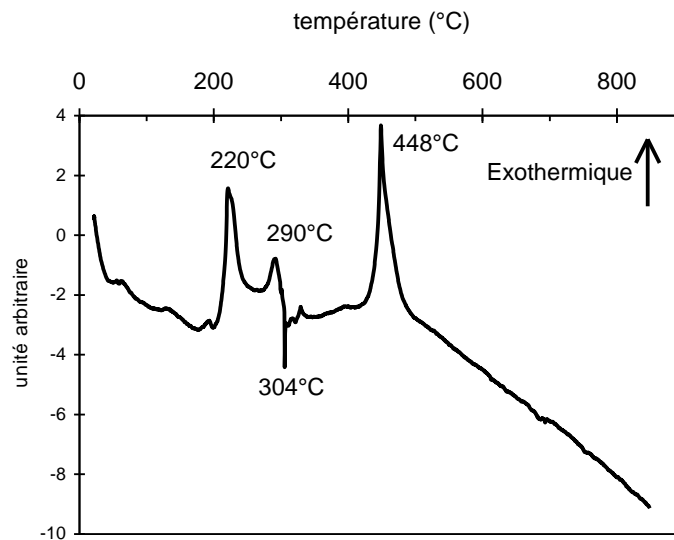
Figure 2.6 — Analyse thermique différentielle du gel.
