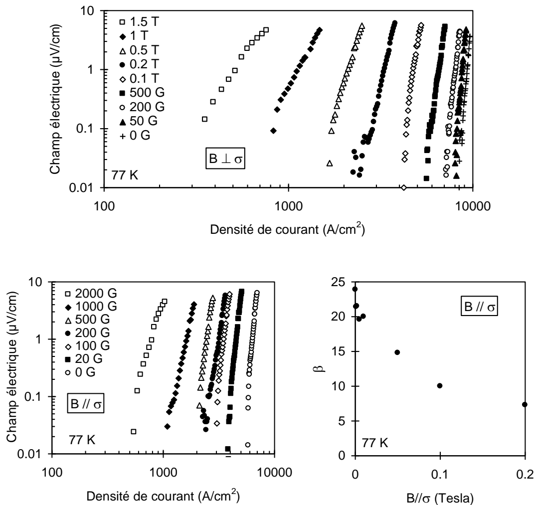
Figure 5.32 — Courbes E - J à 77 K en fonction du champ magnétique B \perp \sigma (haut) et B // \sigma (gauche) ; Dépendance en champ B // \sigma de l'exposant \beta de E = \alpha.J^\beta (droite).
