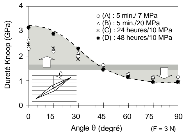
Figure 4.17 — Dureté Knoop en fonction de l'inclinaison de l'empreinte par rapport à l'axe de forgeage, pour plusieurs disques forgés sous différentes conditions de pression et temps.
