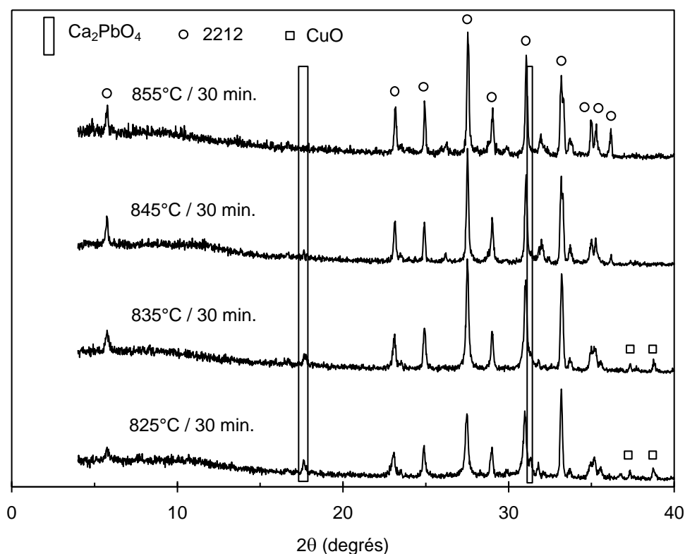
Figure 2.25 — Diffractogrammes RX des pastilles frittées 30 minutes à 825°C, 835°C, 845°C et 855°C. Evolution de la quantité de phase Ca 2 PbO 4 .
