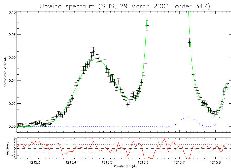
Figure 0.3: Ajustement des données par HST/STIS en 2001. Les deux plus grandes raies sont, en partant de la gauche, l'hydrogène interplanétaire et l'hydrogène géocoronal qui diffusent le rayonnement solaire Lyman-alpha. En bleu, des contaminations dues à l'oxygène géocoronal dont le triplet à 130.4 nm est transmis par d'autres ordres du réseau échelle (Vincent et al., 2011a, ApJ).
