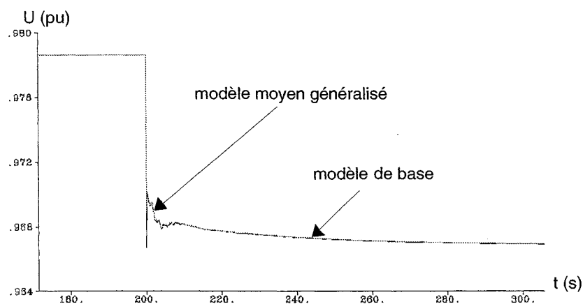
fig. IV.28 : Tension au noeud 8 - déclenchement de la ligne ligne 6-7
