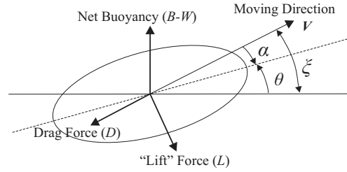
图 A.14: 上升阶段分析。
