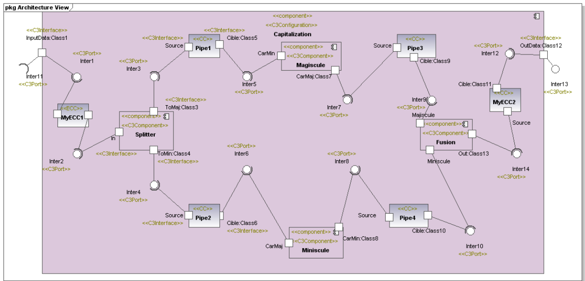
Figure A.2- Application Capitalisation en UModel.
