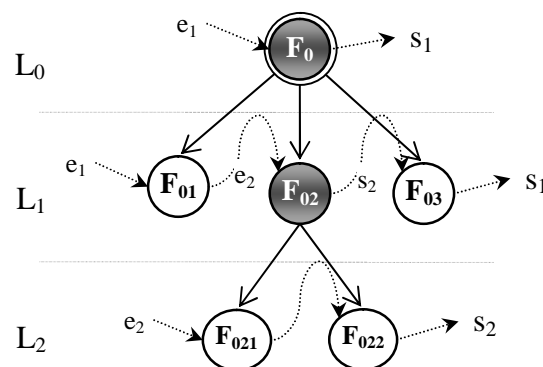
Figure 3.18- Hiérarchie fonctionnelle.
