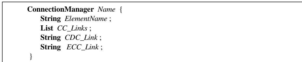
Figure 3.26- Structure du gestionnaire de connexions.
