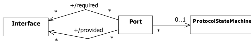
Figure 4.14- La méta-classe Port dans le méta-modèle UML2.0.
