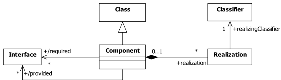
Figure 4.11- Structure de la méta-classe Component.
