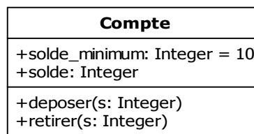
Figure 4.12 – Description de la classe compte.
