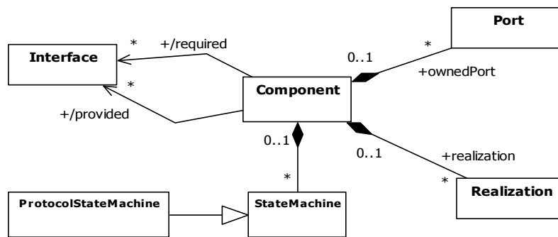
Figure 4.16- La méta-classe Component dans le méta-modèle UML2.0.
