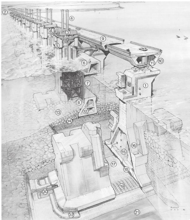
← Figure 28 : coupe technique du barrage. Source : Rijkswaterstaat, 1987
