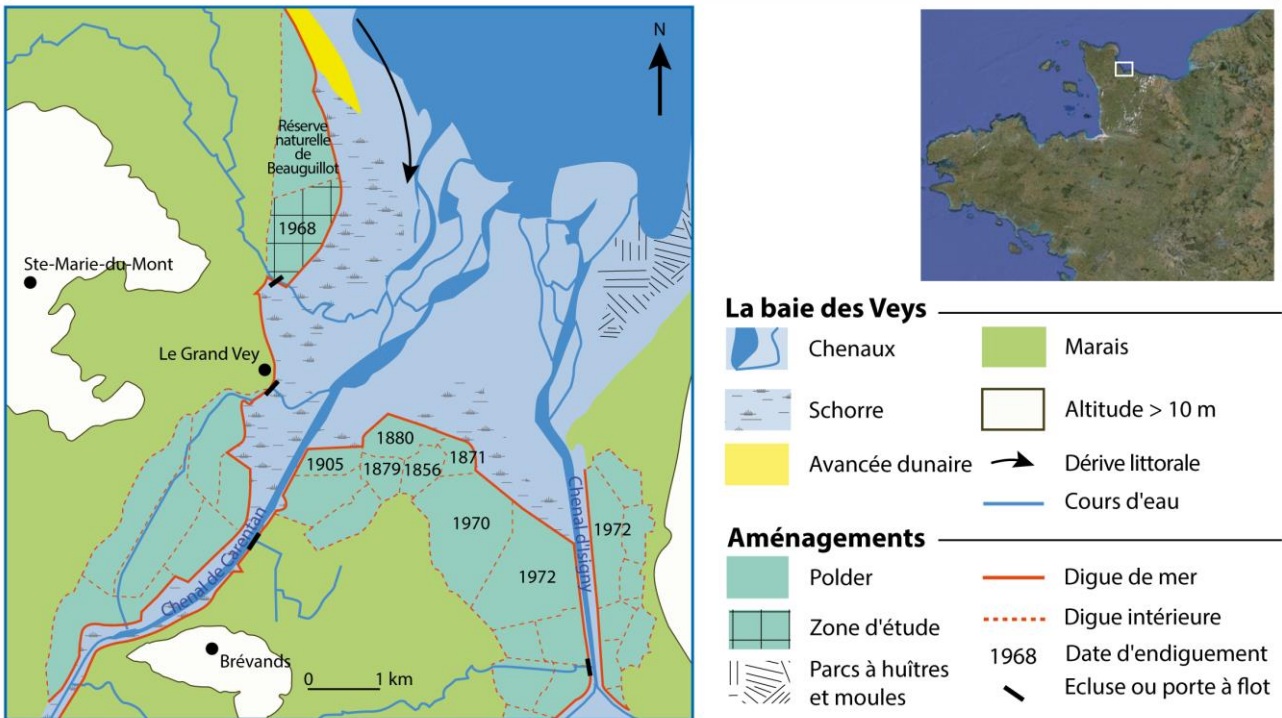
Carte 32 : Le polder de Sainte-Marie-du-Mont au sein de la baie des Veys. Sources : R. Ghirardi et F. Verger, 2009, carte topographique IGN, n° 1311 OT.
