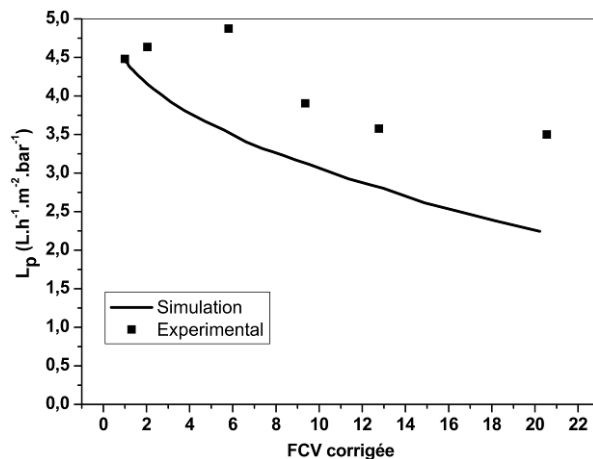
Figure 89 – Perméabilité ( L_p - L.h^{-1}.m^{-2}.bar^{-1} ) en fonction du FCV, Membrane Desal-5DL : ■/— Valeurs expérimentales/Simulation Nanoflux ® .
