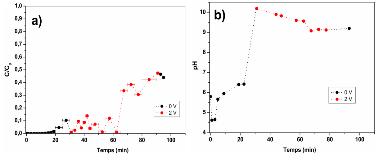
Figure 80 – Essai d'élution électrique : 0 V (●●●), 2 V (●●●). a) Courbe de percée du \text{Co}^{2+} , C_0 = 10 \text{ mg.L}^{-1} ; b) Variation du pH de la solution à la sortie de la colonne.
