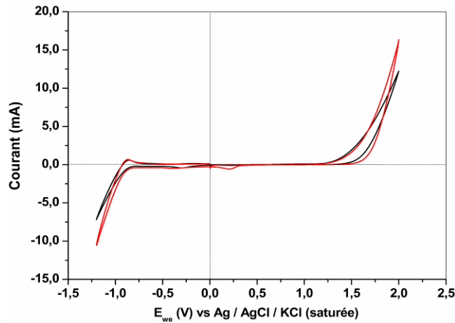
Figure 76 – Voltampérométrie cyclique, WE et CE en platine : (—) solution de \text{Na}_2\text{SO}_4 0,1 \text{ mol.L}^{-1} ; (—) mélange de \text{Na}_2\text{SO}_4 0,1 \text{ mol.L}^{-1} et \text{NaNO}_3 0,2 \text{ mol.L}^{-1} .
