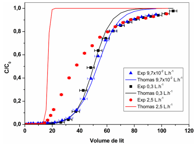
Figure 62 – Influence du débit de circulation dans les courbes de percée du \text{Co}^{2+} . C_0 = 1,5 \times 10^{-4} \text{ mol.L}^{-1} ; \text{pH} = 5,8 ; Volume du lit = 4,6 mL ; Dispositif en colonne ; masse de feutres de carbone \approx 1,2 \text{ g} ; Points expérimentaux/Modèle de Thomas : 9,7 \times 10^{-2} \text{ L.h}^{-1} — / ▲ ; 0,3 \text{ L.h}^{-1} — / ■ ; 2,5 \text{ L.h}^{-1} — / ●.
