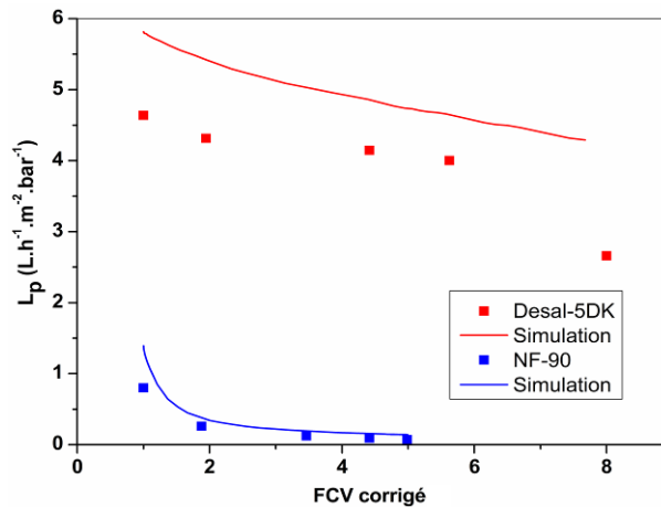
Figure 23 – Comparaison entre la simulation et les résultats expérimentaux de la variation de L_p en fonction du FCV. Valeurs expérimentales/Simulation Nanoflux ® : membrane Desal-5DK (■/—) et membrane NF-90 (■/—).
