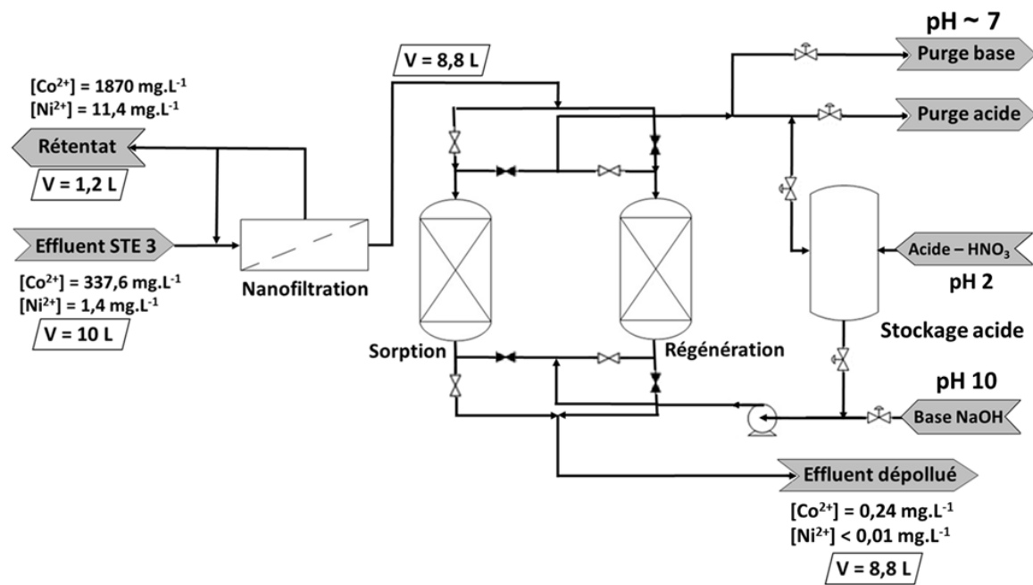
Figure 68 – Schéma de procédé simplifié pour le traitement de la solution STE3. Vanne ouverte : ▷◁ ; Vanne fermée ►◀ .
