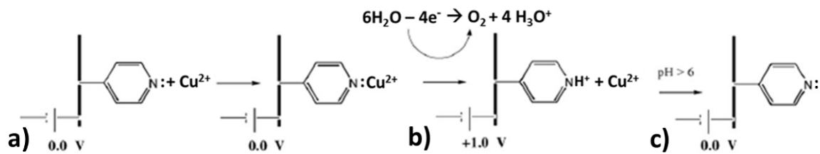
Figure 73 – Régénération électrique de la P4VP d'après [18]. a) complexation des cations Cu 2+ par la pyridine ; b) éluion électrique et création de l'ion pyridinium ; c) retour spontanée à la forme pyridine en absence de courant électrique.
