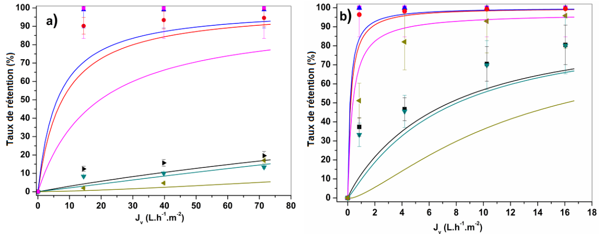
Figure 22 – TR en fonction de la densité de flux ( J_v - \text{L.h}^{-1}.\text{m}^{-2}.\text{bar}^{-1} ); Simulations à pH acide . Prévission/Données expérimentales: -/● \text{Co}^{2+} , -/▲ \text{Ni}^{2+} , -/■ \text{SO}_4^{2-} , -/▼ \text{NO}_3^- , -/◄ \text{NO}_2^- et -/■ \text{Na}^+ . a) Membrane Desal-5DK ; pH = 3,2 ; Ajustement à la solution de \text{NaNO}_3 : X_i = -0,082 ; L_{\text{eff}} = 0,374 \mu\text{m} ; r_p = 0,44 \text{ nm} , L_p^0 = 7,8 (\text{L.h}^{-1}.\text{m}^{-2}.\text{bar}^{-1}) ; Ecart : 5,94 %. b) Membrane Dow NF-90 ; pH = 3,8 ; Ajustement à la solution de \text{NaNO}_3 : X_i = -0,09 ; L_{\text{eff}} = 12,406 \mu\text{m} ; r_p = 0,42 \text{ nm} , L_p^0 = 5,7 (\text{L.h}^{-1}.\text{m}^{-2}.\text{bar}^{-1}) ; Ecart : 7,4 %.
