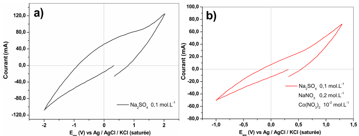
Figure 77 – Voltampérométrie cyclique. Montage électrochimique de base. WE : feutre de carbone FNG et CE : platine. Vitesse de balayage : 10 \text{ mV.s}^{-1} . a) électrolyte : solution de
