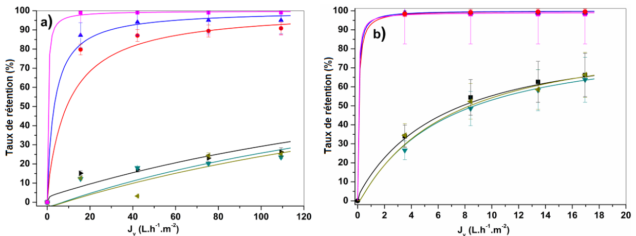
Figure 19 – TR en fonction de la densité de flux ( J_v - \text{L.h}^{-1}.\text{m}^{-2} ). Ajustement à l'effluent ; Préviation/Données expérimentales : \text{---}/\bullet \text{Co}^{2+} , \text{---}/\blacktriangle \text{Ni}^{2+} , \text{---}/\blacksquare \text{SO}_4^{2-} , \text{---}/\blacktriangledown \text{NO}_3^- , \text{---}/\blacktriangleleft \text{NO}_2^- et \text{---}/\blacktriangleright \text{Na}^+ . a) Membrane Desal 5-DK ; pH = 6,2 ; X_i = -0,063 ; L_{\text{eff}} = 0,661 \mu\text{m} ; K_{\text{Born}} présentés au Tableau 17 ; r_p = 0,44 \text{ nm} , L_p^0 = 8 (\text{L.h}^{-1}.\text{m}^{-2}.\text{bar}^{-1}) ; Ecart : 1,2%. b) Membrane NF-90 ; pH = 6,2 ; X_i = -0,04 ; L_{\text{eff}} = 21,06 \mu\text{m} , K_{\text{Born}} présentés au Tableau 17 ; r_p = 0,42 \text{ nm} , L_p^0 = 5,7 (\text{L.h}^{-1}.\text{m}^{-2}.\text{bar}^{-1}) ; Ecart : 0,4%.
