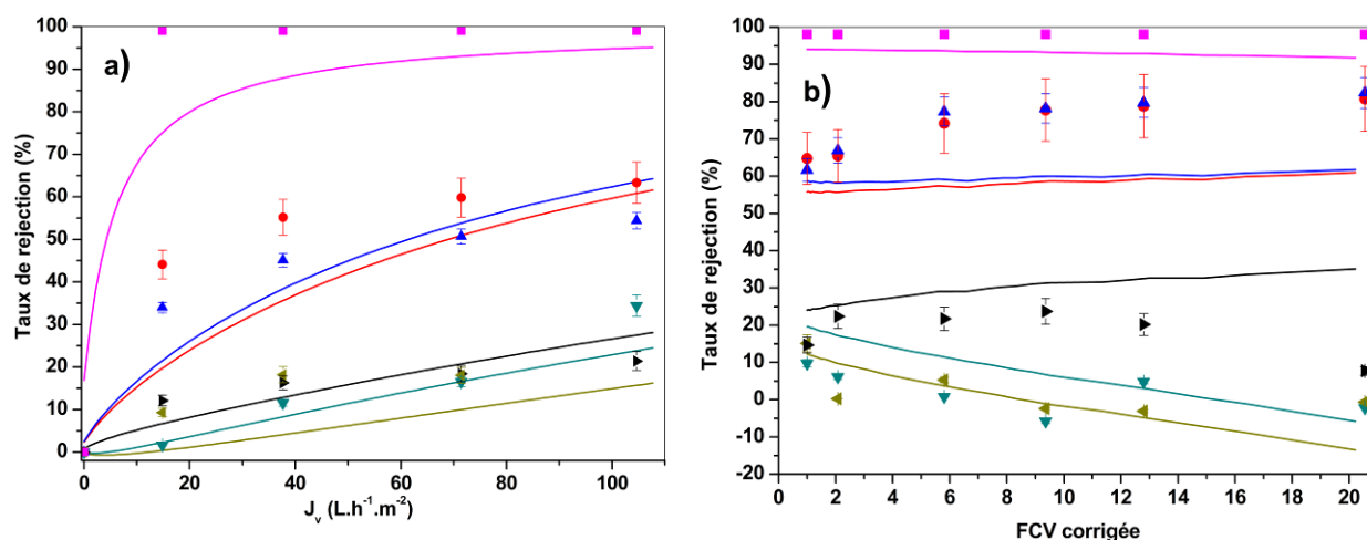
Figure 87 – Evolution du TR au cours de la filtration de l'effluent synthétique ; Membrane Desal-5DL ; pH = 6,2 ; Ajustement à la solution de NaNO 3 : X_i = -0,841 ; L_{eff} = 0,426 \mu\text{m} ; K_{Born} calculés (chap. II § 3.3.1) ; r_p 0,58 nm, L_p^0 5,8 (L.h -1 .m -2 .bar -1 ) ; Prévission Nanoflux®/Données expérimentales : —/● Co 2+ , —/▲ Ni 2+ , —/■ SO 4 2- , —/▼ NO 3 - , —/◀ NO 2 - ; —/▶ Na + ; a) volume constante, écart = 2,4% ; b) concentration volumique.
