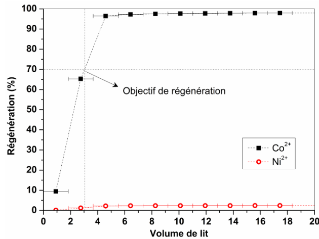
Figure 67 – Profil de la régénération acide d'une colonne saturée: Ni 2+ ○ ; Co 2+ ■. pH de la solution d'éluée = 2. Colonne en verre, volume du lit = 5,5 mL; masse de feutre de carbone = 1 g; Débit = 0,3 L.h -1 .
