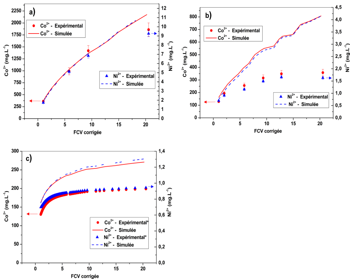
Figure 88 – Concentration des cations divalents en solution en fonction du FCV corrigé. Membrane Desal-5DL. Simulation Nanoflux ® /Données expérimentales : —/● Co 2+ , - - -/▲ Ni 2+ : a) Rétentat ; b) Permétat instantané ; c) Permétat Moyen.
