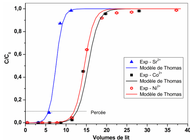
Figure 63 – Courbes de percée de solutions individuelles de \text{Co}^{2+} , \text{Ni}^{2+} et \text{Sr}^{2+} . Points expérimentaux/Modèle de Thomas: \text{Ni}^{2+} \circ /—, C_0 = 8,5 \times 10^{-4} \text{ mol.L}^{-1} , \text{pH} = 5,85 ; \text{Co}^{2+} \blacksquare /—, C_0 = 8,4 \times 10^{-4} \text{ mol.L}^{-1} , \text{pH} = 5,84 ; \text{Sr}^{2+} \blacktriangle /—, C_0 = 8,5 \times 10^{-4} \text{ mol.L}^{-1} , \text{pH} = 5,80 ; Colonne en verre, volume du lit = 5,5 \text{ mL} ; Masse de feutres de carbone = 1 \text{ g} ; Débit = 0,3 \text{ L.h}^{-1} .
