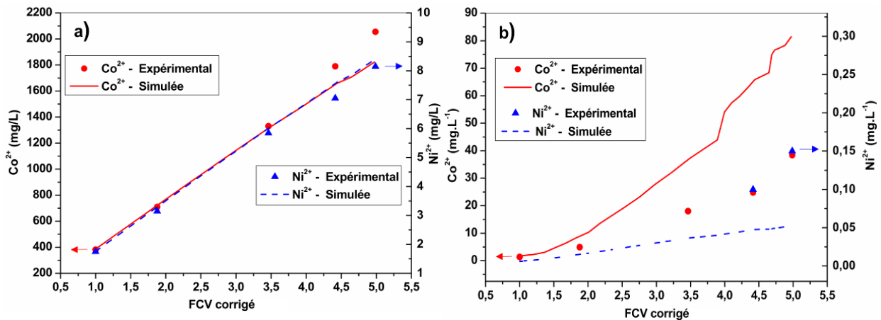
Figure 28 – Concentration des cations divalents en solution en fonction du FCV corrigé. Membrane NF-90 . Simulation Nanoflux®/Données expérimentales : —/● Co 2+ , - - -/▲ Ni 2+ : a) Rétentat ; b) Perméat instantané ([Ni 2+ ] < 0,1 mg.L -1 pour FCV = 1, 1,8 et 3,5).
