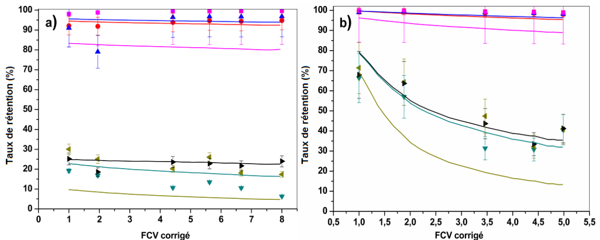
Figure 24 – TR ionique en fonction du FCV corrigé; Ajustement à la solution de NaNO_3 ; Simulation Nanoflux ® /Données expérimentales : Co^{2+} (—/●), Ni^{2+} (—/▲), SO_4^{2-} (—/■), NO_3^- (—/▼), NO_2^- —/◄ et Na^+ —/►. a) Membrane Desal-5DK ; pH = 6,4 X_i = -0,082 ; L_{eff} = 0,374 \mu m ; K_{Borm} calculés ; r_p 0,44 nm, L_p^0 8,1 ( L \cdot h^{-1} \cdot m^2 \cdot bar^{-1} ) ; b) Membrane NF-90 ; pH = 6,2 ; X_i = -0,090 ; L_{eff} = 12,406 \mu m ; K_{Borm} calculés ; r_p = 0,42 nm, L_p^0 5,76 ( L \cdot h^{-1} \cdot m^2 \cdot bar^{-1} ).
