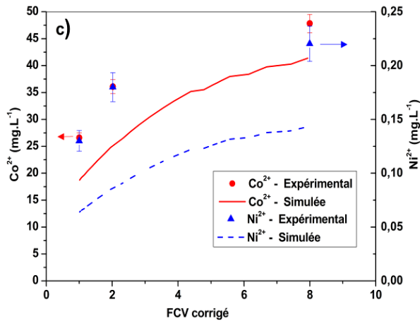
Figure 27 – Concentration des cations divalents en solution en fonction du FCV corrigé. Membrane Desal-5DK . Simulation Nanoflux®/Données expérimentales : —/● Co 2+ , - - -/▲ Ni 2+ . a) Rétentat ; b) Perméat instantané ; c) Perméat Moyen.
