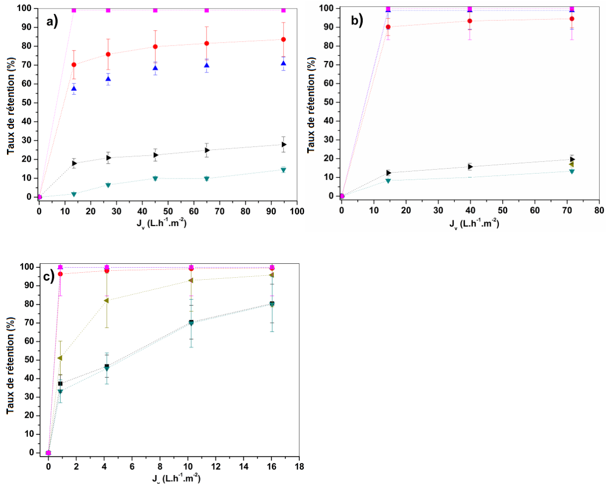
Figure 15 – Evolution du TR de l'effluent à pH acide en fonction de J_v . Valeur expérimentale: ● Co^{2+} , ▲ Ni^{2+} , ■ SO_4^{2-} , ▼ NO_3^- , ◀ NO_2^- et ► Na^+ ; a) Membrane Desal-5DL, pH = 3,2; b) Membrane Desal-5DK, pH = 3,2; c) Membrane Dow NF-90, pH = 3,8.
