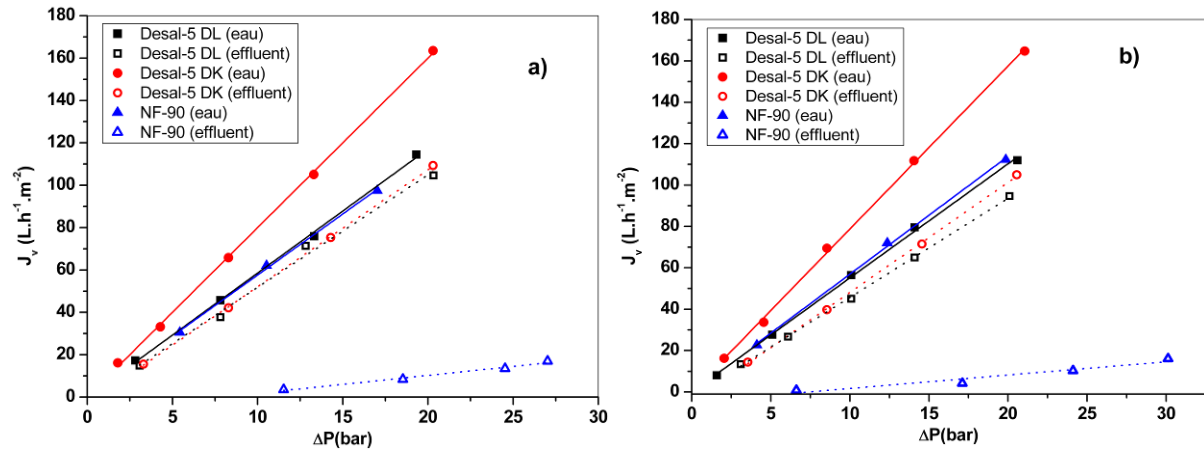
Figure 13 – Variation de J_v en fonction de \Delta P pour les membranes étudiées. Symboles pleins : filtration à l'eau ; symboles ouverts : filtration de l'effluent. Desal-5DL: ■, □; Desal-5DK: ●, ○; NF-90: ▲, △. a) pH naturel et b) pH acide.
