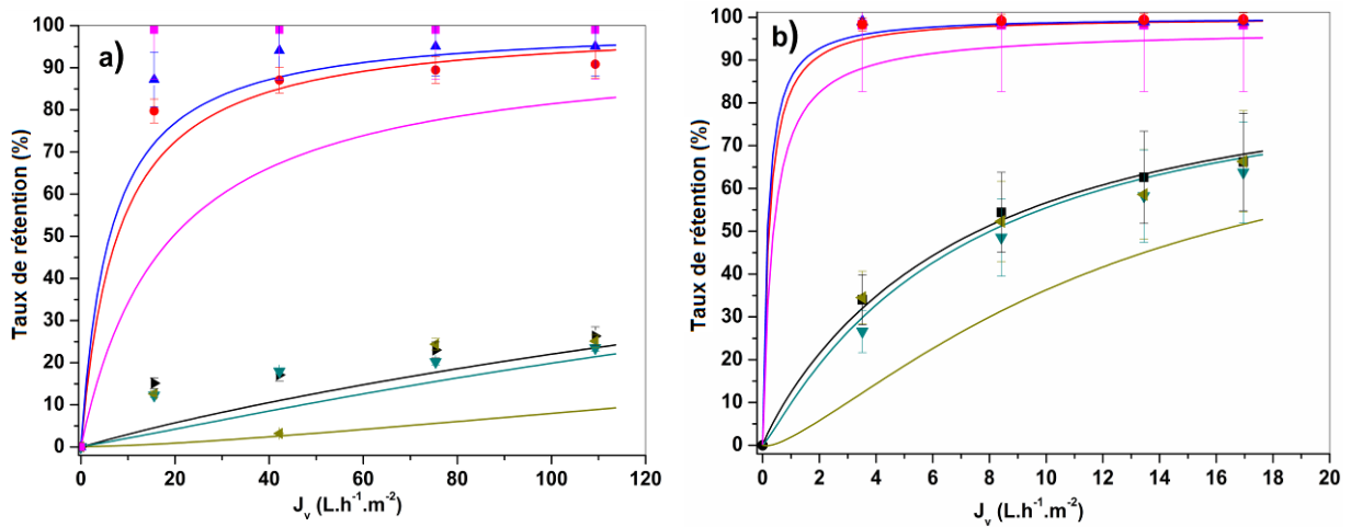
Figure 20 – TR en fonction de la densité de flux ( J_v - L.h^{-1}.m^{-2} ) ; Ajustement à la solution de NaNO_3 ; Préviation/Données expérimentales : -/\bullet Co^{2+} , -/\blacktriangle Ni^{2+} , -/\blacksquare SO_4^{2-} , -/\blacktriangledown NO_3^- , -/\blacktriangleleft NO_2^- et -/\blacktriangleright Na^+ . a) Membrane Desal 5-DK ; pH = 6,2 ; X_i = -0,082 ; L_{eff} = 0,374 \mu m ; K_{Bom} présentés au Tableau 19 ; r_p = 0,44 nm , L_p^0 8 (L.h^{-1}.m^{-2}.bar^{-1}) ; Ecart : 2,4%. b) Membrane NF-90 ; pH = 6,2 ; X_i = -0,09 ; L_{eff} = 12,406 \mu m ; K_{Bom} présentés au Tableau 19 ; r_p = 0,42 nm , L_p^0 5,76 (L.h^{-1}.m^{-2}.bar^{-1}) ; Ecart : 2,3%.
