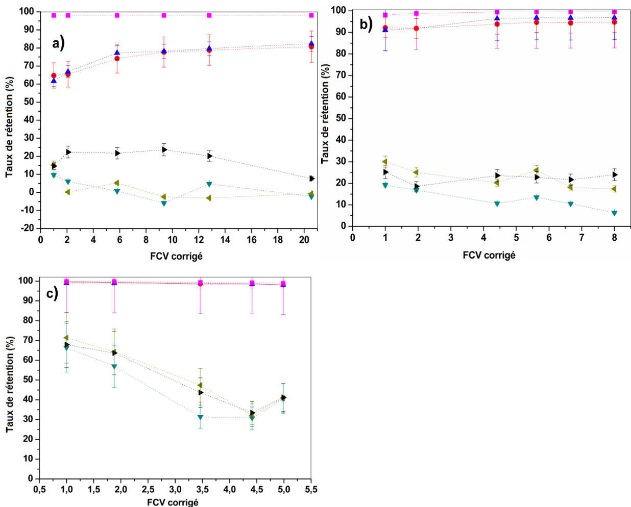
Figure 17 – T.R en fonction de FCV corrigé. Données expérimentales: ● Co 2+ , ▲ Ni 2+ , ■ SO 4 2- , ▼ NO 3 - , ◀ NO 2 - et ► Na + . a) Membrane Desal-5DL ; pH = 6,2 ; b) Membrane Desal-5DK ; pH = 6,4 ; c) Membrane NF-90 ; pH = 6,3
