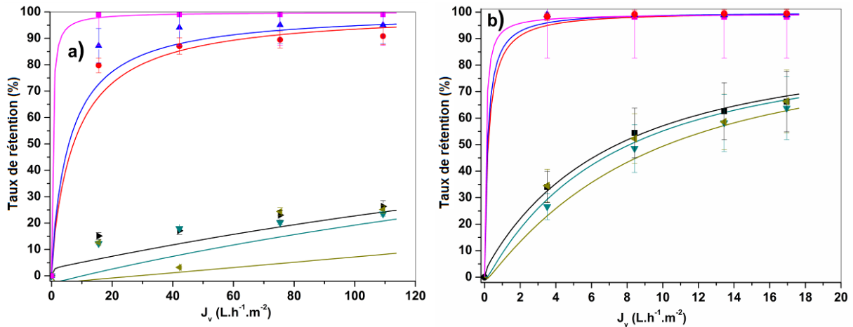
Figure 21 – TR en fonction de la densité de flux ( J_v - \text{L.h}^{-1}.\text{m}^{-2}.\text{bar}^{-1} ) ; X_i et L_{\text{eff}} ajustés à la solution de \text{NaNO}_3 , K_{\text{Born}} ajusté à l'effluent. Prédiction/Données expérimentales : —/● \text{Co}^{2+} , —/▲ \text{Ni}^{2+} , —/■ \text{SO}_4^{2-} , —/▼ \text{NO}_3^- , —/◀ \text{NO}_2^- et —/▶ \text{Na}^+ : a) Membrane Desal 5-DK ; pH = 6,2 ; X_i = -0,082 ; L_{\text{eff}} = 0,374 \mu\text{m} ; K_{\text{Born}} \text{SO}_4^{2-} = 0,0045 ; r_p = 0,44 \text{ nm} , L_p^0 8 (\text{L.h}^{-1}.\text{m}^{-2}.\text{bar}^{-1}) ; Ecart \text{SO}_4^{2-} : 0,60% ; K_{\text{Born}} \text{NO}_2^- = 0,38 ; Ecart \text{NO}_2^- : 6,01%. b) Membrane NF-90 ; pH = 6,2 ; X_i = -0,090 ; L_{\text{eff}} = 12,406 \mu\text{m} ; K_{\text{Born}} \text{SO}_4^{2-} = 0,05 ; r_p = 0,42 \text{ nm} , L_p^0 5,76 (\text{L.h}^{-1}.\text{m}^{-2}.\text{bar}^{-1}) ; Ecart \text{SO}_4^{2-} : 1,56% ; K_{\text{Born}} \text{NO}_2^- = 0,48 ; Ecart \text{NO}_2^- : 5,95%.
