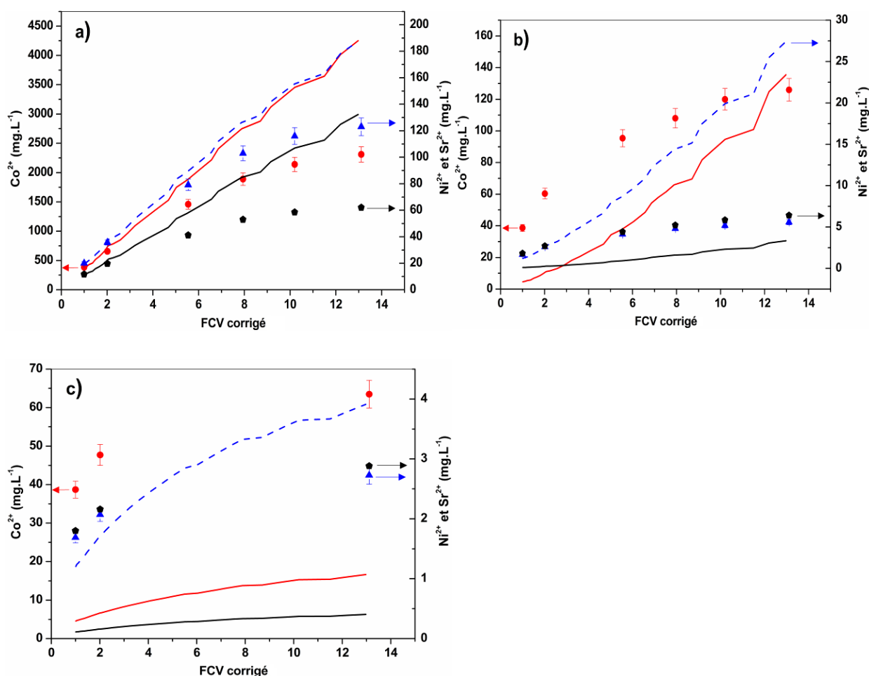
Figure 90 – Concentration des cations divalents en solution en fonction du FCV corrigé pour l'effluent à 8 ions. Membrane Desal-5DK. Simulation Nanoflux®/Données expérimentales : —/● \text{Co}^{2+} , - - -/▲ \text{Ni}^{2+} , —/■ \text{Sr}^{2+} : a) Rétentat ; b) Perméat instantané ; c) Perméat Moyen.
