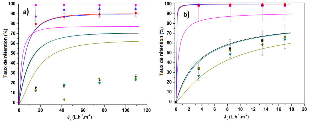
Figure 18 – TR en fonction de la densité de flux ( J_v - L.h^{-1}.m^{-2} ). X_i et L_{eff} à priori ; Prédiction/Données expérimentales : \text{---}/\bullet Co^{2+} , \text{---}/\blacktriangle Ni^{2+} , \text{---}/\blacksquare SO_4^{2-} , \text{---}/\blacktriangledown NO_3^- , \text{---}/\blacktriangleleft NO_2^- et \text{---}/\blacktriangleright Na^+ . ; a) Membrane Desal-5DK; pH = 6,2 ; X_i = -0,346 ; L_{eff} = 20,145 \mu m ; K_{Born} = 1 ; r_p = 0,44 \text{ nm} , L_p^0 = 8 (L.h^{-1}.m^{-2}.bar^{-1}) . Ecart : 8,5%. b) Membrane NF-90; pH = 6,2 ; X_i = 0,047 ; L_{eff} = 36,90 \mu m , K_{Born} = 1 ; r_p = 0,42 \text{ nm} , L_p^0 = 5,76 (L.h^{-1}.m^{-2}.bar^{-1}) . Ecart : 1,8 %.
