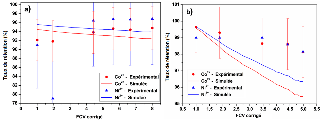
Figure 25 – TR des cations divalents en fonction du FCV corrigé; Ajustement à la solution de NaNO 3 ; Simulation Nanoflux®/Données expérimentales : Co 2+ (—/●), Ni 2+ (—/▲). a) Membrane Desal-5DK ; b) Membrane NF-90.
