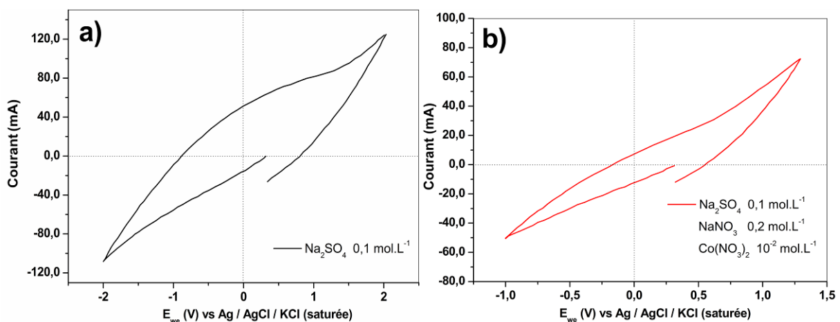
Figure 77 – Voltampéromme cyclique. Montage électrochimique de base. WE : feutre de carbone FNG et CE : platine. Vitesse de balayage : 10 \text{ mV.s}^{-1} . a) électrolyte : solution de
