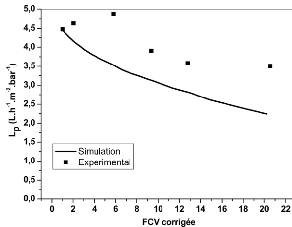
Figure 89 – Perméabilité ( L_p - L \cdot h^{-1} \cdot m^2 \cdot bar^{-1} ) en fonction du FCV, Membrane Desal-5DL : ■/— Valeurs expérimentales/Simulation Nanoflux ® .
