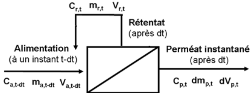
Figure 10 – Représentation d'un pas pour la simulation de la nanofiltration en concentration volumique.
