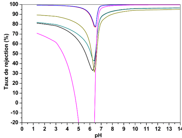
Figure 11 – T.R en fonction du pH de l'effluent. \Delta P = 21 bar et T = 25^\circ\text{C} . — \text{Co}^{2+} , — \text{Ni}^{2+} , — \text{SO}_4^{2-} , — \text{NO}_3^- , — \text{NO}_2^- et — \text{Na}^+ . Membrane Dow NF-90 , r_p 0,42 nm, and L_p^0 5,3 ( \text{L}/(\text{h}.\text{m}^2.\text{bar}) ) ; K_{\text{Born}} = 1 ; L_{\text{eff}} et X_m fournis par Nanoflux à priori.
