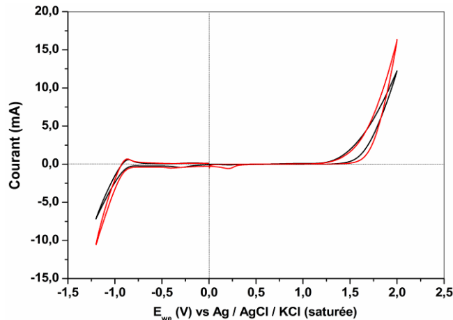
Figure 76 – Voltampéromme cyclique, WE et CE en platine : (—) solution de \text{Na}_2\text{SO}_4 0,1 \text{ mol.L}^{-1} ; (—) mélange de \text{Na}_2\text{SO}_4 0,1 \text{ mol.L}^{-1} et \text{NaNO}_3 0,2 \text{ mol.L}^{-1} .
