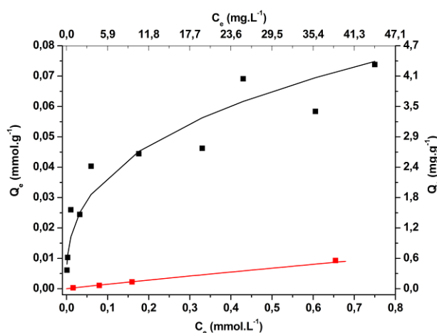
Figure 48 – Comparaison des isothermes de sorption du \text{Co}^{2+} sur les feutres de carbone non greffés. Données expérimentales / isotherme de Freundlich : (■/—) pH 2 et (●/—) pH naturel (5,8).
