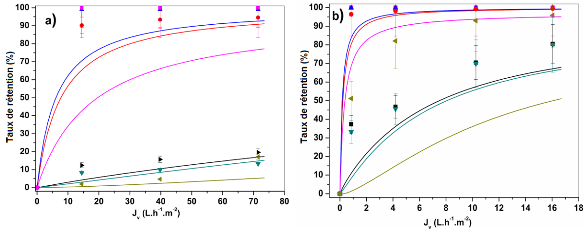
Figure 22 – TR en fonction de la densité de flux ( J_v - \text{L.h}^{-1}.\text{m}^{-2}.\text{bar}^{-1} ); Simulations à pH acide . Préviation/Données expérimentales: -/● \text{Co}^{2+} , -/▲ \text{Ni}^{2+} , -/■ \text{SO}_4^{2-} , -/▼ \text{NO}_3^- , -/◄ \text{NO}_2^- et -/■ \text{Na}^+ . a) Membrane Desal-5DK ; pH = 3,2 ; Ajustement à la solution de \text{NaNO}_3 : X_i = -0,082 ; L_{\text{eff}} = 0,374 \mu\text{m} ; r_p = 0,44 \text{ nm} , L_p^0 = 7,8 (\text{L.h}^{-1}.\text{m}^{-2}.\text{bar}^{-1}) ; Ecart : 5,94 %. b) Membrane Dow NF-90 ; pH = 3,8 ; Ajustement à la solution de \text{NaNO}_3 : X_i = -0,09 ; L_{\text{eff}} = 12,406 \mu\text{m} ; r_p = 0,42 \text{ nm} , L_p^0 = 5,7 (\text{L.h}^{-1}.\text{m}^{-2}.\text{bar}^{-1}) ; Ecart : 7,4 %.
