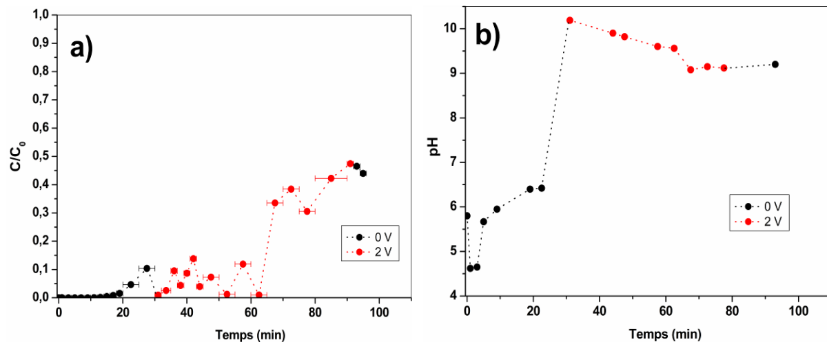
Figure 80 – Essai d'éluion électrique : 0 V (●●●), 2 V (●●●). a) Courbe de percée du \text{Co}^{2+} , C_0 = 10 \text{ mg.L}^{-1} ; b) Variation du pH de la solution à la sortie de la colonne.
