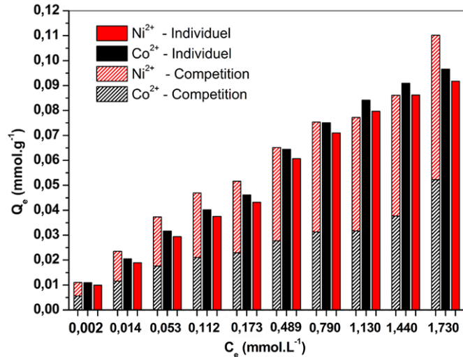
Figure 52 – Capacités de sorption des ions Co 2+ et Ni 2+ sur feutre de carbone non greffé. Co 2+ en solution individuelle (■) ; Ni 2+ en solution individuelle (■) ; Co 2+ en mélange (▨) ; Ni 2+ en mélange (▨).
