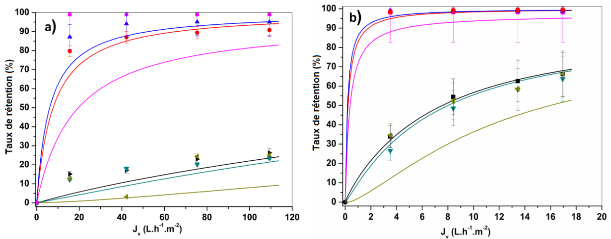
Figure 20 – TR en fonction de la densité de flux ( J_v - L.h^{-1}.m^{-2} ) ; Ajustement à la solution de NaNO_3 ; Préviation/Données expérimentales : —/● Co^{2+} , —/▲ Ni^{2+} , —/■ SO_4^{2-} , —/▼ NO_3^- , —/◄ NO_2^- et —/► Na^+ . a) Membrane Desal 5-DK ; pH = 6,2 ; X_i = -0,082 ; L_{eff} = 0,374 \mu m ; K_{Bom} présentés au Tableau 19 ; r_p = 0,44 \text{ nm} , L_p^0 = 8 (L.h^{-1}.m^{-2}.bar^{-1}) ; Ecart : 2,4%. b) Membrane NF-90 ; pH = 6,2 ; X_i = -0,09 ; L_{eff} = 12,406 \mu m ; K_{Bom} présentés au Tableau 19 ; r_p = 0,42 \text{ nm} , L_p^0 = 5,76 (L.h^{-1}.m^{-2}.bar^{-1}) ; Ecart : 2,3%.
