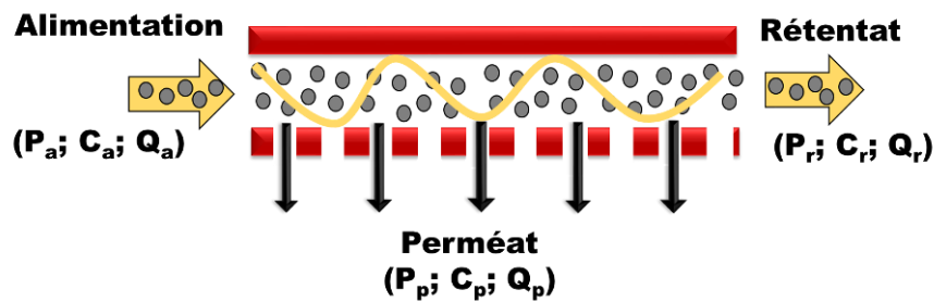
Figure 3 – La filtration tangentielle dans le cas d'une rétention ionique.
