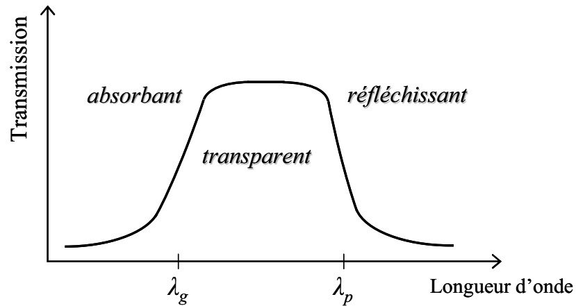
Figure 2. Dépendance spectrale typique d'un TCO 11 .
