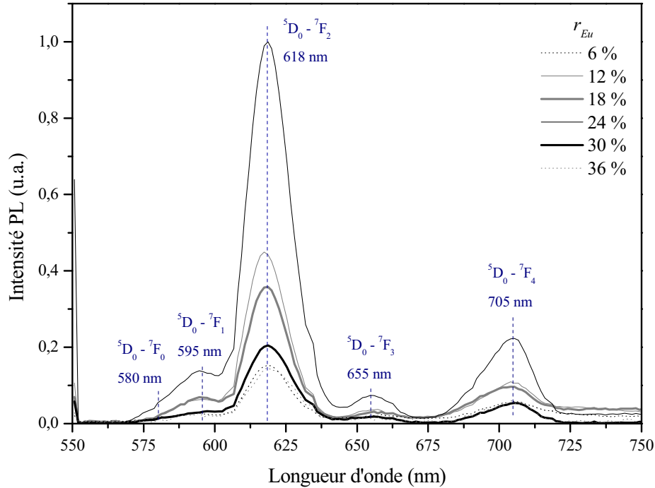
Figure 29. Spectres de photoluminescence de films d'oxyde de gallium dopés à l'europium déposés sur silicium. Différentes valeurs de r_{Eu} sont étudiées : 6% ; 12% ; 18% ; 24% ; 30% et 36%. Les films ont été fabriqués avec les paramètres de dépôt d=7 cm ; T_s=100^\circ\text{C} ; P_{Ar}=0,015 mbar ; P_{RF}=150 W.
