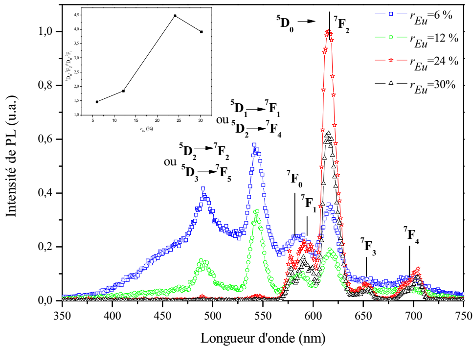
Figure 7. Spectres de photoluminescence de films d'oxyde de gallium dopés à l'euporium. Les films sont excités à une longueur d'onde de 275 nm. L'encart montre l'évolution du rapport d'intensité des transitions {}^5D_0 \rightarrow {}^7F_2 et {}^5D_0 \rightarrow {}^7F_1 en fonction du rapport r_{Eu} .
