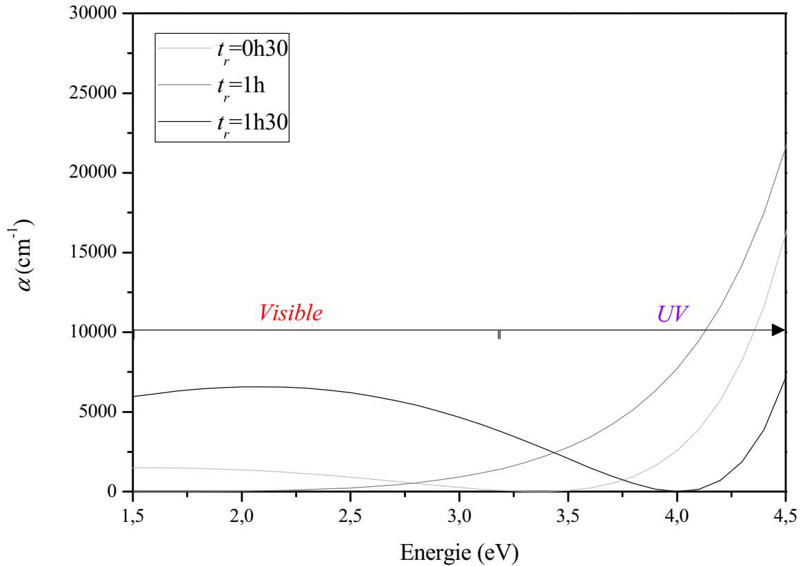
Figure 14. Evolution du coefficient d'absorption \alpha en fonction de l'énergie de trois films recuits à 1000°C pendant trois durées différentes : 0h30 ; 1h ; 1h30. Les trois films sont issus d'un même dépôt effectué avec les paramètres suivants : d=7 \text{ cm} ; T_s=100^\circ\text{C} ; t=1\text{h} ; P_{Ar}=0,017 \text{ mbar} ; P_{RF}=200 \text{ W} .
