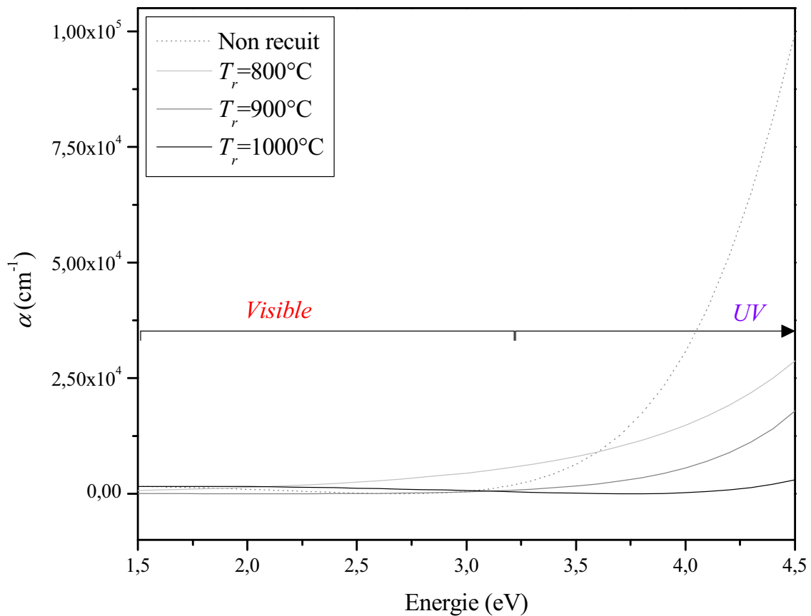
Figure 12. Evolution du coefficient d'absorption \alpha en fonction de l'énergie d'un film non recuit et de trois films recuits pendant 1h sous azote à des températures différentes: 800^\circ\text{C} ; 900^\circ\text{C} ; 1000^\circ\text{C} . Les quatre films sont issus d'un même dépôt effectué avec les paramètres suivants : d=7 \text{ cm} ; T_s=100^\circ\text{C} ; t=0\text{h}30 ; P_{Ar}=0,017 \text{ mbar} ; P_{RF}=200 \text{ W} .
