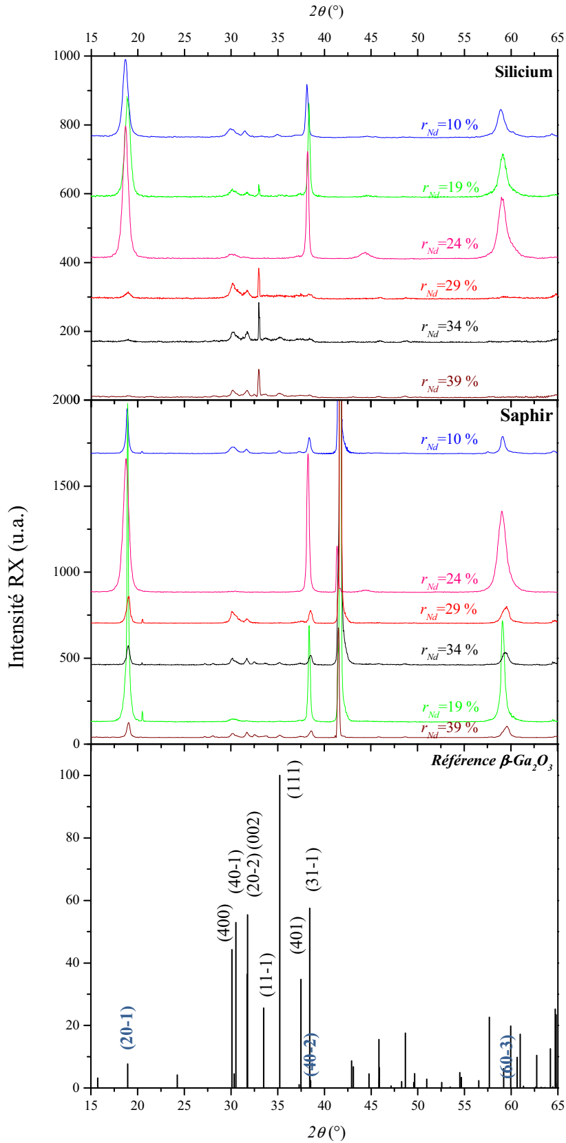
Figure 12. Diagrammes de diffraction des rayons X de films dopés au néodyme déposés sur substrats de silicium et de saphir avec r_{Nd}=10\% ; 19% ; 24% ; (d) 29% ; (e) 34% et (f) 39%.
