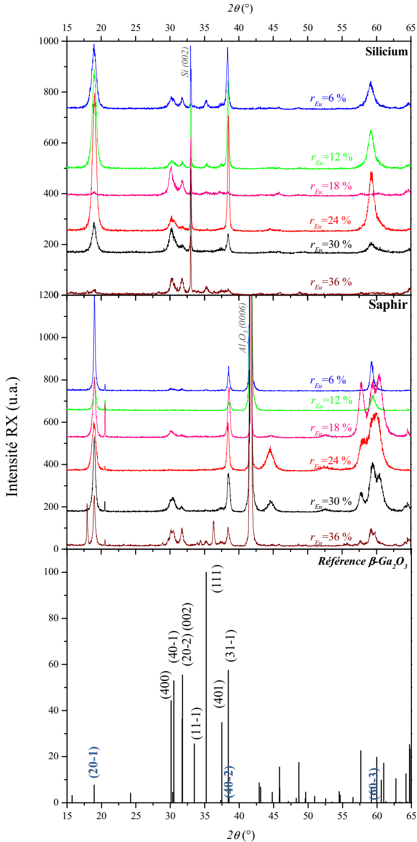
Figure 13. Diagrammes de diffraction des rayons X de films dopés à l'europium déposés sur substrats de silicium et de saphir avec r_{Eu}=6 ; 12% ; 18% ; 24% ; 30% et 36%.
