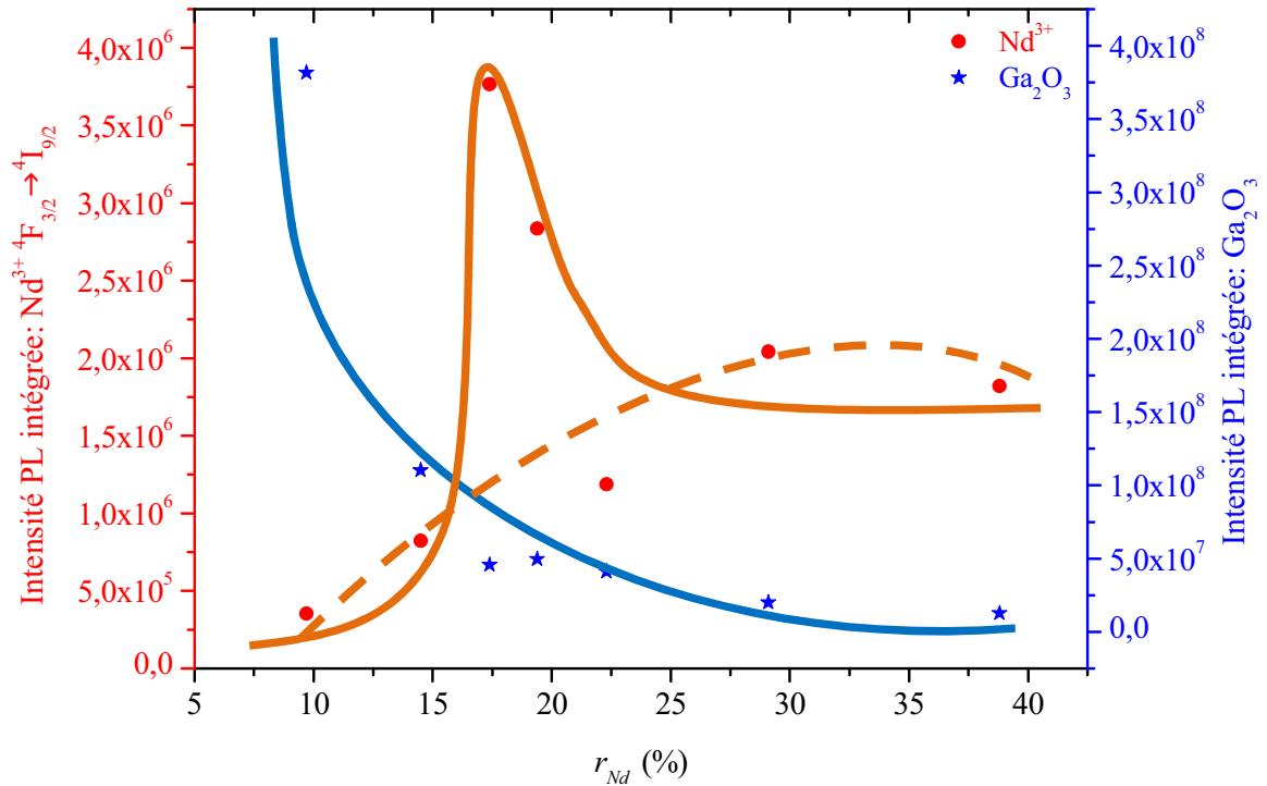
Figure 3. Evolution de l'intensité de PL intégrée des ions \text{Nd}^{3+} en fonction de r_{\text{Nd}} (transition 4F_{3/2} \rightarrow 4I_{9/2} ) et de la bande de défauts de \text{Ga}_2\text{O}_3 dans le visible. La longueur d'onde d'excitation est de 266 nm.
