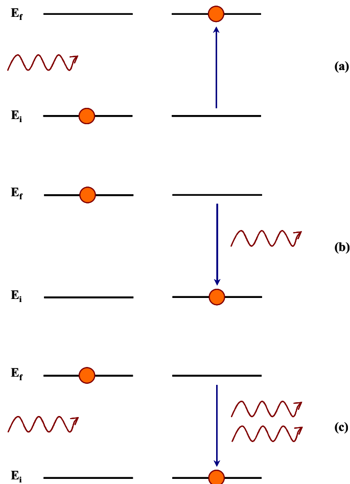
Figure 15. Représentation des trois processus (a) absorption, (b) émission spontanée, (c) émission stimulée pouvant se produire dans un matériau luminescent. La flèche ondulée correspond à un photon d'énergie E_f - E_i .
