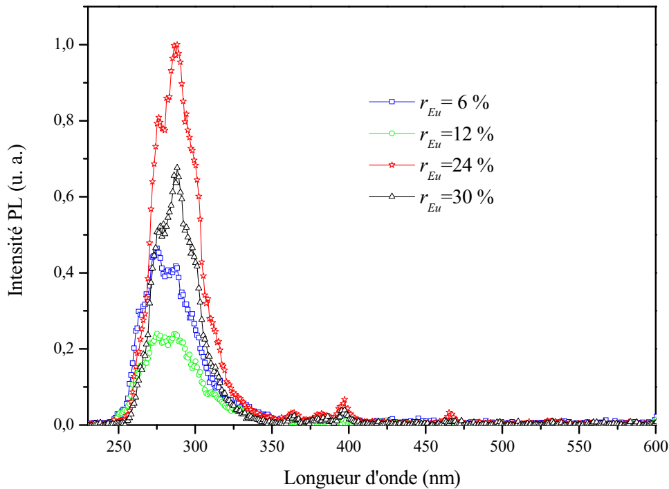
Figure 6. Spectres d'excitation de la photoluminescence des films d'oxyde de gallium dopés à l'eupruium et déposés sur des substrats de saphir. La longueur d'onde de détection de la PL est de 615 nm.
