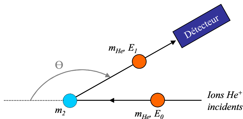
Figure 9. Principe de la technique RBS. Dans notre cas, l'angle \Theta est fixé à 165^\circ .
