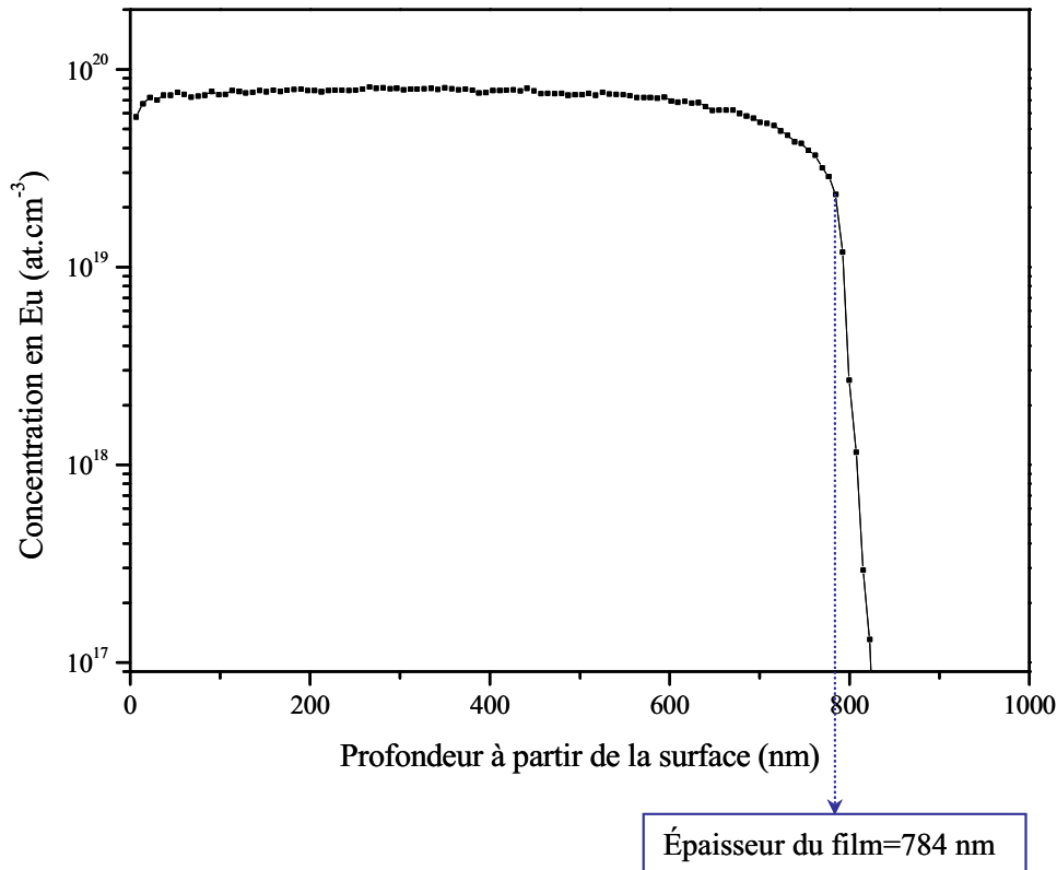
Figure 12. Profil de concentration d'un échantillon d'oxyde de gallium dopé à l'euphium. La concentration moyenne en europium dans la couche est de 7 \times 10^{19} atomes.cm -3 , et l'épaisseur de l'échantillon est évaluée à 784 nm.
