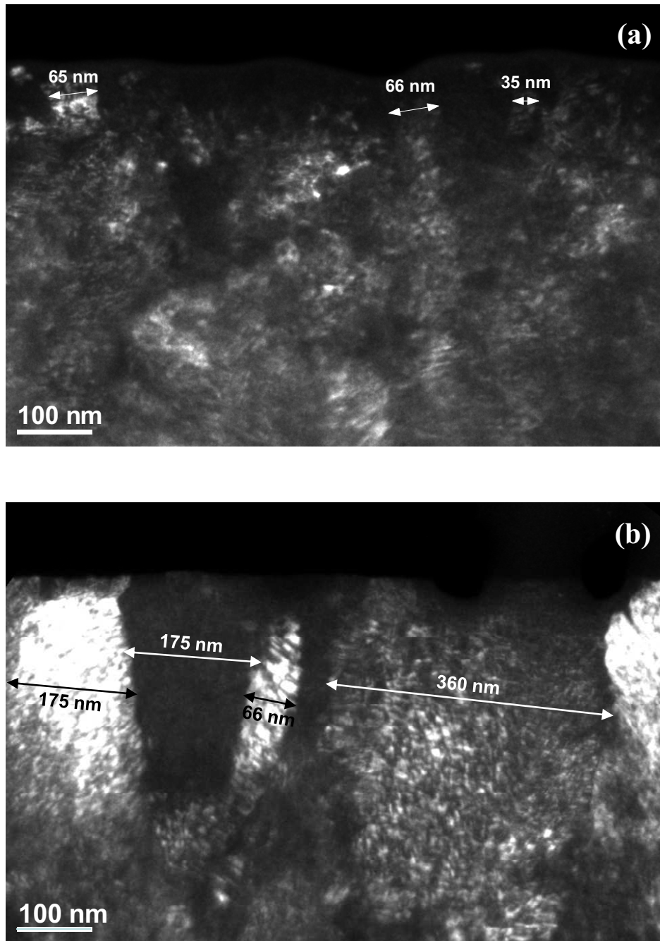
Figure 18. Image MET en champ noir d'un film d'oxyde de gallium dopé à l'europium avec r_{Eu}=30\% et déposé pendant le même processus sur un substrat (a) de silicium et (b) de saphir.
