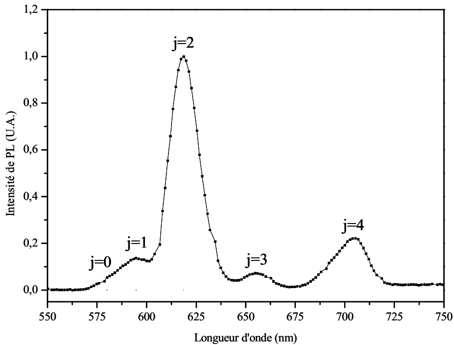
Figure 30. Spectre de PL d'un échantillon d'oxyde de gallium dopé à l'euporium ( r_{Eu} = 24\% ).
