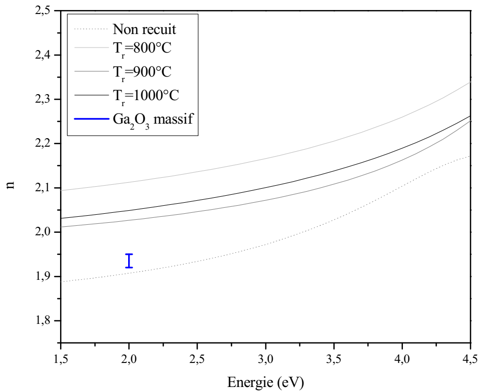
Figure 11. Courbes de dispersion de l'indice de réfraction n d'un film non recuit et de trois films recuits pendant 1h sous azote à des températures différentes: 800^\circ\text{C} ; 900^\circ\text{C} ; 1000^\circ\text{C} .
