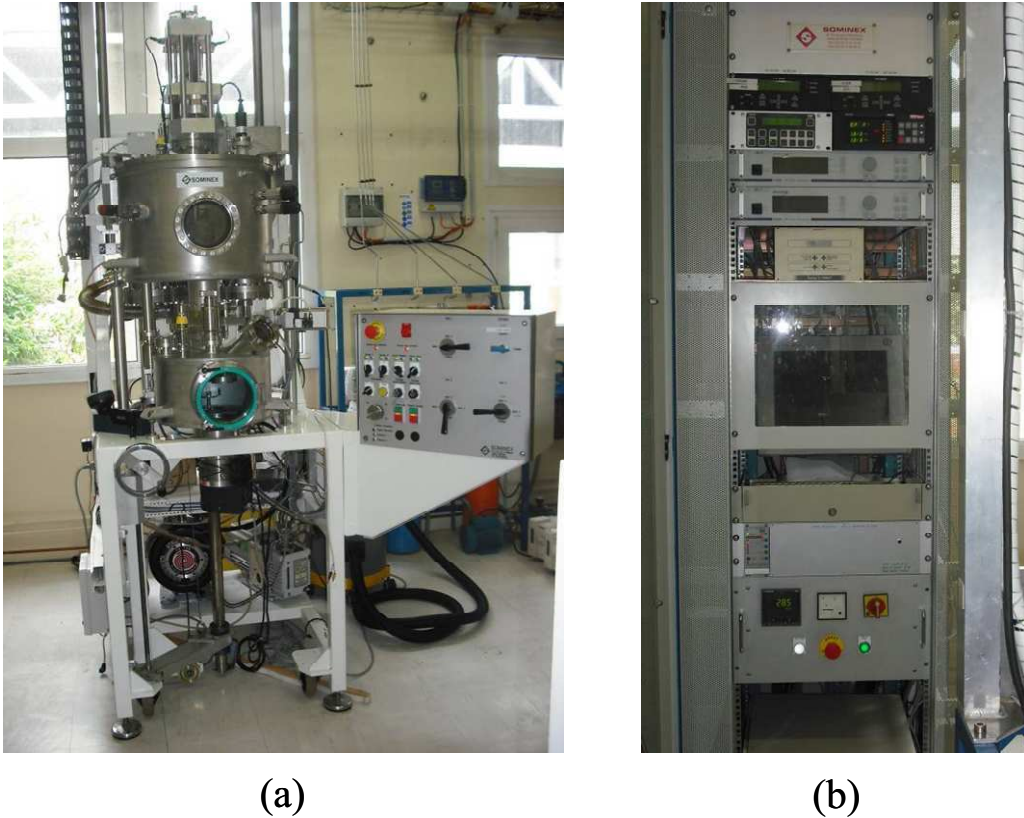
Figure 4. (a) Bâti de pulvérisation SOMINEX utilisé pour le dépôt des films minces ; (b) interface de contrôle des paramètres de dépôt.
