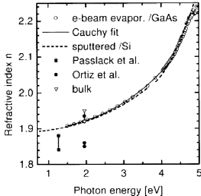
Figure 10. Indices de réfraction de films minces de \text{Ga}_2\text{O}_3 obtenus avec des méthodes de croissance différentes : spray pyrolyse (Ortiz et al. 64 ), évaporation par faisceau d'électrons (Passlack et al. 59 , Rebien et al. 60 ) et pulvérisation cathodique (Rebien et al. 60 ). L'indice de réfraction du cristal massif de \text{Ga}_2\text{O}_3 a été représenté pour une valeur d'énergie de 2 eV.
