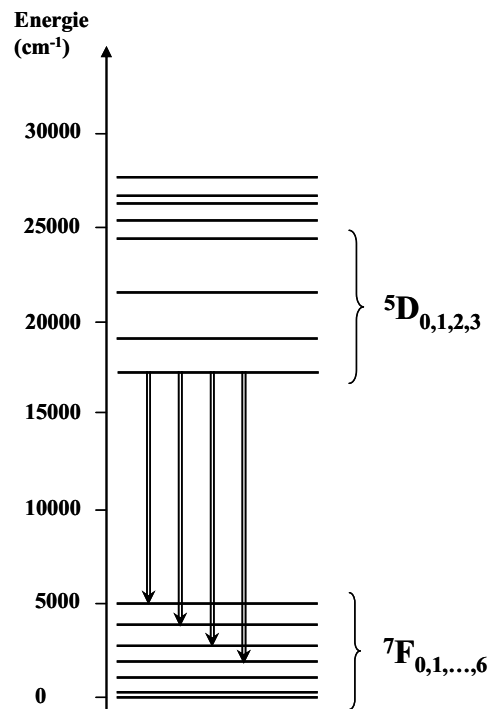
Figure 17. Diagramme partiel des niveaux d'énergie électronique de l'ion \text{Eu}^{3+97} .
