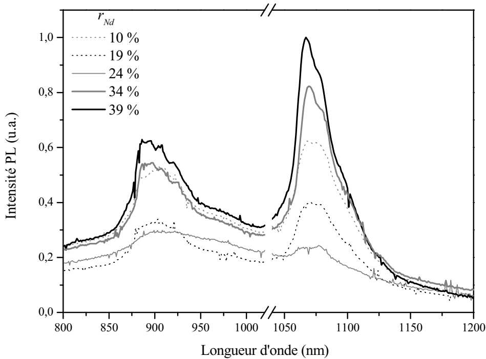
Figure 28. Spectres de photoluminescence de films d'oxyde de gallium dopés au néodyme déposés sur substrat de saphir. Différentes valeurs de r_{Nd} sont étudiées : 10% ; 19% ; 24% ; 34% et 39%. Les films ont été fabriqués avec les paramètres de dépôt d=7 cm ; T_s=100^\circ\text{C} ; P_{Ar}=0,015 mbar ; P_{RF}=150 W.
