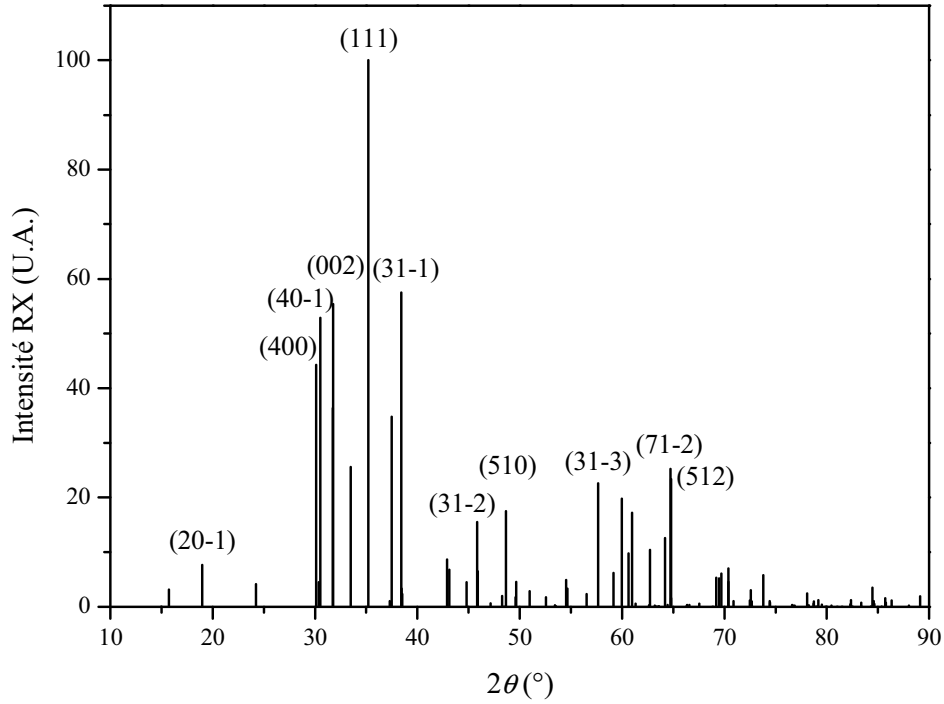
Figure 18. Diagramme théorique de diffraction des rayons X d'une poudre de Ga 2 O 3 monoclinique.
