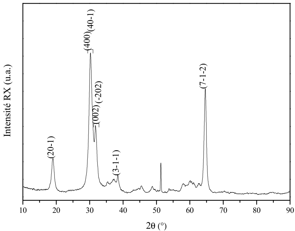
Figure 10. Diagramme RX d'un film mince déposé à T_s=600^\circ\text{C} et recuit à 1000^\circ\text{C} pendant 1h. Les paramètres du dépôt sont les suivants : d=7 cm ; t=0\text{h}30 ; P_{Ar}=0,017 mbar ; P_{RF}=200 W.
