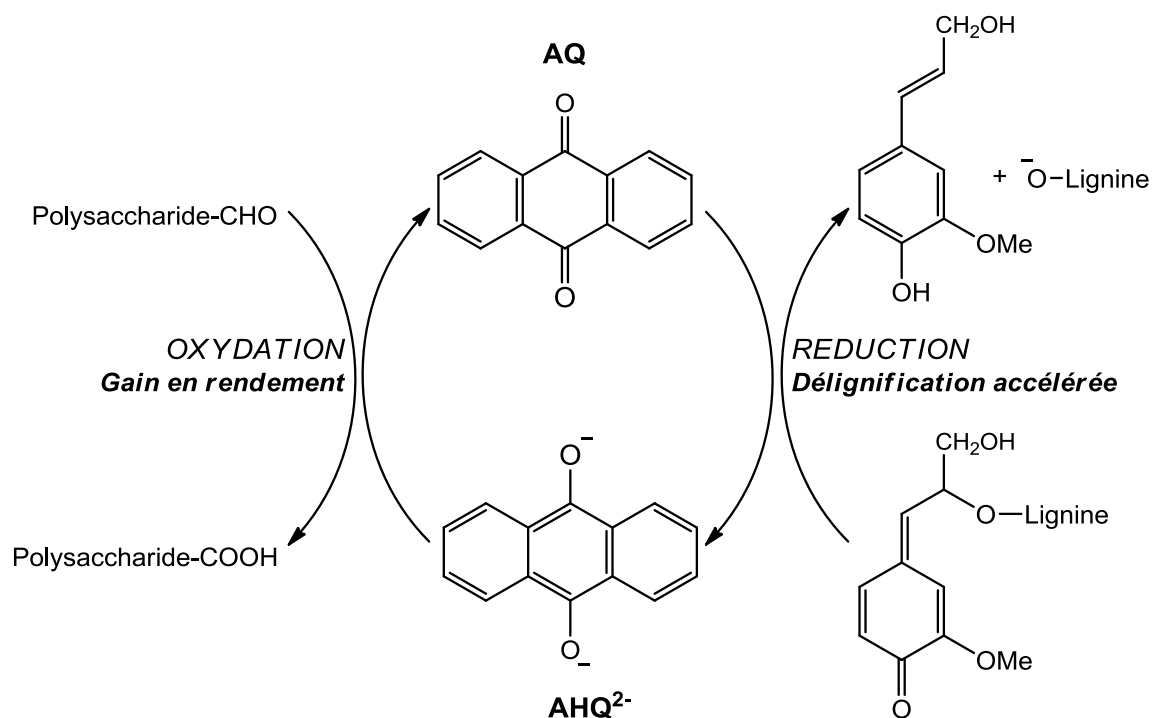
Figure I.25. Le cycle redox de l'action catalytique de l'antraquinone
