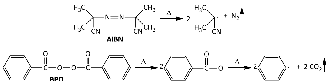
Figure II.4. Décomposition thermique des amorceurs
