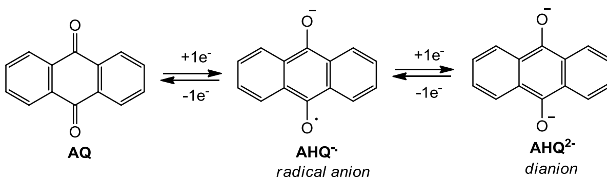
Figure I.24. Les différents états d'oxydation de l'antraquinone
