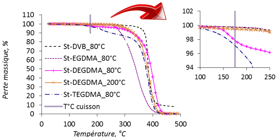
Figure II.30. Stabilité thermique des monolithes N° 7, 8, 9, 10 avant cuisson
