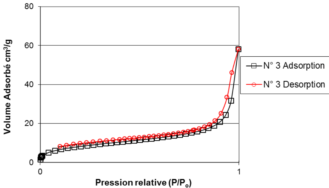
Figure II.9. Isotherme d'adsorption-désorption d'azote du monolithe N° 3
