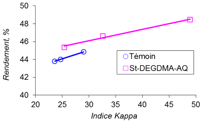
Figure III.14. Rendement en pâte obtenu en fonction de l'indice kappa final pour des cuissons visant des indices kappa faibles en présence ou non des monolithes anthraquinoniques
