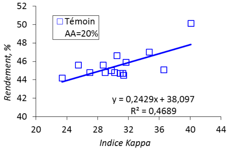
Figure III.22. Dispersion des témoins pour un alcali actif (AA) constant de 20%
