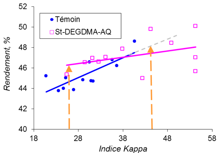
Figure III.18. Rendement en pâte obtenu en fonction de l'indice kappa final pour des cuissons visant des indices kappa faibles en présence ou non des monolithes St-DEGDMA-AQ
