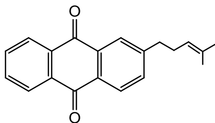
Figure III.10. Structure de l'AQMB, dérivé de l'antraquinone
