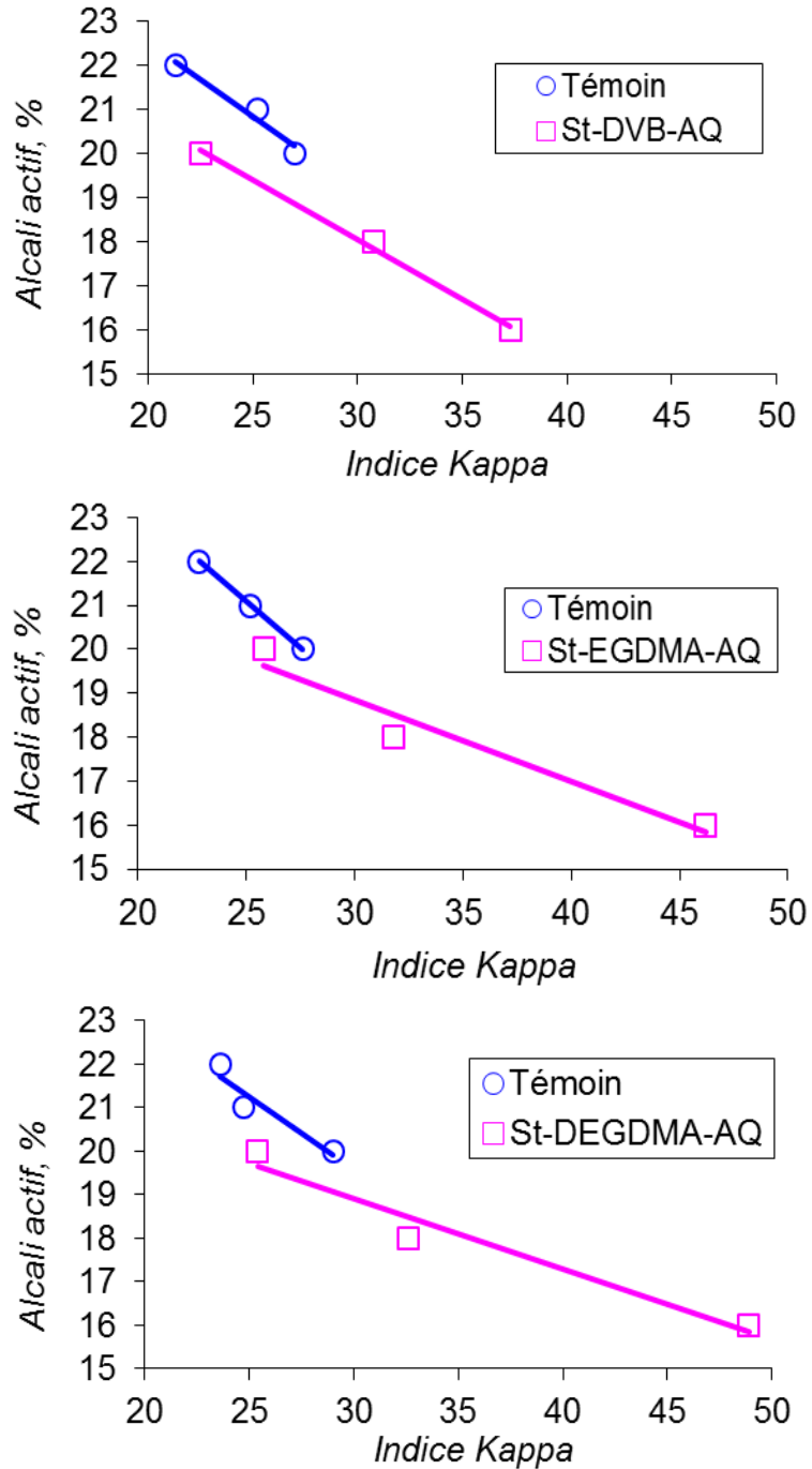
Figure III.13. Alcali actif utilisé en fonction de l'indice kappa final pour des cuissons visant des indices kappa faibles en présence ou non des monolithes antraquinoniques
