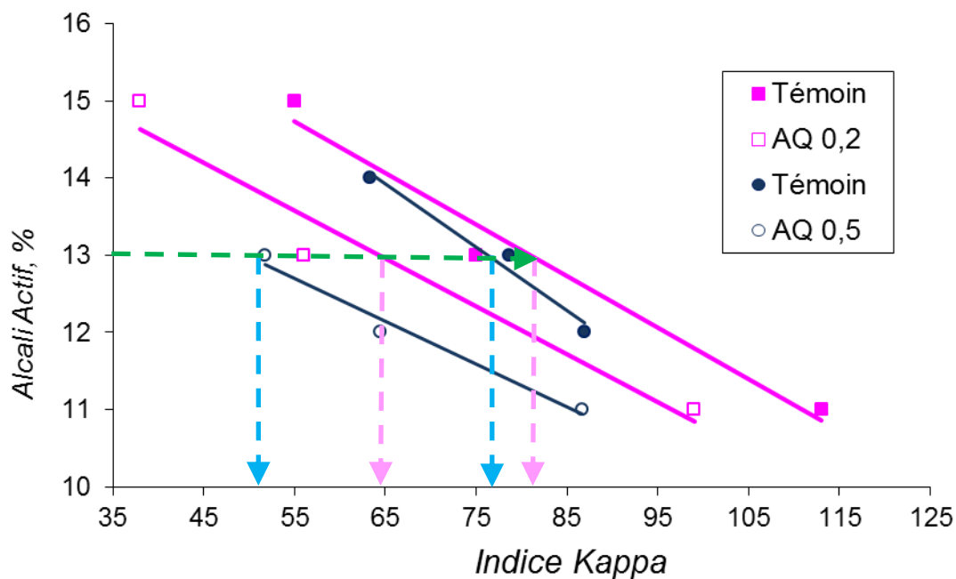
Figure III.6. Alcali actif utilisé en fonction de l'indice kappa final pour des cuissons visant des indices kappa élevés en présence ou non d'antraquinone (poudre)
