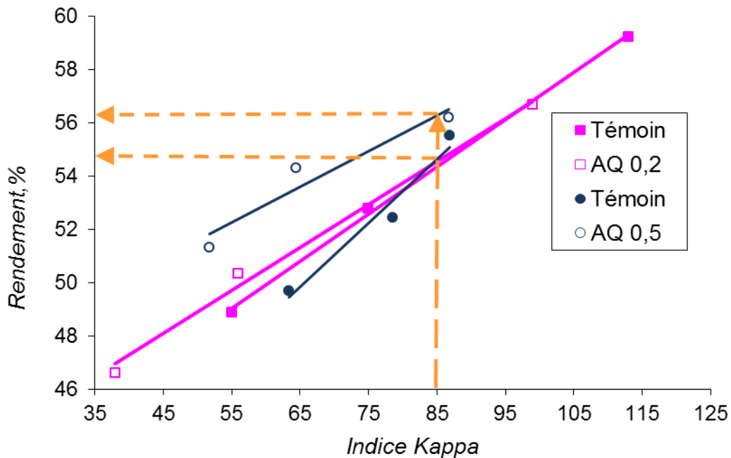
Figure III.7. Rendement en pâte obtenu en fonction de l'indice kappa final pour des cuissons visant des indices kappa élevés en présence ou non d'antraquinone (poudre)
