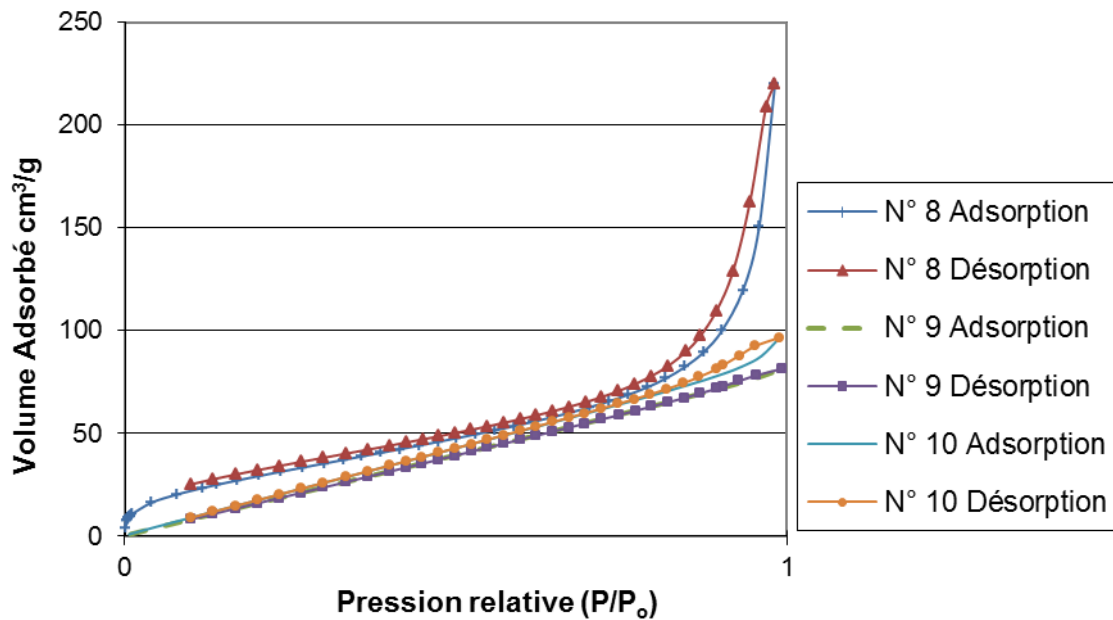
Figure II.19. Isothermes d'adsorption-désorption d'azote des monolithes N° 8, 9 et 10
