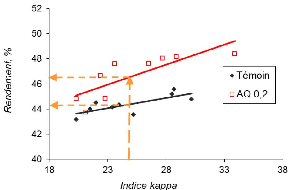
Figure III.9. Rendement en pâte obtenu en fonction de l'indice kappa final pour des cuissons visant des indices kappa faibles en présence ou non d'antraquinone (poudre)
