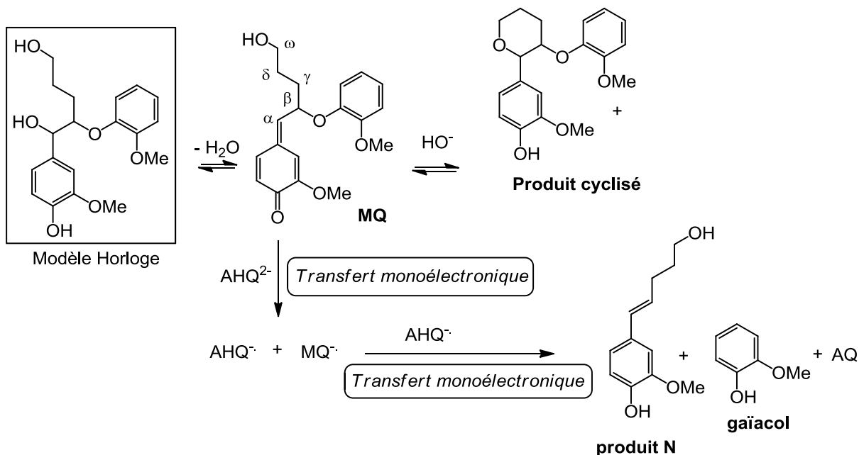
Figure I.27. Mécanisme de l'action catalytique de l'antraquinone sur le modèle « horloge »
