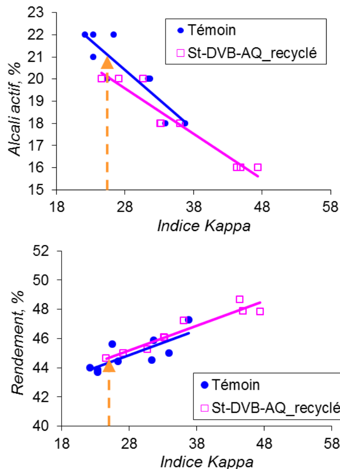
Figure III.20. Influence sur l'alcali actif et le rendement des monolithes St-DVB-AQ recyclés
