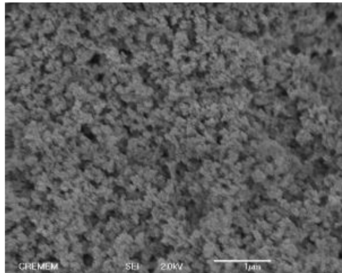
Figure II.26. Morphologie des monolithes St-EGDMA (N° 12) de diamètre 6 mm (x20000)
