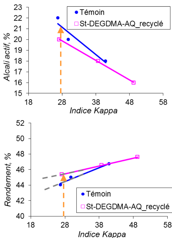
Figure III.21. Influence sur l'alcali actif et le rendement des monolithes St-DEGDMA-AQ recyclés
