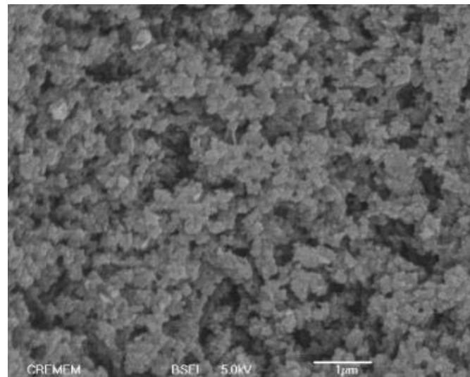
Figure II.39. Morphologie des monolithes St-EGDMA-AQ (N° 15) (x20000)
