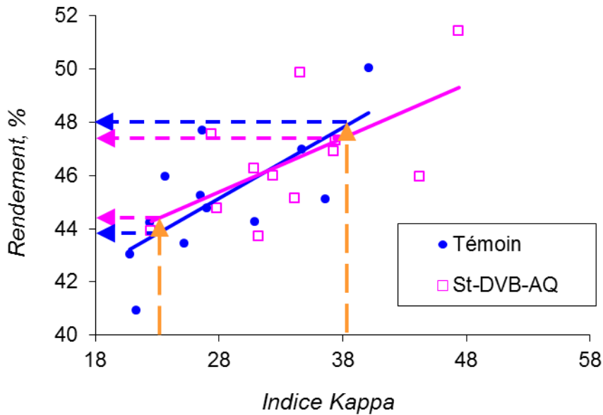
Figure III.17. Rendement en pâte obtenu en fonction de l'indice kappa final pour des cuissons visant des indices kappa faibles en présence ou non des monolithes St-DVB-AQ
