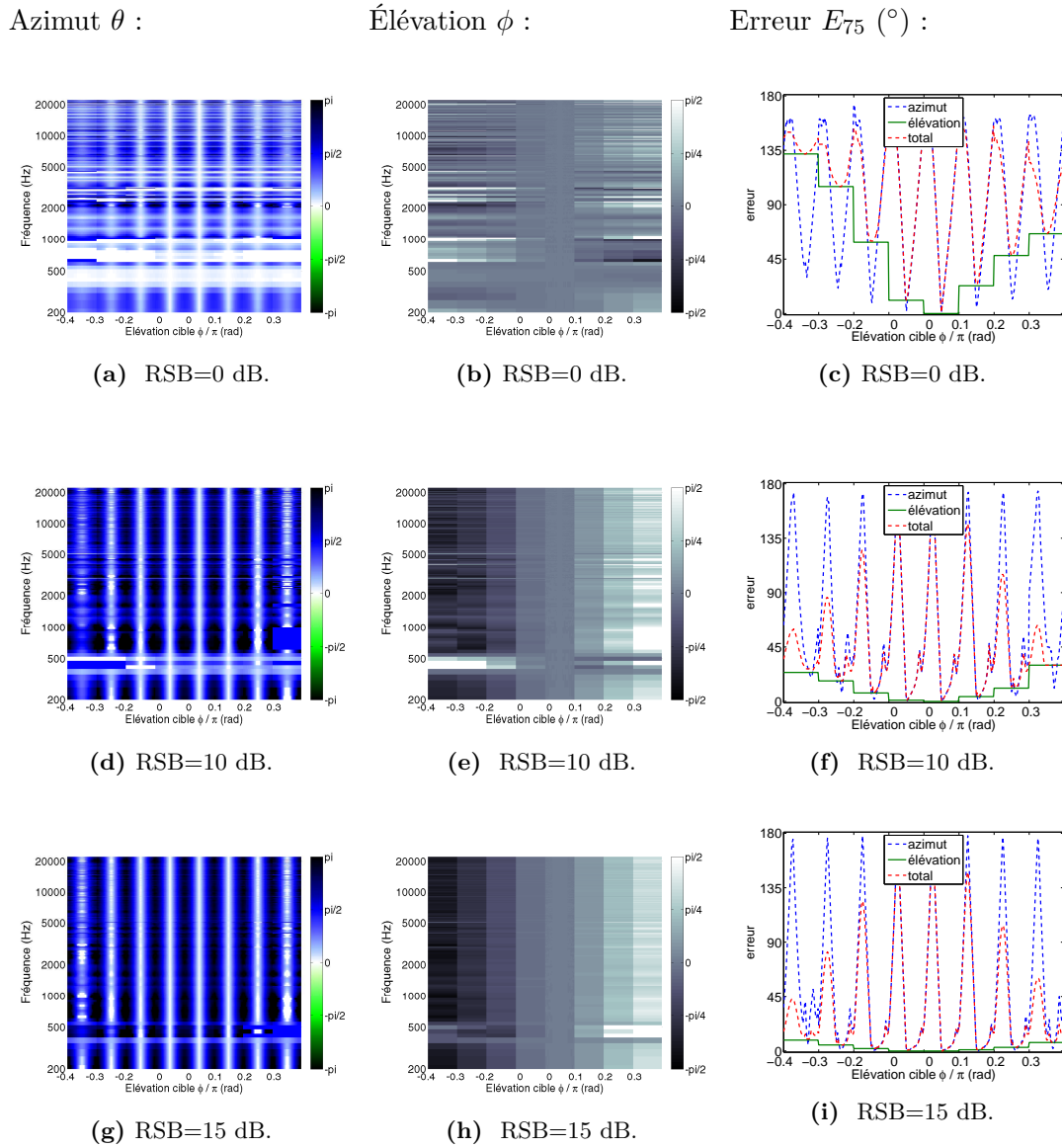
Figure IV.28 : Localisation d'une source large bande suivant la trajectoire illustrée dans la figure IV.14 en présence d'une source de bruit à (0,0) avec des RSB différents (ligne 1 0 dB, ligne 2 10 dB, ligne 3 15 dB). Localisation effectuée à partir du format B de l'ambisonique à l'ordre 1. L'estimation de l'azimut en colonne 1 et de l'élévation en colonne 2 sont affichées dans une représentation conjointe position-fréquence. Les erreurs E_{75} associées sont représentées dans la troisième colonne.
