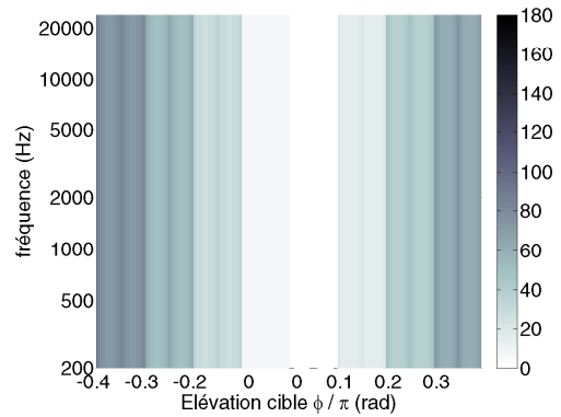
(d) Représentation conjointe position-fréquence de l'erreur de localisation E_t ( ^{\circ} ).
