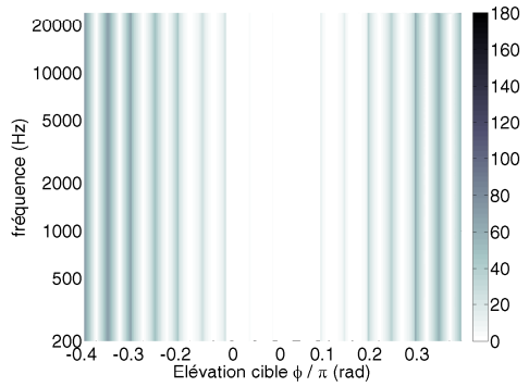
(c) Erreur de localisation sur l'azimut E_{\theta} dans une représentation conjointe position-fréquence.
