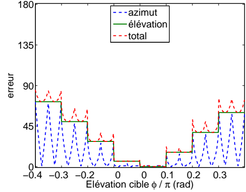
(b) Erreur E_{75} ( ^{\circ} ).
