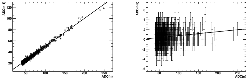
FIGURE 3.20 – Détermination des pentes \frac{n-1}{n} et \frac{n-2}{n} pour une tour de déclenchement typique. Pour le second rapport, un grand nombre de pulses est nécessaire aux basses énergies pour que les valeurs ADC (entières) se moyennent.
