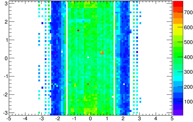
FIGURE 3.29 – Intervalle de recouvrement ( \text{GeV } E_T ) des domaines de validité de l’algorithme à détection de pic et de celui à seuils, tel que calculé pour le run 165632.
