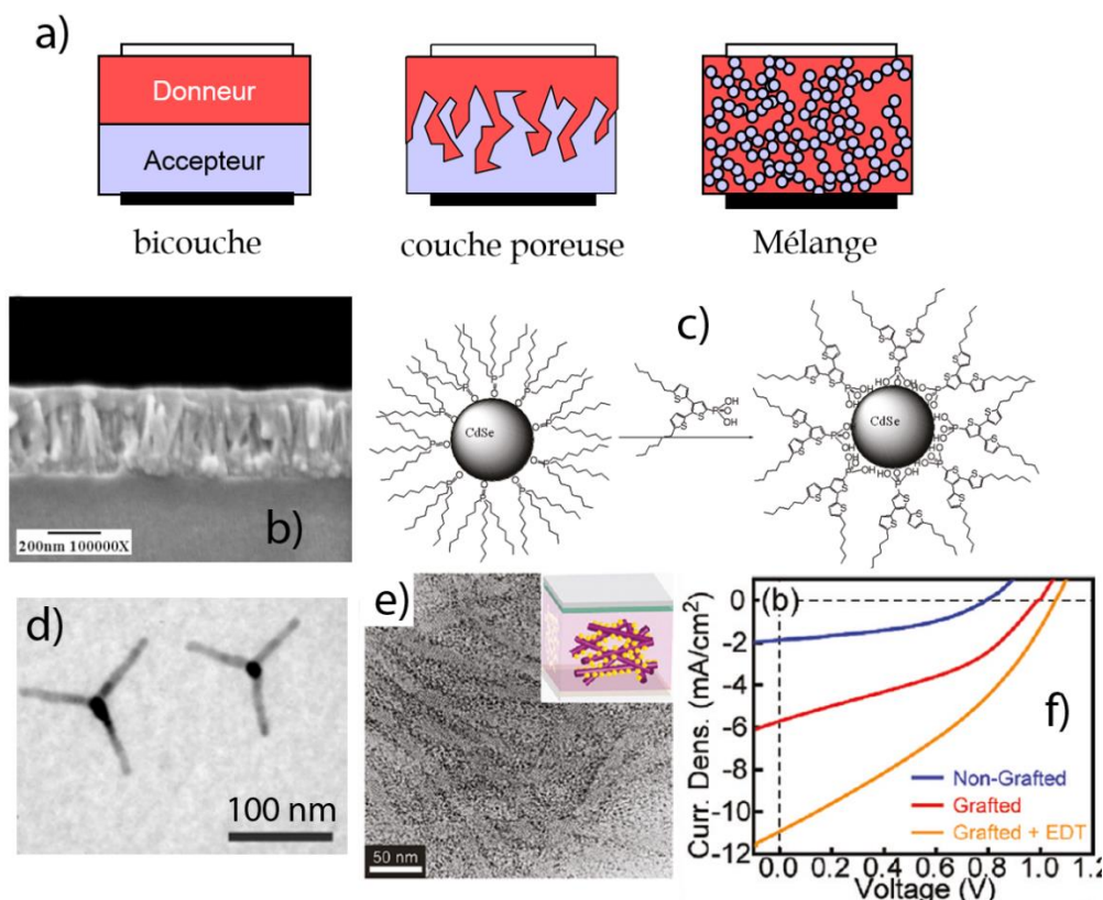
Figure 18 – a) Structures schématiques des approches hybrides à hétérojonctions. b) Image de microscopie électronique d'une électrode à base de nanofibres de ZnO infiltrée par du P3HT (D. C. Olson et al., J. Phys. Chem. C 111 (2007) 16670). c) Exemple de procédure d'échange de ligands appliquée à des nanocristaux de CdSe (Y. Park et al., Chem. Mater. 23 (2011) 4273). d) Tétrapodes de CdSe utilisés dans des mélanges polymère/nanocristaux de près de 3% de rendement (B. Sun et al., J. Appl. Phys. 97 (2005) 014914). e) Morphologie d'un composite fibriles de P3HT/CdS et f) caractéristiques courant-tension correspondant au rendement de conversion record (4.1%) pour un mélange polymère/nanocristaux (S. Ren et al., Nano Letters 11 (2011) 3998).
