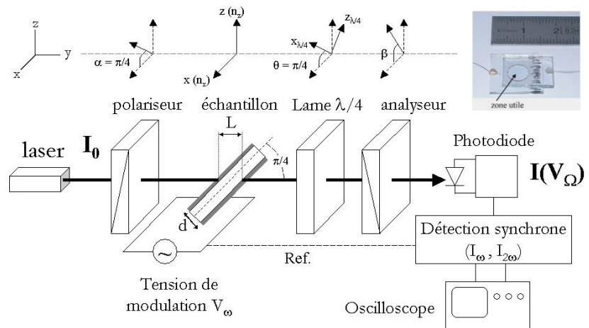
Figure 12 – Montage de Sénarmont en régime dynamique pour la mesure des propriétés électro-optiques des composites polymère/SiC
