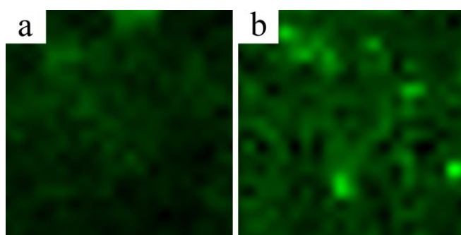
Figure 47 – Cartographies Raman des nanopoudres composites \text{TiO}_2/\text{NTC} (a) ex situ (concentration en NTC de 0.1% en masse) et (b) in situ (concentration en NTC de 0.03% en masse) sur une surface de 40 \times 40 \mu\text{m} . Le contraste est associé à l'amplitude de la bande de désordre (bande D) associée aux nanotubes. A droite sont présentés les paramètres photovoltaïques déduits sous illumination standard des cellules ssDSSCs réalisées à partir d'électrodes poreuses composites.
