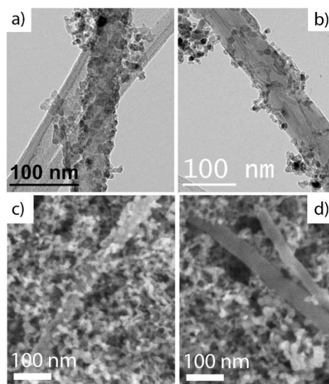
Figure 46 – Images MET de composites \text{TiO}_2/\text{NTC} (a) in situ et (b) ex situ . En (c) et (d) : images par MEB des mêmes composites mis sous la forme d'électrodes poreuses.
