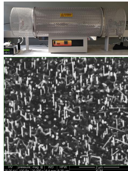
Figure 79 – Four tubulaire utilisé à XLIM pour la synthèse par VLS de nanofils de ZnO et premiers nanofils synthétisés au laboratoire en 2014.
