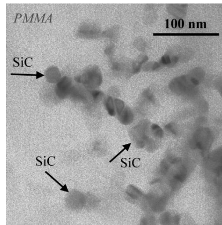
Figure 11 - Image MET d'un composite polymère (PMMA):SiC (1% en masse)
