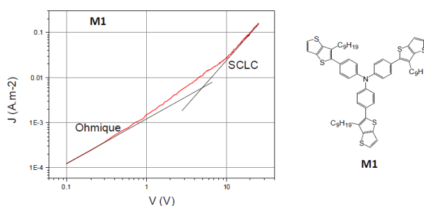
Figure 42 – Caractéristique J(V) d'un composant « à trous » élaboré à partir du verre moléculaire M1 (LPPI, Cergy-Pontoise) permettant d'estimer une mobilité de charge de 1,5 \cdot 10^{-5} \text{ cm}^2 \cdot \text{V}^{-1} \cdot \text{s}^{-1}
