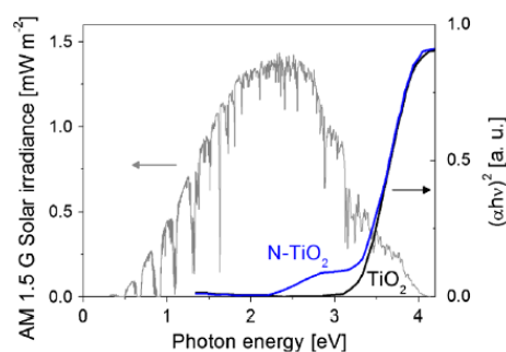
Figure 32 – Comparaison des propriétés optiques de nanopoudres de TiO 2 et N-TiO 2 par rapport au spectre solaire standard.
