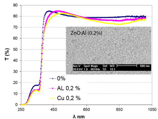
Figure 26 – Transmission optique de couches minces de \text{ZnO} dopées réalisées par pyrolyse en spray et image MEB correspondante ( \text{ZnO:Al} )
