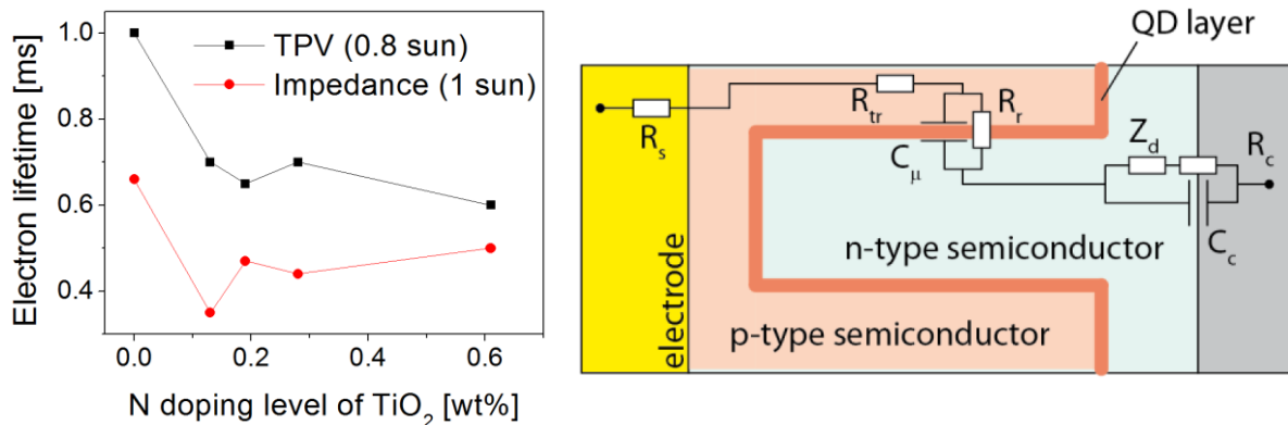
Figure 69 – A gauche : Durée de vie des électrons mesurée par décroissance de photo-tensions (TPV) et par spectroscopie d'impédance sur des cellules ssDSSC à base d'électrodes poreuses de TiO 2 pour différents taux de dopage à l'azote. A droite : Circuit électrique équivalent potentiel associé à une cellule QSSC.
