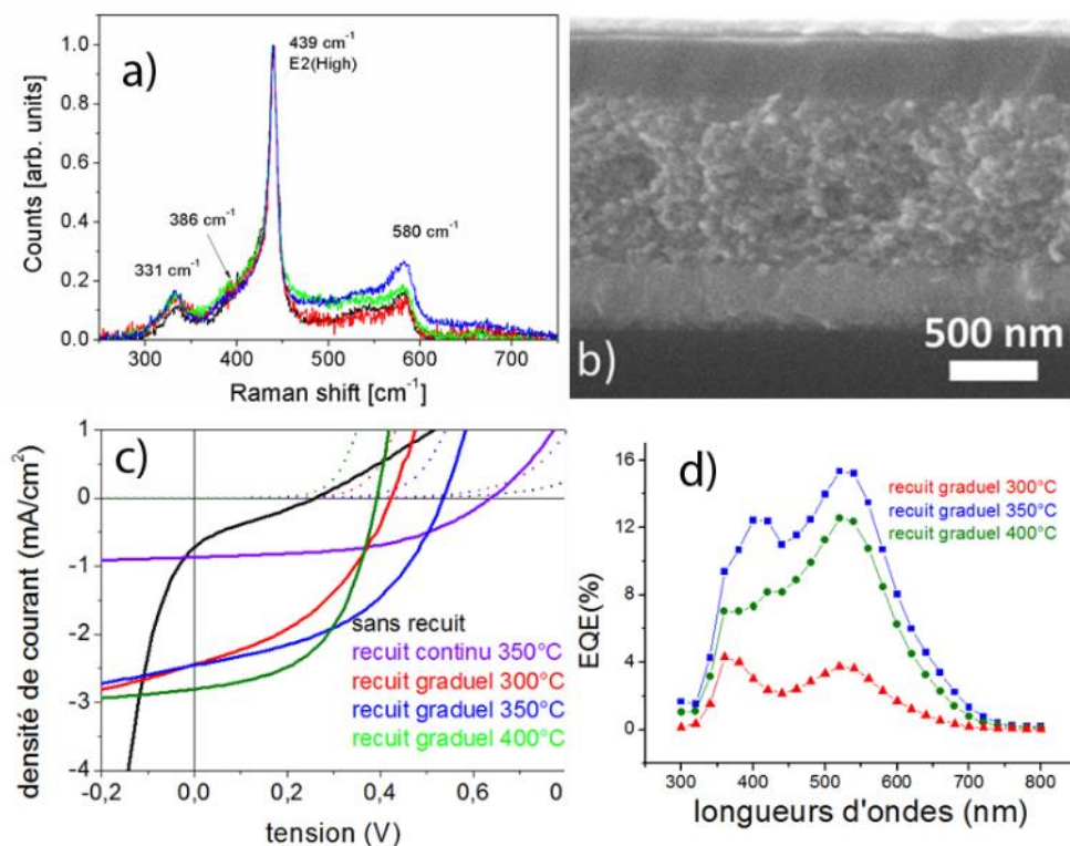
Figure 28 – a) Spectres de diffusion Raman de couches poreuses de ZnO élaborées en solution. b) Coupe transverse d'une cellule ssDSC ZnO. c) caractéristiques électriques des cellules ssDSC en fonction des paramètres de recuit des couches. d) Spectres IPCE correspondants.
