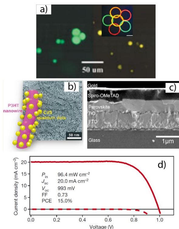
Figure 7 - a) et b) : exemples de composites hybrides luminescents CdTe/polymère fonctionnel AFPC (microspheres et anneaux, issu de H. Zhang et al., Adv. Mater. 17 (2005) 853). b) Composite nanofils de P3HT/nanocristaux de CdS pour la conversion photovoltaïque (S. Ren et al., Nano Letters 11 (2011) 3998). c) Structure d'une cellule hybride pérovskite et d) caractéristique courant-tension sous illumination standard (Burschka et al., Nature 499 (2013) 316).
