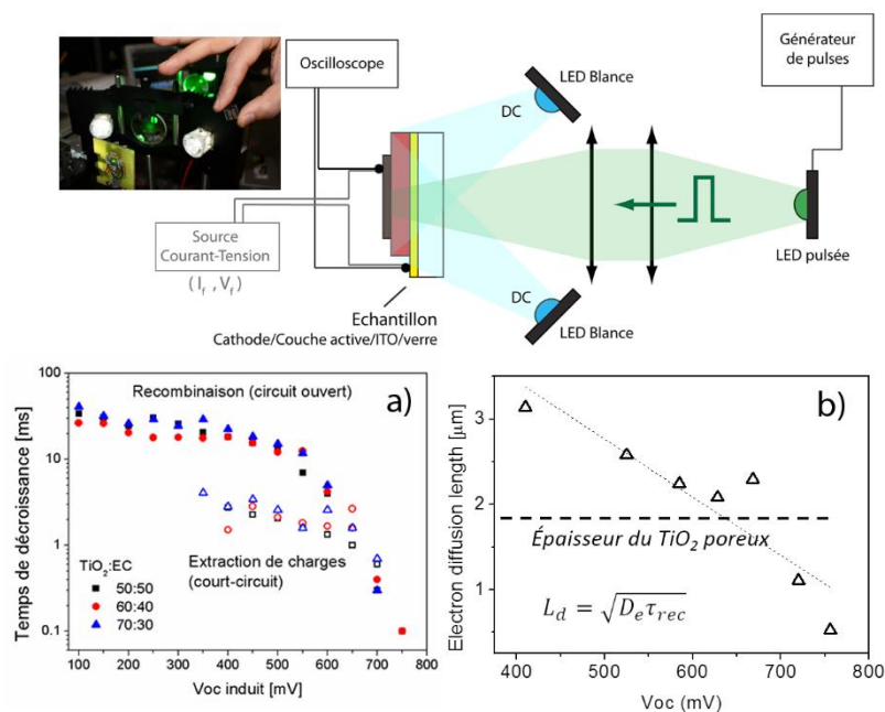
Figure 60 – Montage expérimental pour les mesures TPV-TPC. a) Exemple de caractérisations menées à Limoges sur des cellules ssDSSC solides à base de \text{TiO}_2 et pour différentes formulations de colles de \text{TiO}_2 (rapport \text{TiO}_2 :ethylcellulose (EC)). b) Longueurs de diffusion des électrons déduite de la mesure.
