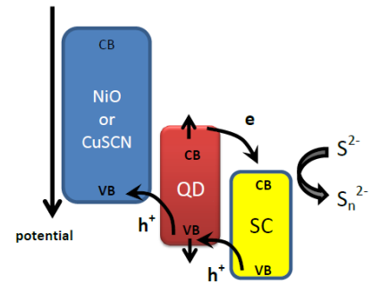
Figure 66 – Schéma illustrant les mouvements électroniques d'un système à base de QD sur NiO ou CuSCN, en présence d'un revêtement semi-conducteur et d'un électrolyte liquide (schéma projet QUEPHELEC).
