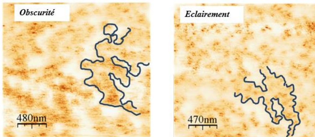
Figure 53 – Cartographies de photo-courants obtenues dans le noir et sous éclairage solaire simulé sur une couche active P3HT:PCBM présentant un rapport massique de 1:1.2 (tension de polarisation de -2V).
