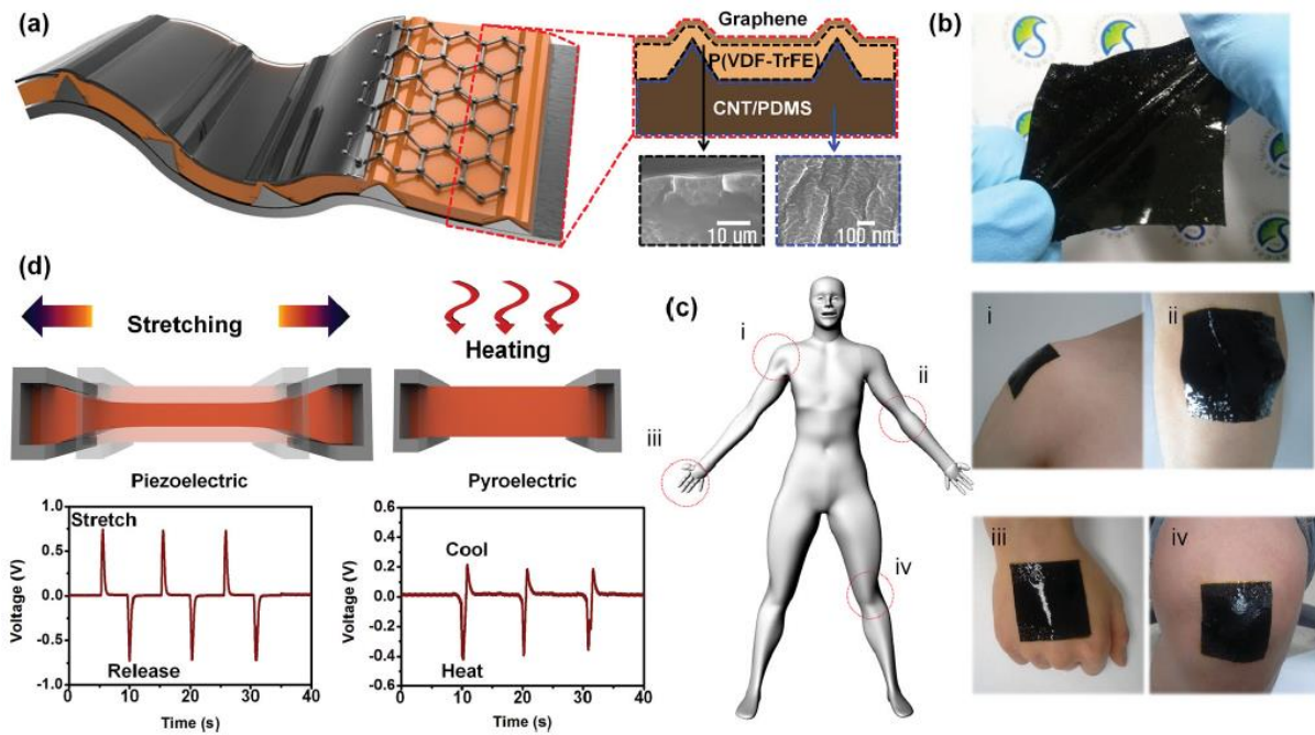
Figure 77 – Nano-générateur hybride piézoélectrique / pyroélectrique à base de P(VDF-TrFE) et d'électrodes de graphène et de composite PDMS/NTC. Le système est étirable et permet de récupérer l'énergie thermique et mécanique environnante (J.-H. Lee et al., Adv. Mater. 26 (2014) 765).
