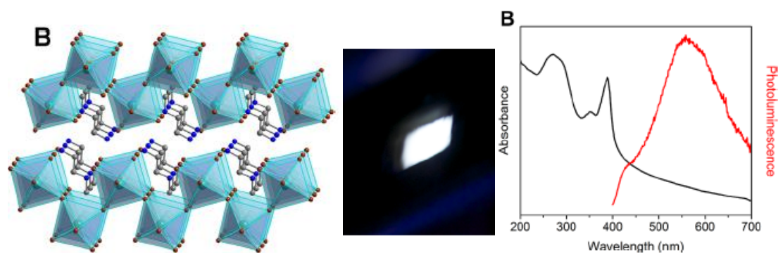
Figure 86 – A gauche : structure de la pérovskite 2D (N-MEDA)^6[PbBr_4] présentant une photoluminescence dans le blanc (photographie centrale). A droite : spectres optiques d'absorption et d'émission (excitation à 380nm) du matériau. Issu de E. R. Dohner et al., J. Am. Chem. Soc. 136 (2014) 1718).
