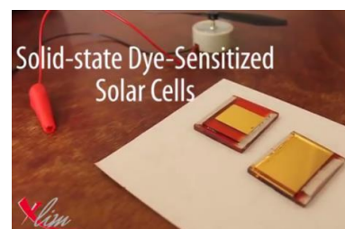
Figure 31 – Démonstrateurs XLIM ssDSSC (surface active 4 cm 2 )
