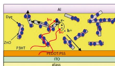
Figure 23 – Système hybride à base d'un mélange P3HT/nano-bâtonnets de \text{ZnO} greffés par des ligands porphyrines TCPP (A. Said et al., J. Phys. Chem. C 114 (2010) 11273).
