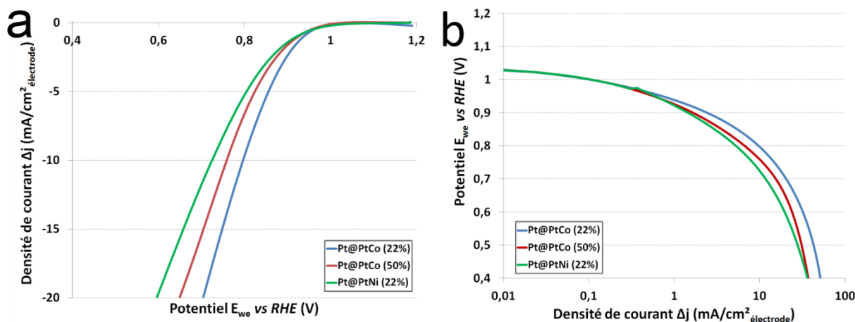
Figure 95 : Voltampérogrammes sous O_2 des particules Pt@PtM (5 mV/s; H_2SO_4 0,5M; N_2 : environ 200\mu g_P/cm^2_{\text{électrode}} )
