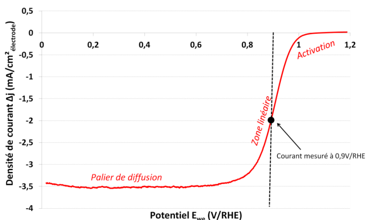
Figure 61 : Voltampérométries sous O_2 à 900 rpm du catalyseur PtCo/C corrigé de l'effet capacitif et des réactions parasites. (1 mV/s, H_2SO_4 0,5 M)
