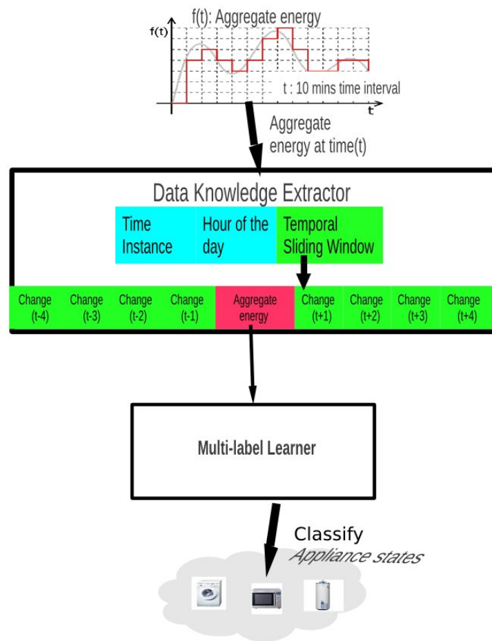
FIGURE 11.13 – Synoptique d'identification des charges
