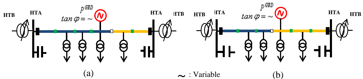
Figure I.9 : (a) Coordination optimale des moyens de réglage (configuration, GED, gradins, transformateurs) et (b) reconfiguration optimale avec GED
