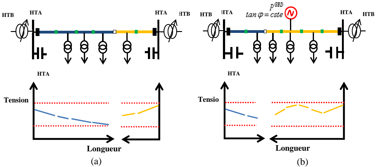
Figure I.8 : Reconfiguration sans et avec GED
