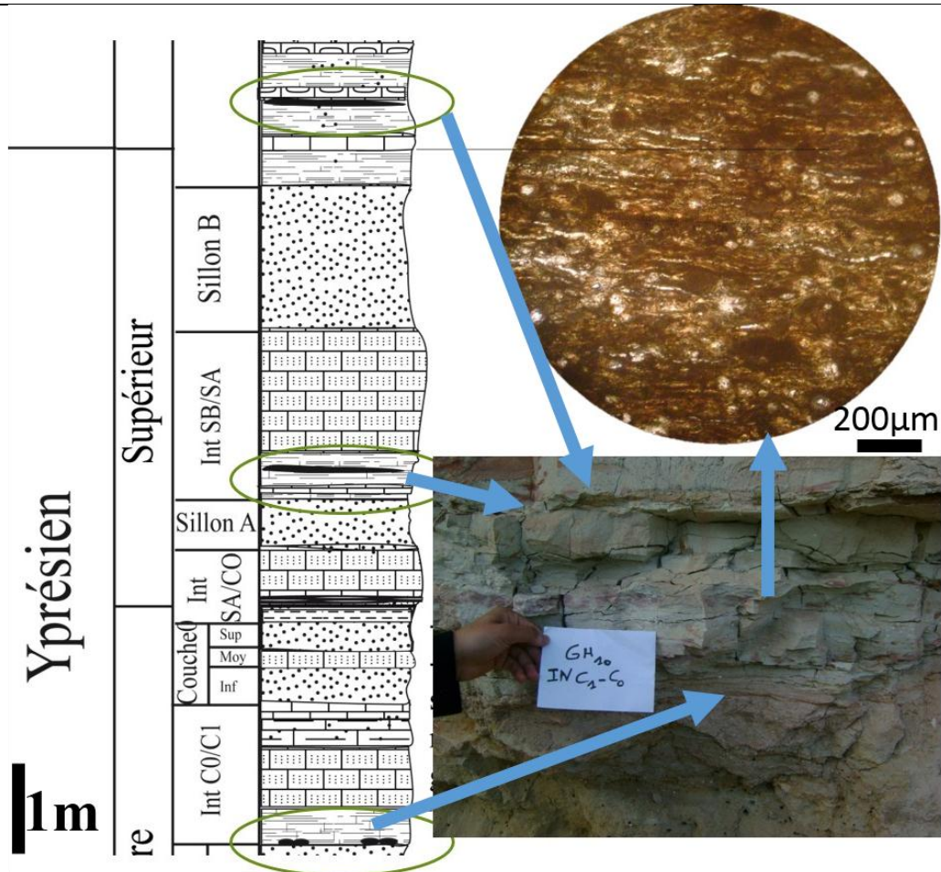
Figure 27: Microfaciès marneux siliceux et silicifiés du gisement de Ghar Tajer du bassin des Ouled Abdoun (EL Haddi et al. , 2014a)
