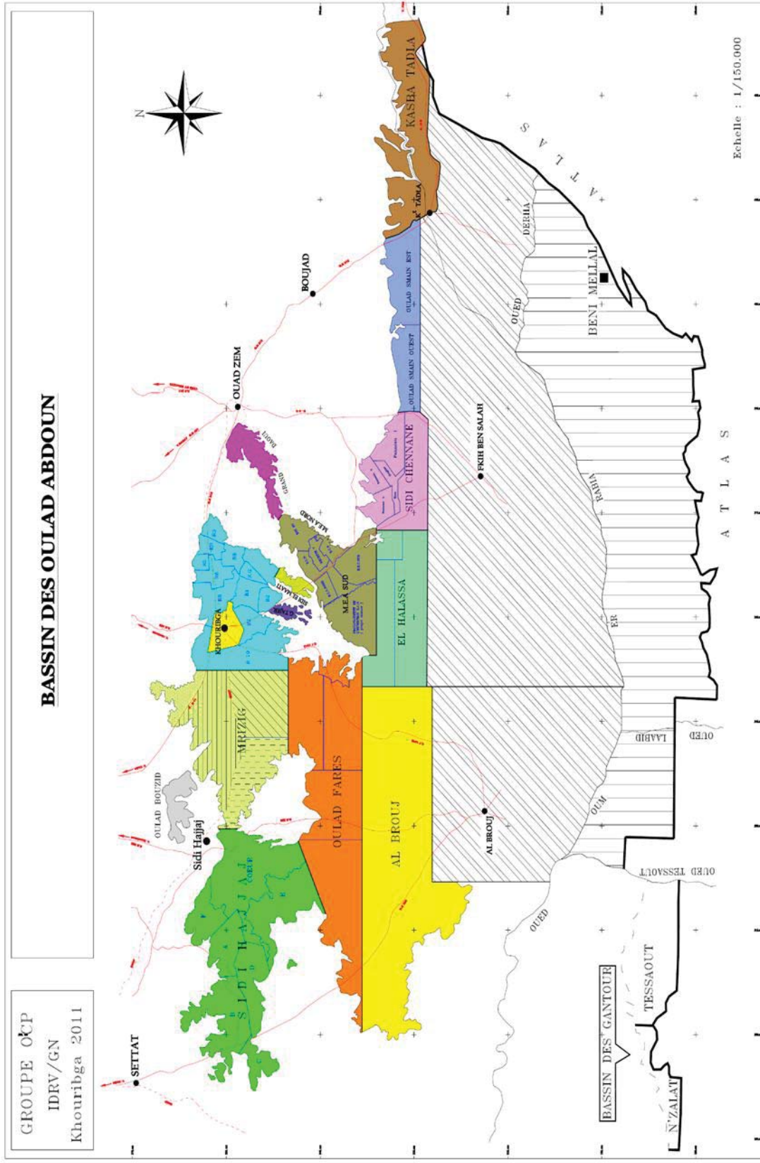
Figure 15: Localisation géographique des gisements du bassin des Ouled Abdoun d'après IDR V/GN (2011)
