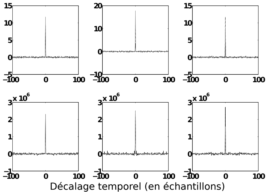
FIGURE II.9 – Autocorrélation des signaux blanchis \tilde{c}A^n (ligne supérieure) and \tilde{c}D_T^n (ligne inférieure) pour des filtres blanchisseurs à 1 pôle-1 zéro. Les paramètres et couleurs utilisés sont les mêmes que figure II.5.
