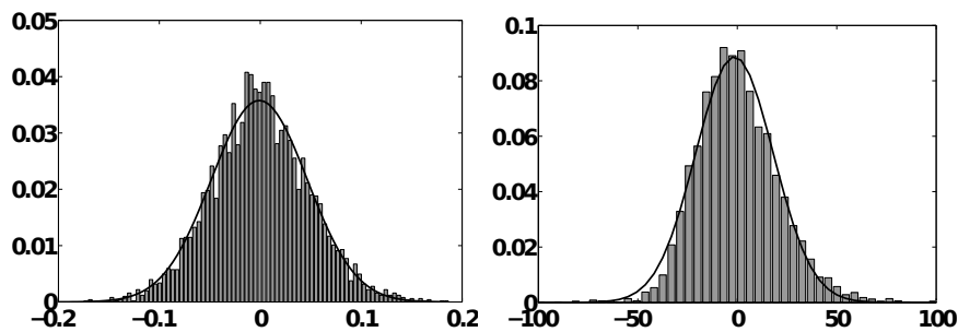
FIGURE II.10 – Barres : densité de probabilité estimée de \tilde{c}A (gauche) et \tilde{c}D_T (droite). Courbe noire : estimation par les moindres carrés des lois gaussiennes. Pour rester lisible, seules les estimations avec les paramètres \kappa=5 \cdot 10^9 \text{ N.m}^{-\alpha} \cdot \text{kg}^{-1} , \mu=1 \text{ s.m}^{-1} and \beta=-0.5 sont représentées. Les estimations pour les autres jeux de paramètres sont disponibles en annexe A.
