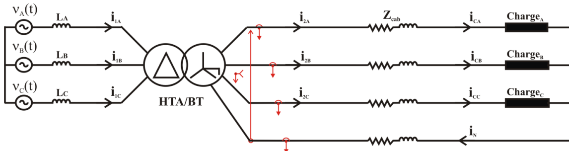
Fig. 2-14. Schéma équivalent simplifié d'un réseau à neutre isolé
