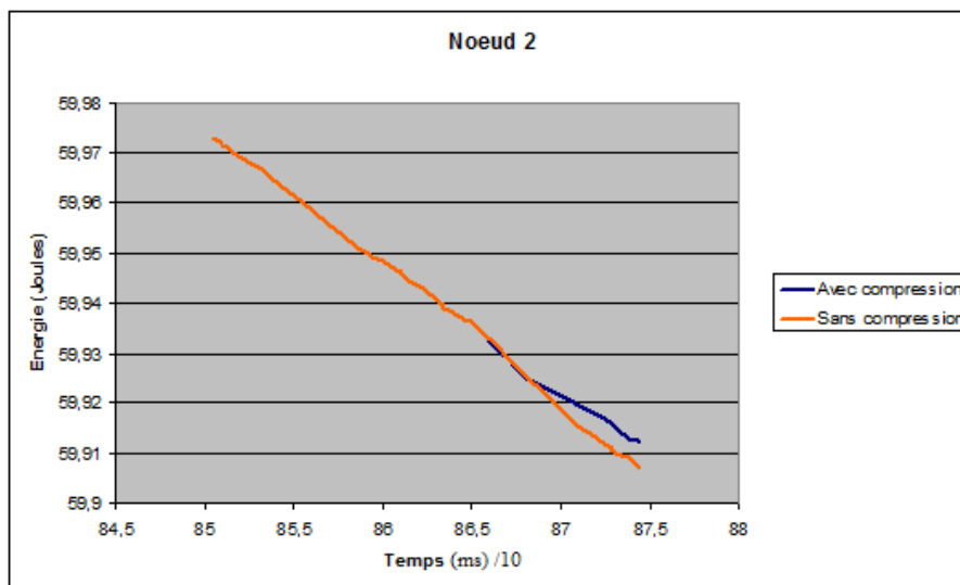
FIGURE 4.22 – Influence de la compression en énergie
