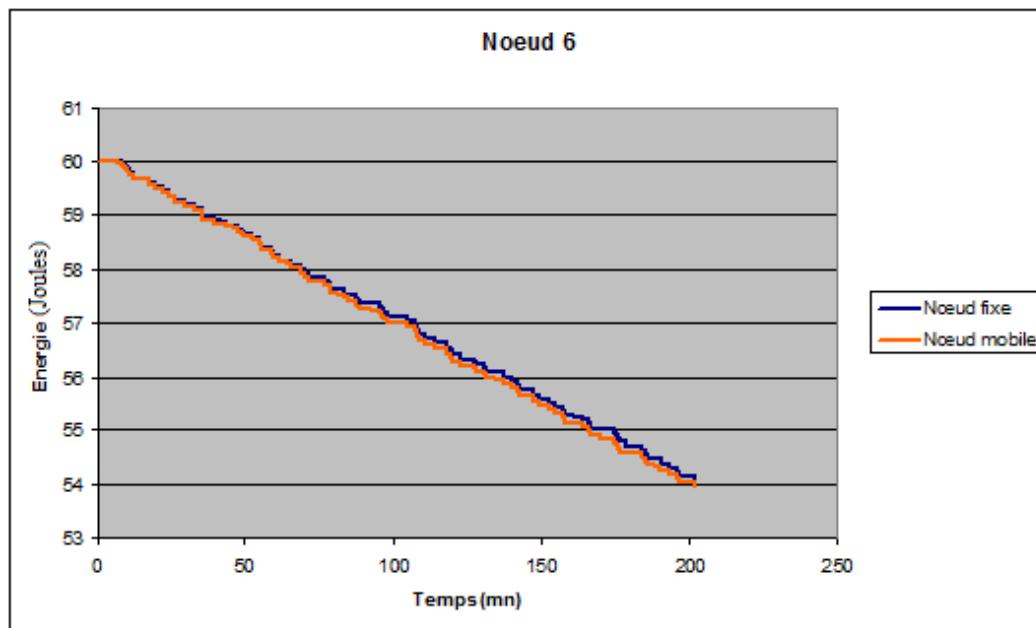
FIGURE 4.13 – Impact de la mobilité d'un noeud
