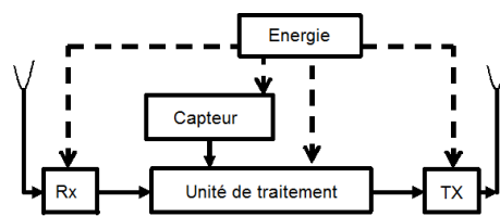
FIGURE 1.4 – Architecture d'un exemple de noeud capteur
