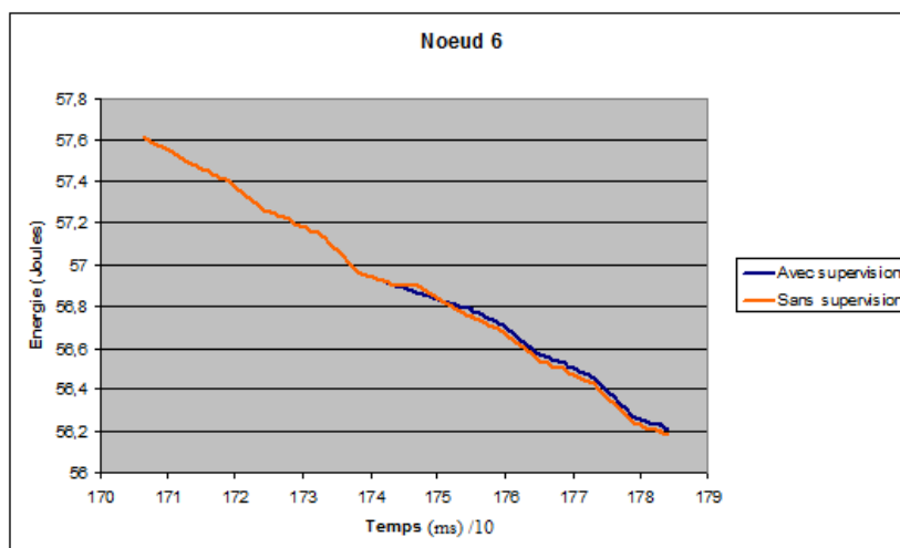
FIGURE 4.18 – Gain en énergie de la fonction supervision
