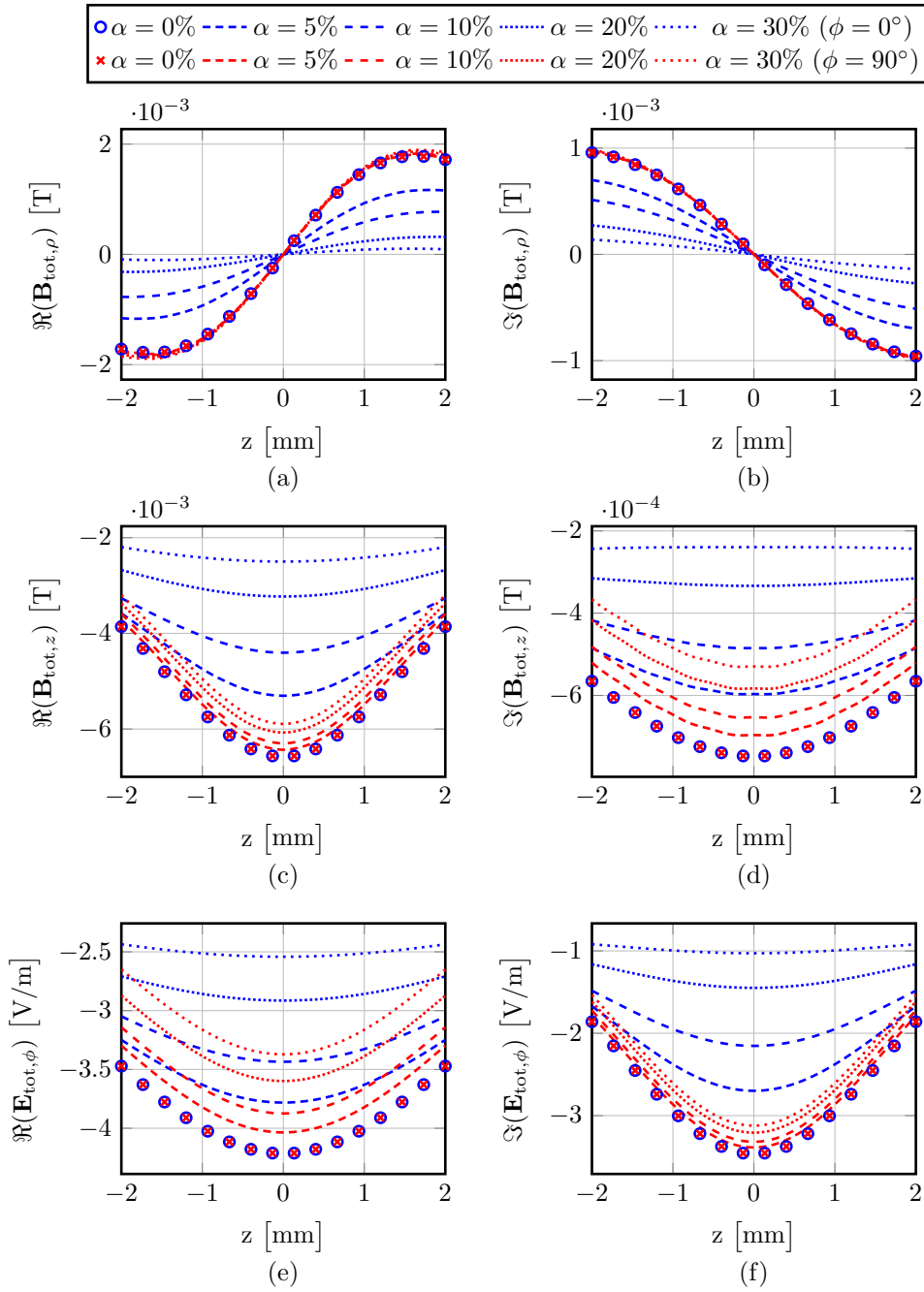
FIGURE 6.27 – Parties réelle (à gauche) et imaginaire (à droite) des composantes des champs électromagnétiques en ( \phi = 0^\circ , \rho = R_x + 0,3 mm) et en ( \phi = 90^\circ , \rho = R_y + 0,3 mm) pour un tube à section elliptique (cas test #5 avec \sigma_1 = 1 MS/m et N_{elem} = 2640 ) à une fréquence f = 100 kHz).
