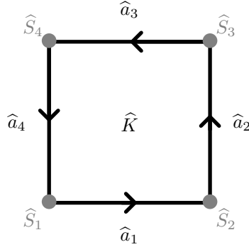
FIGURE 4.1 – Sommets et arêtes sur l'élément de référence \widehat{K} .
