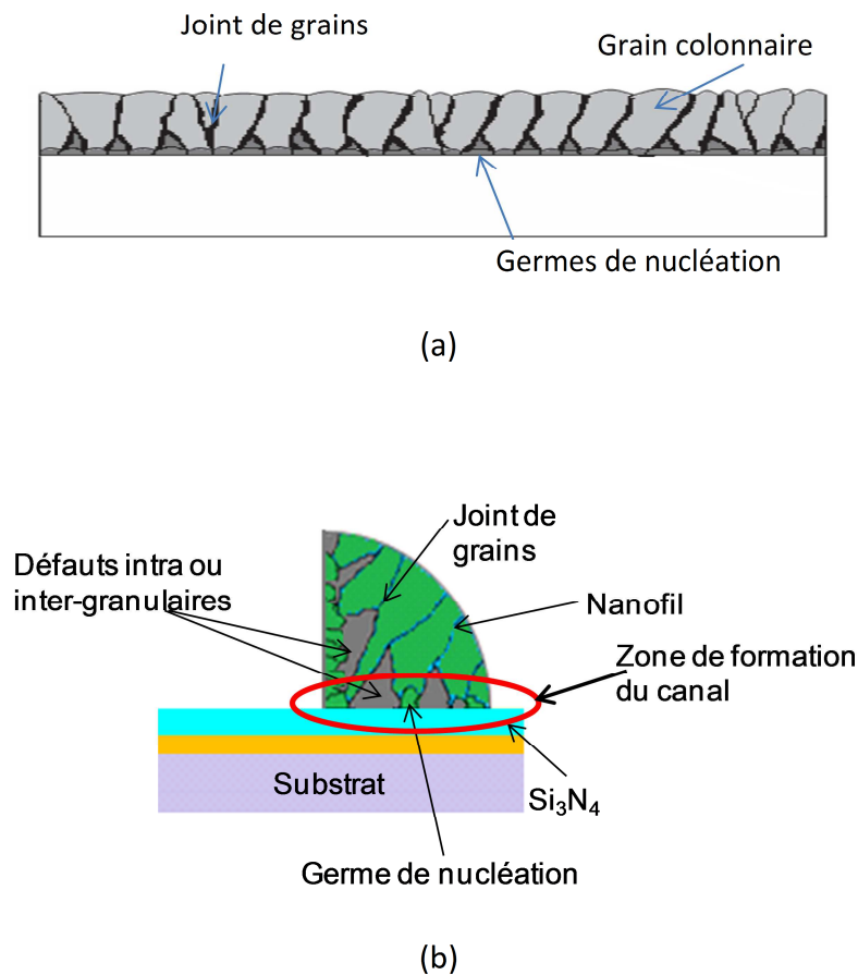
Figure 74 : (a) Structure colonnaire d'une couche de silicium polycristallin déposé par la technique LPCVD, (b) vue en coupe schématique d'un nanofil.
