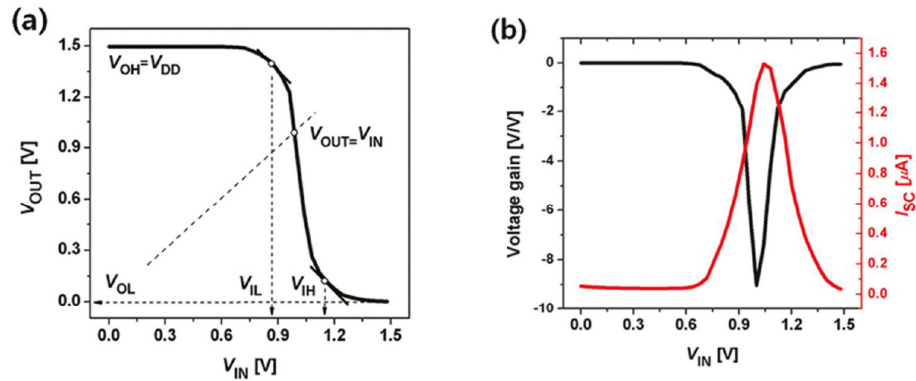
Figure 50 : Caractéristiques en statique d'un inverseur à nanofils de silicium (a) caractéristique de transfert en statique, gain de tension et courant d'alimentation en fonction de la tension d'entrée avec V_{DD} = 1.5 V (b) [61].
