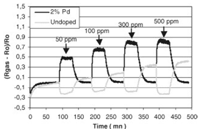
Figure 11 : Réponse d'un capteur à oxyde métallique sous l'influence du CO à une température de 450°C [24].
