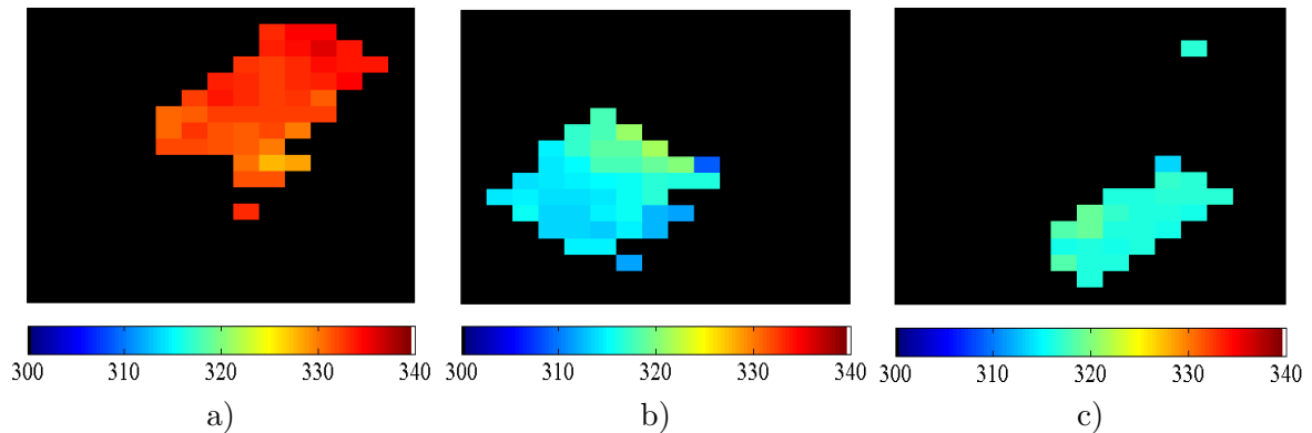
FIGURE 5.11 – Estimation des trois cartes de températures subpixelliques en K pour l’asphalte (a), le gravier (b) et le Bakélite (c).
