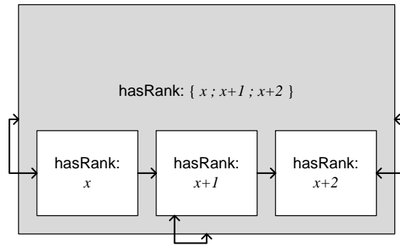
FIGURE 7.5 – Relations dans le cas d'une inclusion multiple entre une case contenant (en gris) et un ensemble de cases contenues (en blanc). Les flèches représentent les relations hasNextPanel établies entre les cases.
