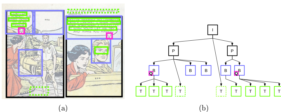
FIGURE 6.6 – Validation des hypothèses respectant les contraintes de notre conceptualisation. Les éléments validés sont en traits continus.
