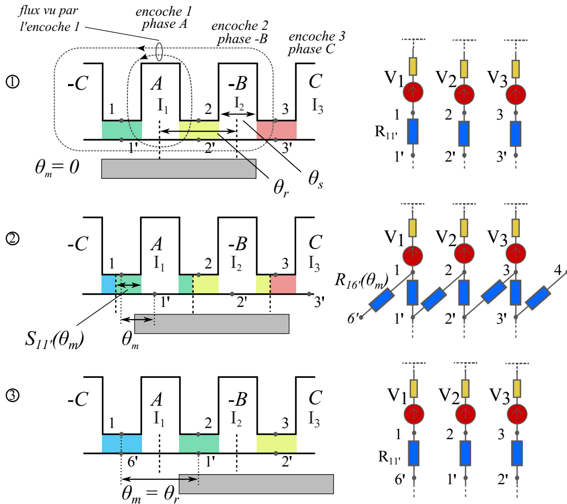
FIGURE II.22 – Représentation de la méthode avec réductances d'entrefer paramétrées
