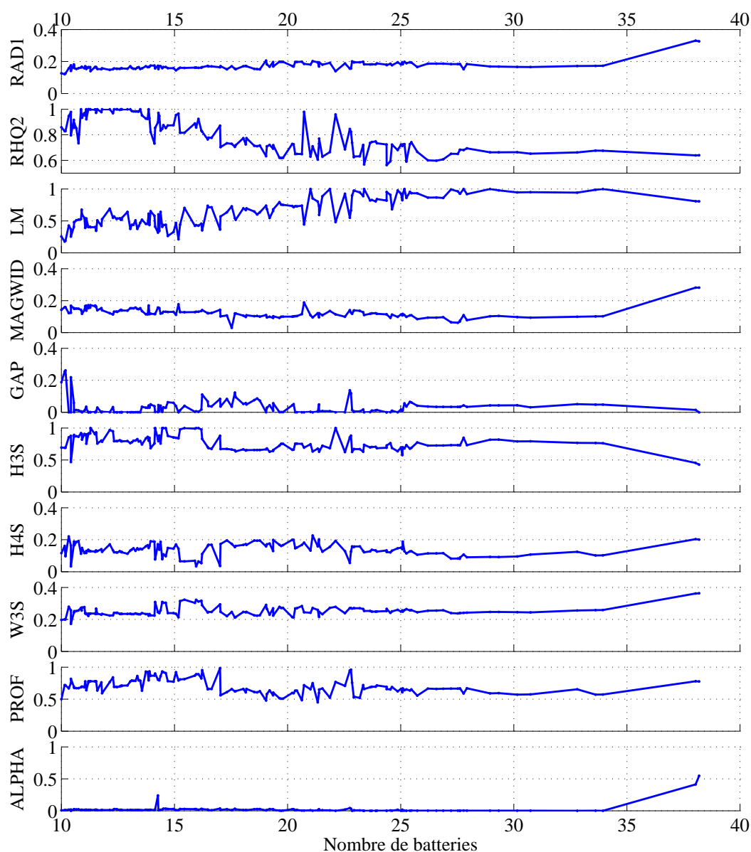
FIGURE IV.19 – Représentation des dimensionnements non dominés normalisés du moteur électrique en fonction du nombre de batteries - cycle Hyzem routier - méthode \mathcal{M}_1
