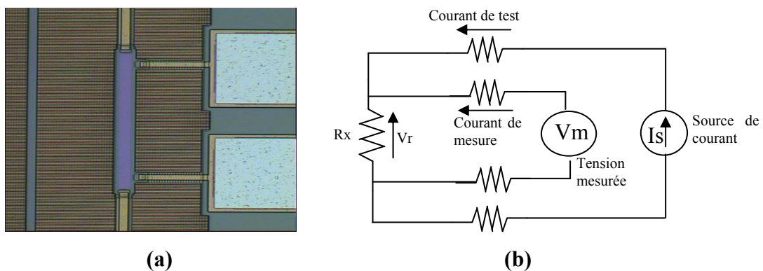
Fig. 4-12- (a) Résistance Kelvin composée de 16 carrés de 10 x 10µm, et (b) Principe de la mesure Kelvin ou quatre points
