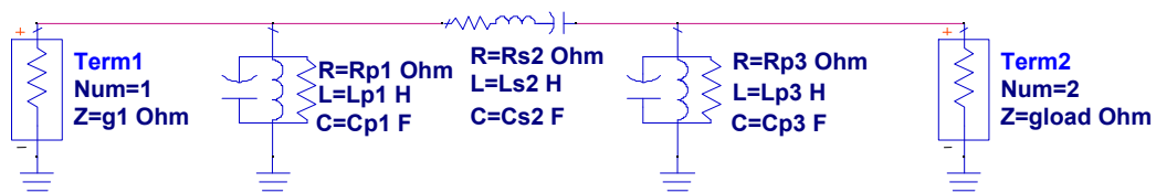
Fig. 1-5 – Filtre du troisième ordre de Tcheychev
