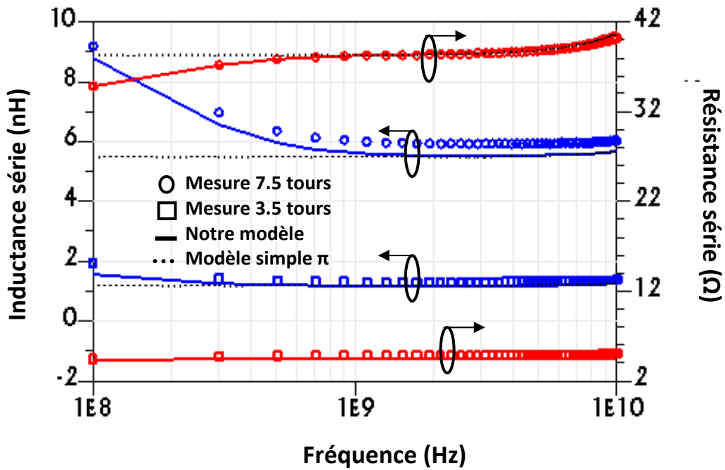
Fig.5-15 - Comparaison entre données mesurées et modélisées à partir du modèle d'échelle développé et celui précédemment proposé par [134]) pour l'inductance équivalente série L_{series}(\omega) et la résistance équivalente série R_{series}(\omega) pour des inductances de 7.5 tours, avec w=3\mu\text{m} , s=2.5\mu\text{m} et d_{out}=145\mu\text{m} , et 3.5-tours avec w=12\mu\text{m} , s=2.5\mu\text{m} et d_{out}=145\mu\text{m} .
