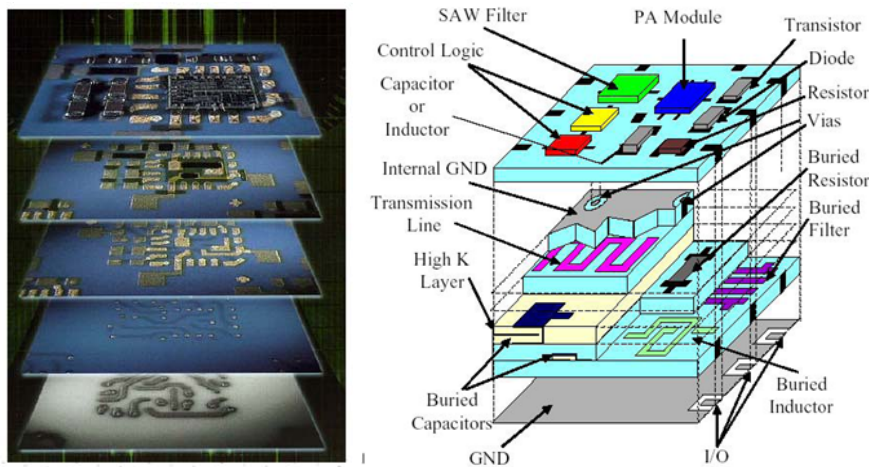
Fig. 2-2 - Exemple de circuit LTCC multicouche
