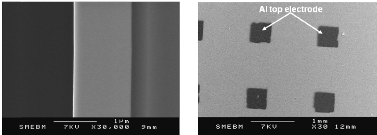
Fig. 3-6 - Image MEB (a) Vue en coupe d'une couche de Ti_{0,28}Ta_{0,19}O de 500nm et (b) Vue de la surface des plots d'aluminium déposés par évaporation
