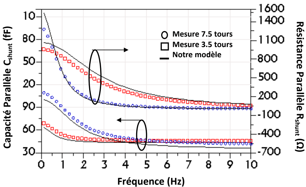
Fig. 5-16 - Comparaison entre données mesurées et modélisées à partir du modèle d'échelle développé et celui précédemment proposé par [134]) pour la capacité équivalente parallèle C_{shunt}(\omega) et la résistance équivalente parallèle R_{shunt}(\omega) pour des inductances de 7.5 tours avec w=3\mu\text{m} , s=2.5\mu\text{m} et d_{out}=145\mu\text{m} , et 3.5-tours avec w=12\mu\text{m} , s=2.5\mu\text{m} and d_{out}=145\mu\text{m} .
