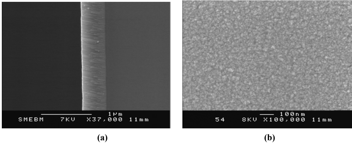
Fig. 4-9- (a) Vue en tranche et (b) de la surface d'une couche de TiN_{0.85}O_{0.68} déposée à 350^{\circ}C
