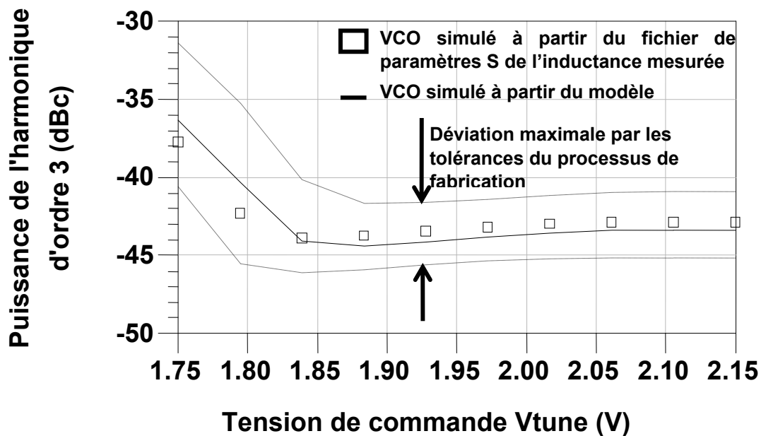
Fig.5-19 – Puissance de l'harmonique d'ordre 3 simulée des VCOs avec : comme référence la réponse du VCO implantée à partir des fichiers de paramètres S mesurés, modélisés, et ceux des inductances simulées en 3D qui tiennent compte des variations maximales induites par le processus de fabrication
