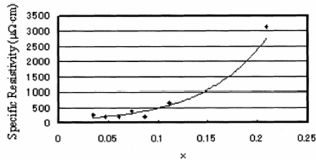
Fig. 4-1 : Résistivité en fonction de la fraction d’oxygène (x) dans le film
