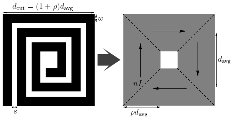
Fig. 5-5 – Approximation de l'inductance comme un anneau symétrique formé de conducteurs infiniment plats et parcourus par des courants uniformes
