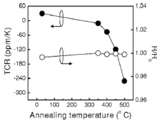
Fig. 4-4 : TCR et R/R 0 en fonction de la température de recuit [129]
