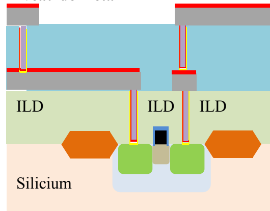
Fig. 2-15- Etapes de formation des niveaux de PLUGS 2 et de Métal M2 de la filière CMOS 0.5µm
