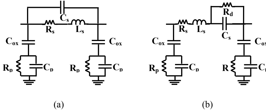
Fig. 1-14 - Modèle en \pi (a) d'inductances et (b) condensateurs intégrés en technologie CMOS
