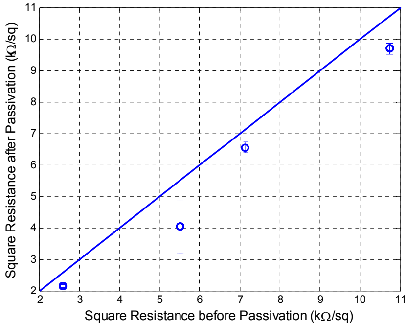
Fig. 4-16- Densité de résistance avant et après l'étape de passivation
