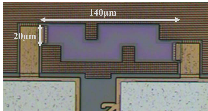
Fig. 4-10- Résistance intégrée composée de 10 carrés de 20\mu m \times 20\mu m en serpentins
