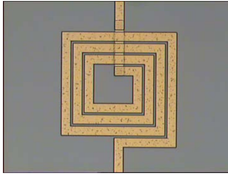
Fig. 5-1 – Image effectuée au microscope optique d’inductances spirales réalisées en technologie CMOS 0.5 \mu m
