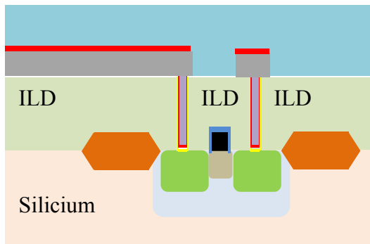
Fig. 2-15- Etapes de formation des niveaux de PLUGS 2 et de Métal M2 de la filière CMOS 0.5µm
