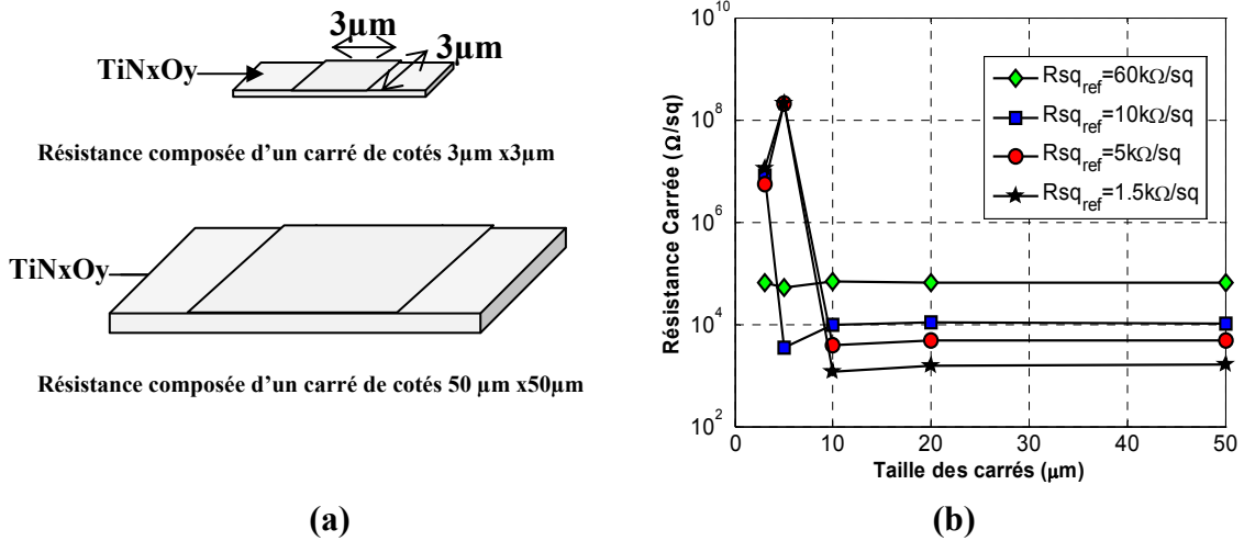
Fig. 4-20- (a) Illustration du test de la taille des carrés et (b) R_{sq} en fonction de la taille des carrés
