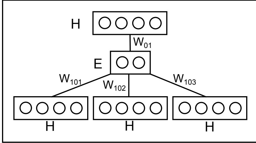
FIGURE 6.3 – Autoencodeur discriminant multi-classes, illustration pour 3 classes.
