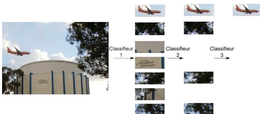
FIGURE 2.3 – Principe d’une cascade de classifieur. Chaque étage de la cascade retire des exemples négatifs.
