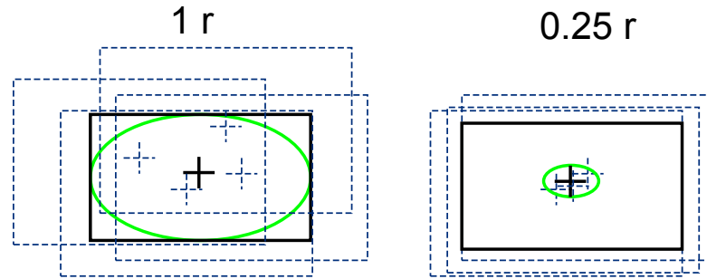
FIGURE 4.3 – Un véhicule et les fenêtres déclarées positives, en utilisant toutes les fenêtres dans un rayon 1r (à gauche) ou rayon 0.25r (à droite), r étant le rayon de l'ellipse dans un axe donné.
