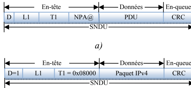
b) Exemple d'encapsulation ULE pour un paquet IPv4
