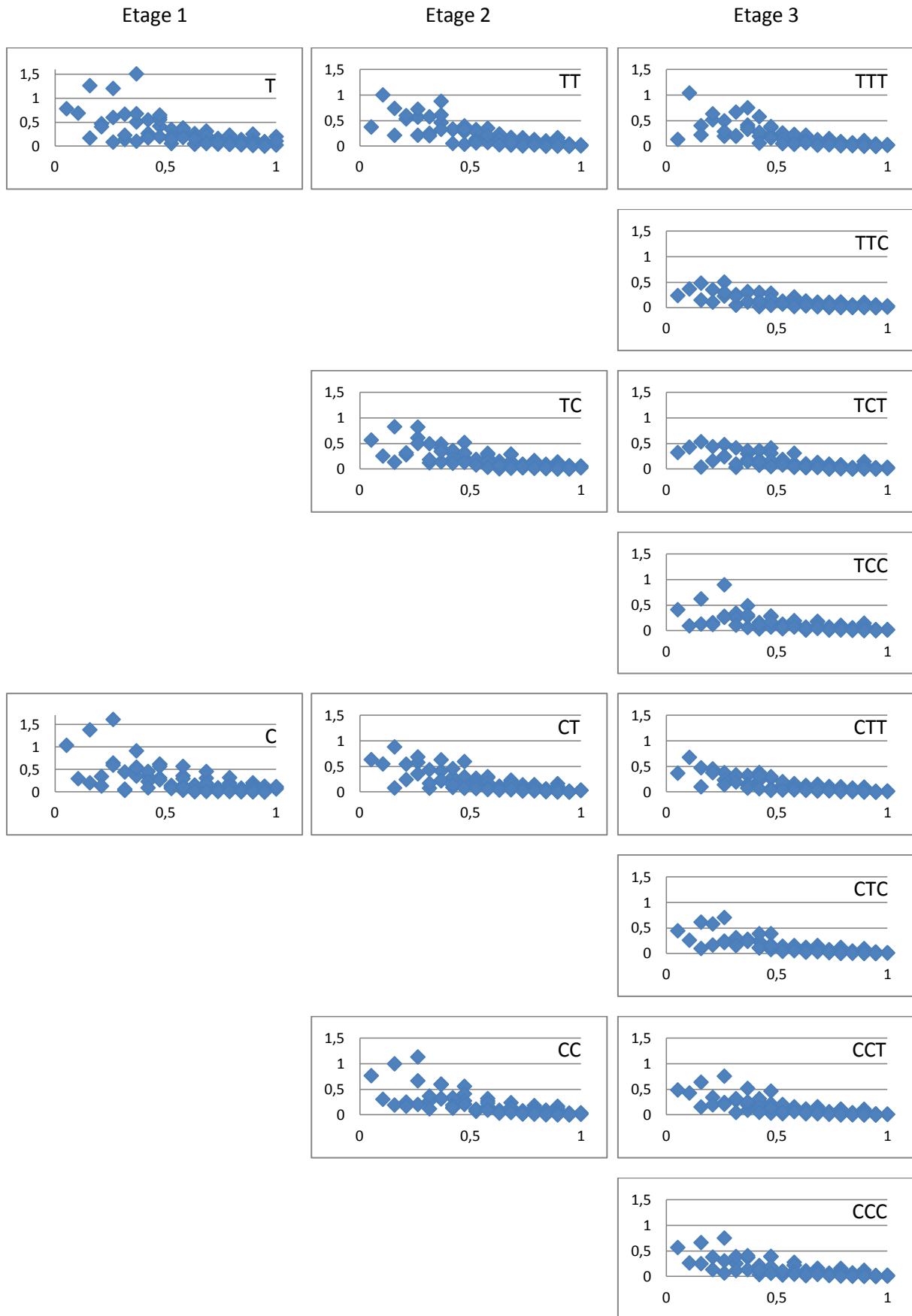
Figure 152 : Module des amplitudes complexes des champs dans le coupleur N×N, pour un champ incident annulaire
