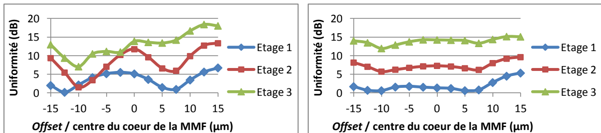
Figure 162 : Uniformité de la puissance en sortie des coupleurs 2x2, 4x4 et 8x8, pour un champ d'entrée gaussien à base elliptique ( X = 6 ; Y = 2 ) avec différents offsets par rapport au cœur de la MMF, à 850 (gauche) et 1300 nm (droite)
