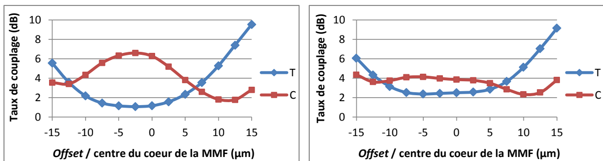
Figure 161 : Pertes d'insertion du coupleur 2x2, pour un champ d'entrée gaussien à base elliptique ( X = 6 ; Y = 2 ), avec différents offsets suivant X par rapport au cœur de la MMF, à 850 (gauche) et 1300 nm (droite)
