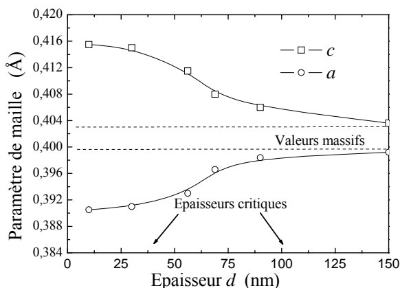
Figure II-31 : Variation des paramètres de maille pour des couches épitaxiées de BaTiO 3 de différentes épaisseurs [II-58]
