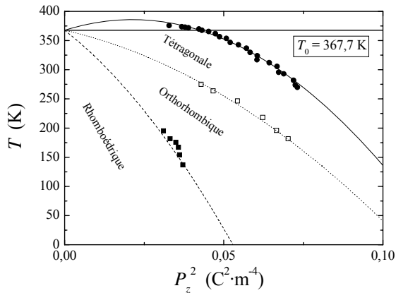
Figure II-17 : Polarisation P_z^2 pour les différentes phases polaire de \text{BaTiO}_3 en fonction de la température T . Comparaison avec l'expérience (Vieder [II-25] et Chynoweth [II-23])
