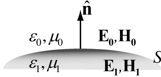
FIGURE 1.1 – Représentation des champs électromagnétiques au niveau de l'interface délimitant deux milieux LHI semi-infinis.
