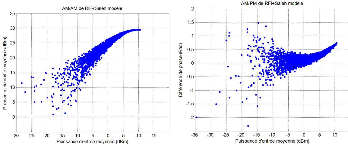
(a) Caractéristique AM/AM de l'AP simulé (RIF-Saleh modèle) (b) Caractéristique AM/PM de l'AP simulé (RIF - Saleh modèle)
