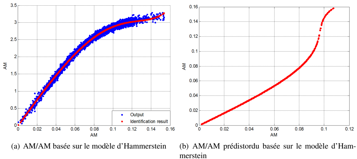
Figure 5.17 – Modélisation/Prédistorion basée sur le modèle d'Hammerstein avec la puissance moyenne d'entrée de -11 dBm
