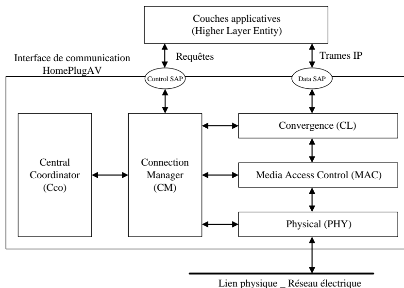
Figure 4.2 – Organisation des dispositifs supportant le protocole HPAV.
