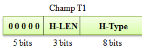
Figure 2.6. Structure du champ TI pour indiquer un entête d'extension ULE
