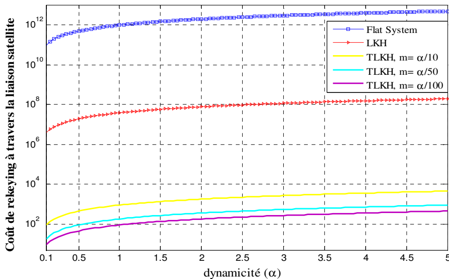
Figure 2.25. Co t de rekeying   travers la liaison satellitaire dans les diff rents syst mes
