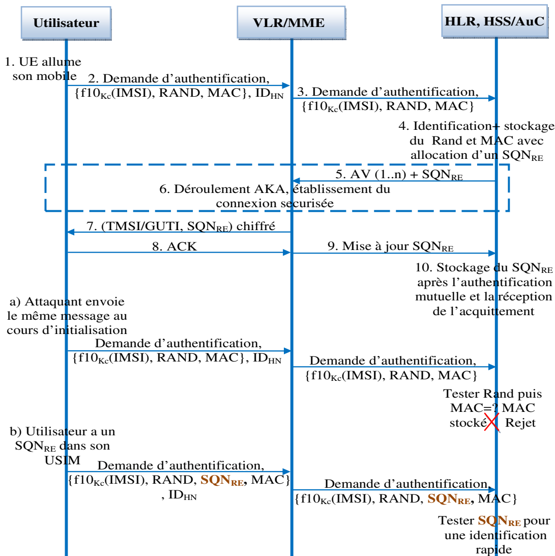
Figure 4.7. Détection rapide des attaques par le SQN_{RE}
