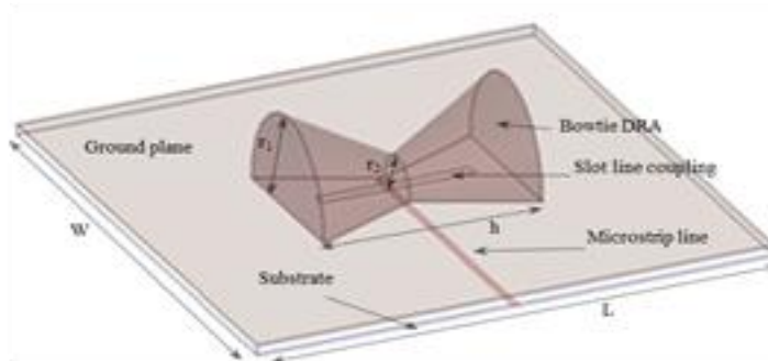
Figure 3.28. Structure d'une antenne Papillon
