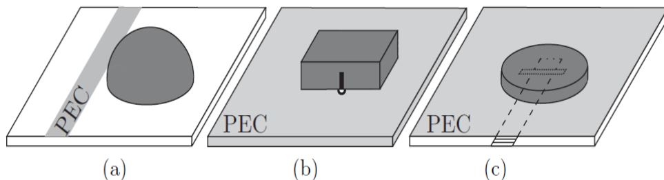
Figure 2.1. Configurations d'ARD les plus populaires : (a) ARDH couplée par une ligne microruban, (b) ARDR couplée par une sonde coaxiale et (c) ARDC couplé à travers une fente.
