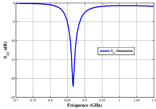
Figure 5.30. Coefficient de réflexion simulé de la structure en présence de la couche de métamatériaux
