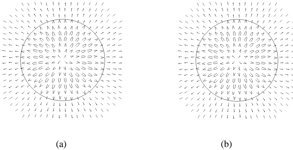
Figure 2.4. Cartes de champs du mode TE_{01\delta} : (a) distribution du champ magnétique, (b) distribution du champ électrique
