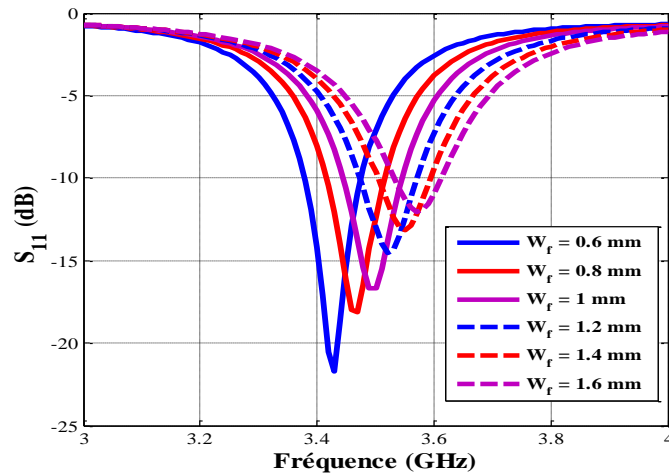
Figure 2.21. Influence de la largeur de la fente W_f sur la fréquence de résonance
