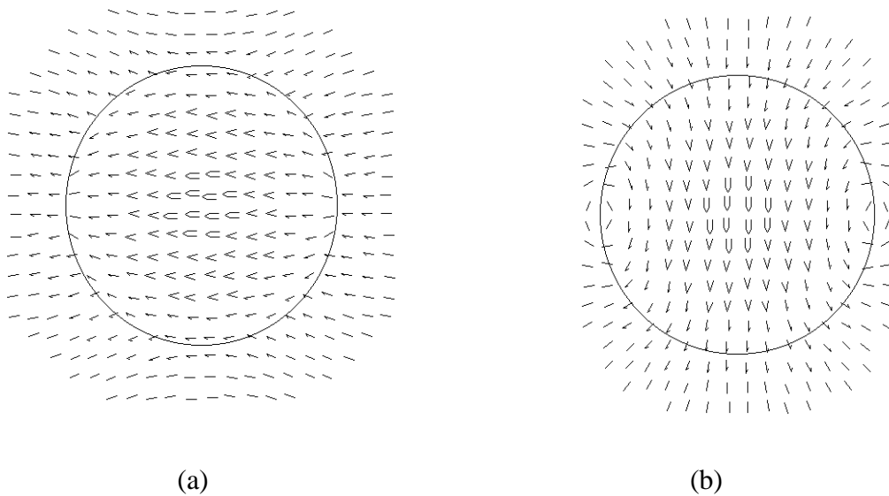
Figure 2.5. Cartes de champs du mode HEM_{11\delta} : (a) distribution du champ magnétique et (b) distribution du champ électrique.
