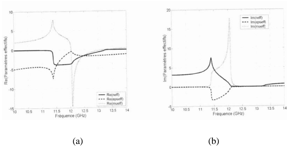
Figure 5.27. Indice de réfraction ( n_{eff} ), permittivité ( \epsilon_{seff} ) et perméabilité ( \mu_{seff} ) effectifs du matériau main gauche simulé - (a) partie réelle « Re » (b) partie imaginaire « Im »
