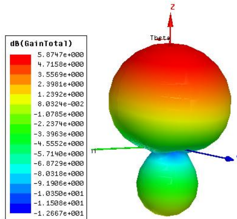
Figure 5.32. Variation du gain tridimensionnel à la fréquence 866 MHz
