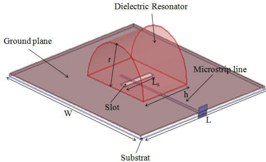
Figure 5.3. Configuration de l'antenne étudiée
