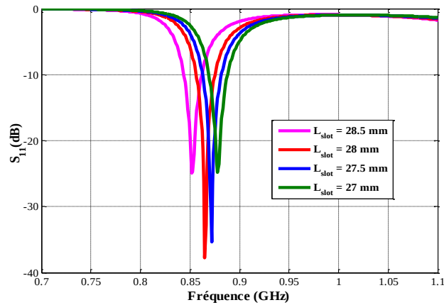
Figure 5.7. Coefficient de réflexion à l'entrée pour différentes valeurs de la longueur de la fente
