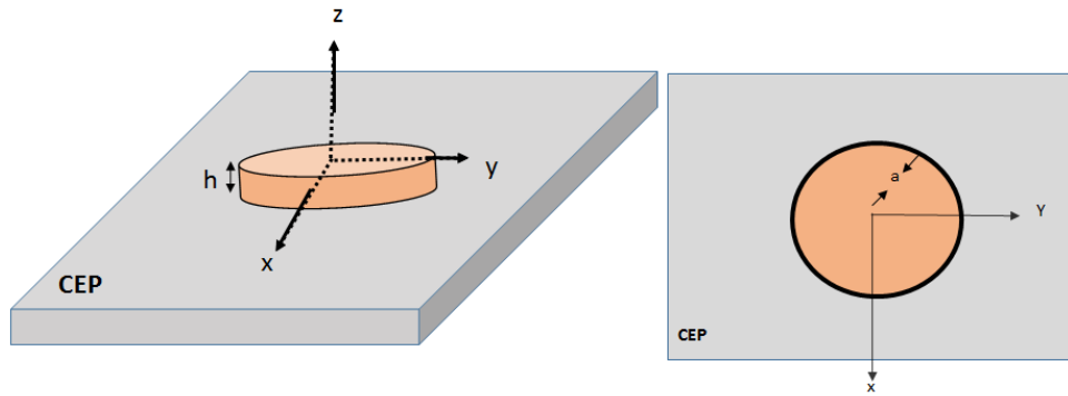
Figure 2.2. Antenne à résonateur diélectrique cylindrique: (a) Vue en 3D, (b) Vue de dessus.
