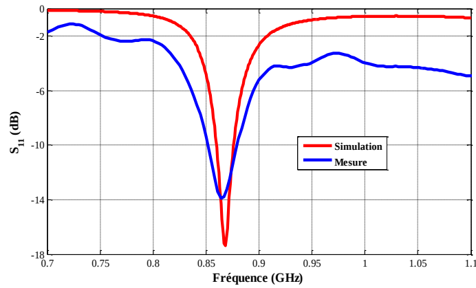
Figure 5.13. Coefficient de réflexion de l'ARDR
