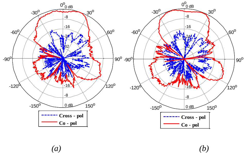
Figure 3.27. Diagrammes de rayonnement mesurés dans les deux plans E et H à 5.5 GHz:
