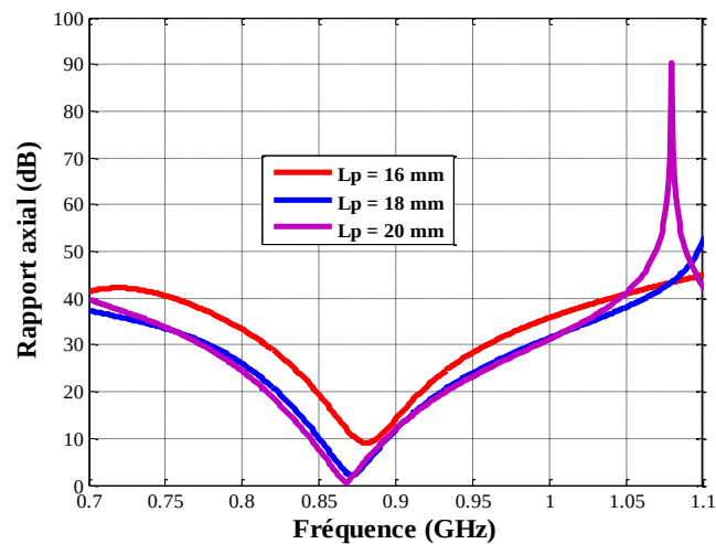
Figure 5.20. Variation du rapport axial en fonction de la longueur de ruban métallique L_p
