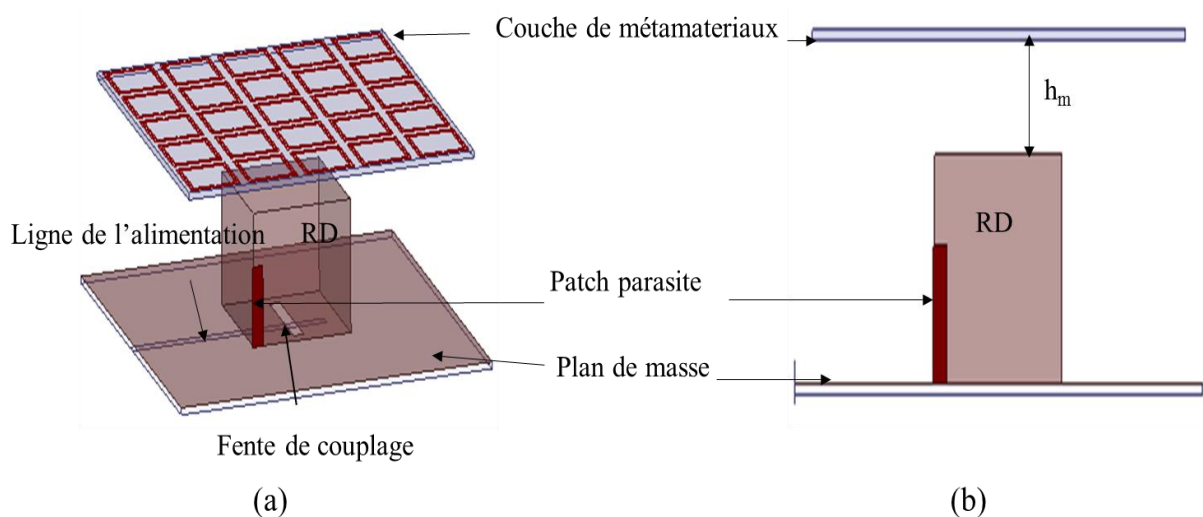
Figure 5.28. Structure de l'antenne étudiée avec une couche de métamatériaux (a) Vue générale, (b) Vue de coté
