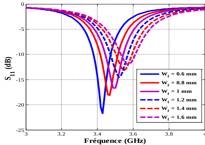
Figure 2.21. Influence du largeur de la fente W_f sur la fréquence de résonance
