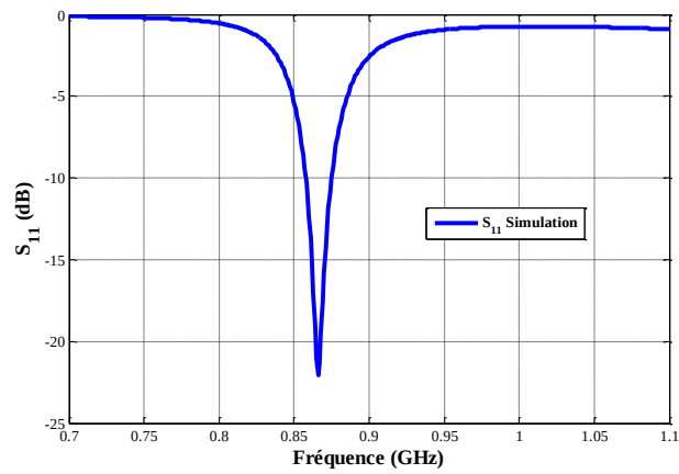
Figure 5.30. Coefficient de réflexion simulé de la structure en présence de la couche de métamateriaux
