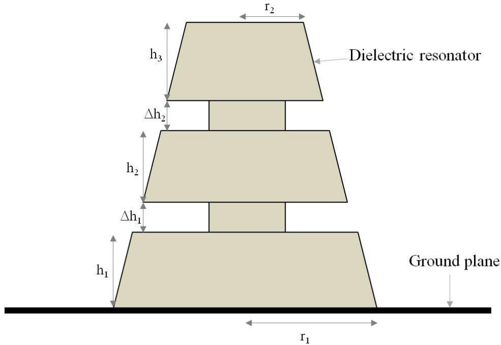
Figure 3.20. Structure de l'antenne Yagi étudiée
