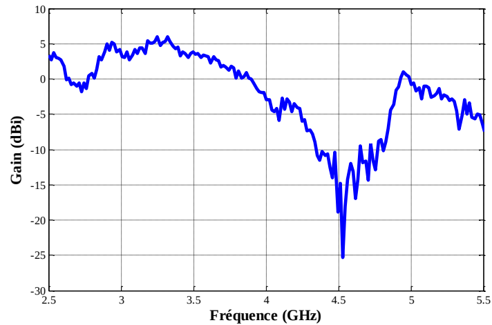
Figure 4.16. Évolution du gain mesuré en fonction de la fréquence
