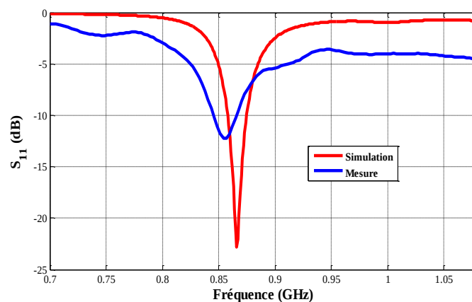
Figure 5.21. Variation fréquentielle du coefficient de réflexion simulé et mesuré
