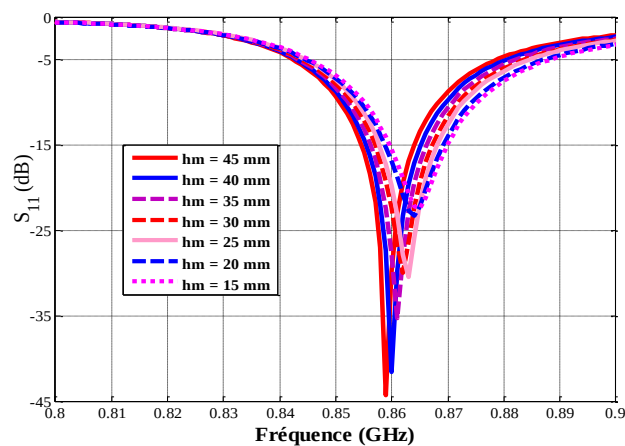
Figure 5.29. Variation de coefficient de réflexion en fonction de la hauteur h_m
