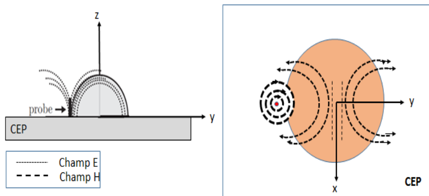
Figure 2.12. Résonateur diélectrique excité par une sonde coaxiale
