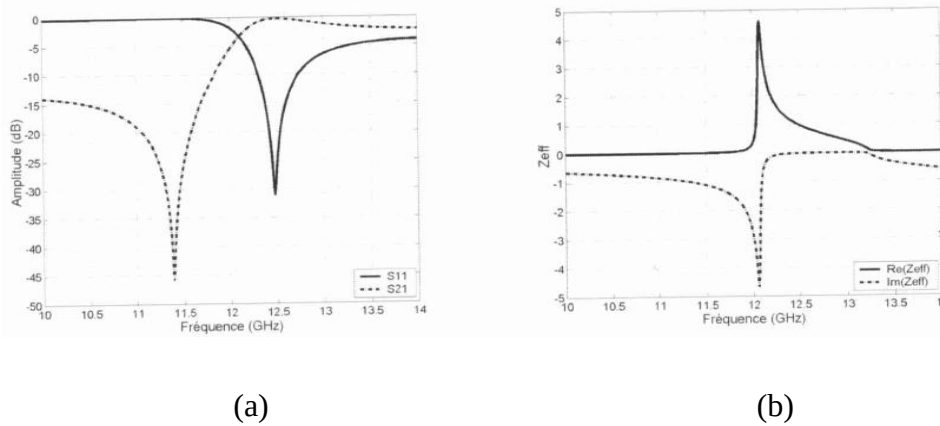
Figure 5.266. (a) Coefficients de réflexion ( S_{11} ) et de transmission ( S_{21} ) simulés sous HFSS (b) Impédance d'onde calculée en utilisant la méthode NRW
