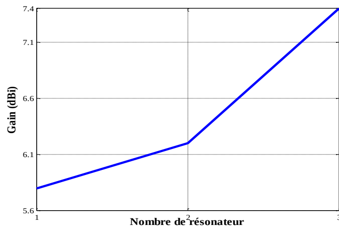
Figure 3.22. Variation du gain de l'antenne en fonction du nombre de résonateurs
