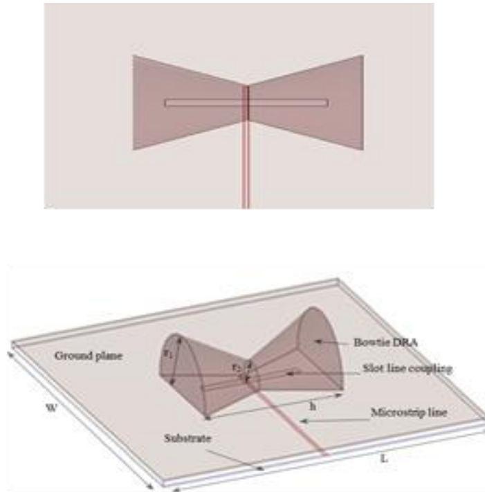
Figure 3.28. Structure d'une antenne Papillon
