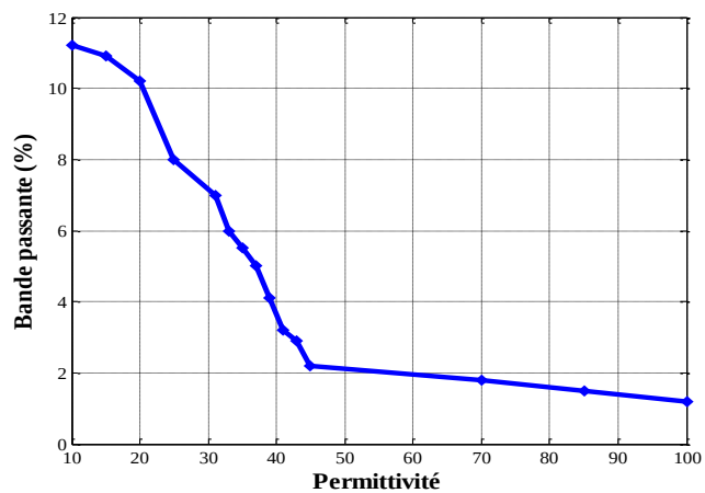
Figure 2.17. Influence de permittivité de résonateur sur la bande passante
