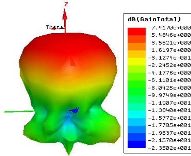
Figure 3.26. Diagramme de gain total en 3D simulé à 5.5 GHz
