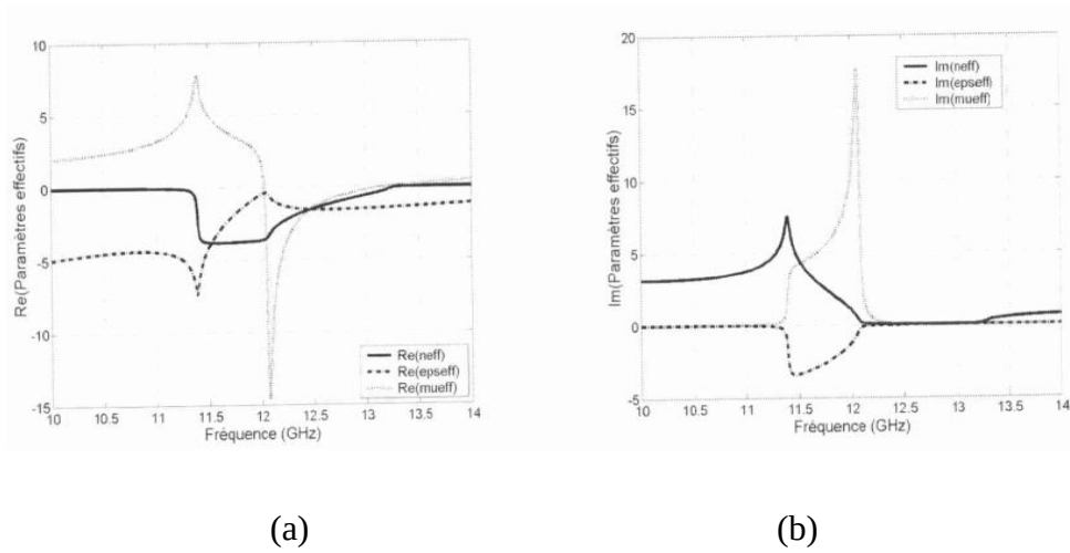
Figure 5.27. Indice de réfraction ( n_{\text{eff}} ), permittivité ( \epsilon_{\text{eff}} ) et perméabilité ( \mu_{\text{eff}} ) effectifs du matériau main gauche simulé - (a) partie réelle « Re » (b) partie imaginaire « Im »
