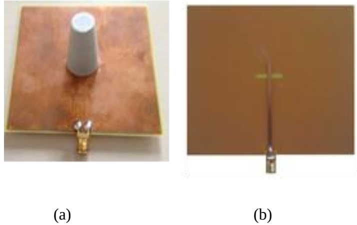
Figure 3.7. Prototype de l'antenne réalisée: (a) Vue générale; (b) Vue de dessous
