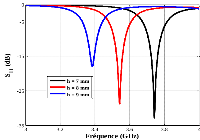
Figure 2.19. Variation de la fréquence de résonance en fonction de la hauteur ( h )
