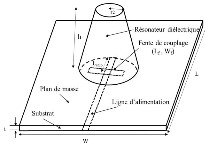
Figure 3.4. Structure de l'antenne conique
