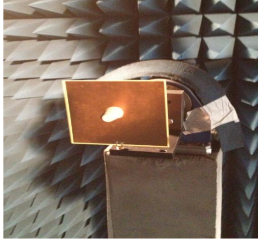
Figure 3.23. Mesures de l'antenne dans la chambre anechoïde de l'ESEO
