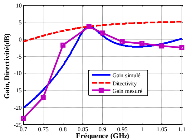
Figure 5.10. Evolution du gain et de la directivité en fonction de la fréquence
