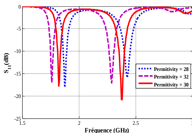
Figure 4.3. Variation du coefficient de réflexion de l'antenne en fonction de la valeur de permittivité
