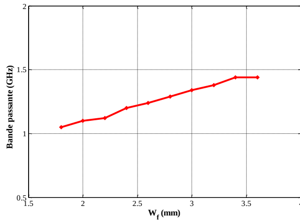
Figure 3.30. Variation de bande passante en fonction de la largeur de la fente W_f
