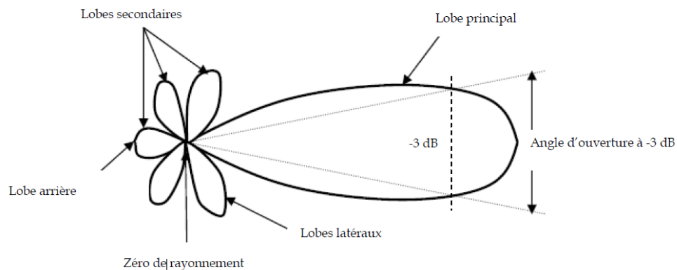
Figure 1.7. Diagramme de rayonnement d'une antenne directive
