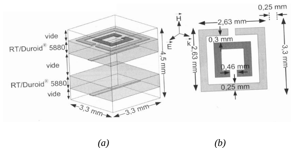
Figure 5.25. (a) Cellule élémentaire du matériau main gauche - (b) dimensions du SRR et des tiges métalliques
