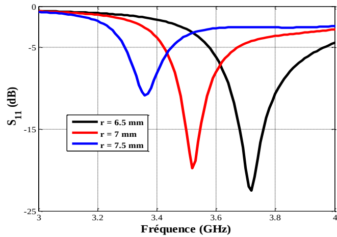
Figure 2.18. Variation de la fréquence de résonance en fonction du rayon ( r )
