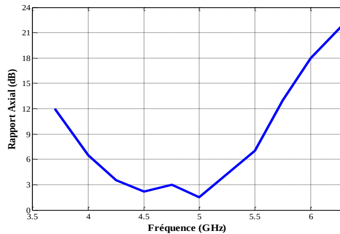
Figure 3.18. Rapport axial mesuré
