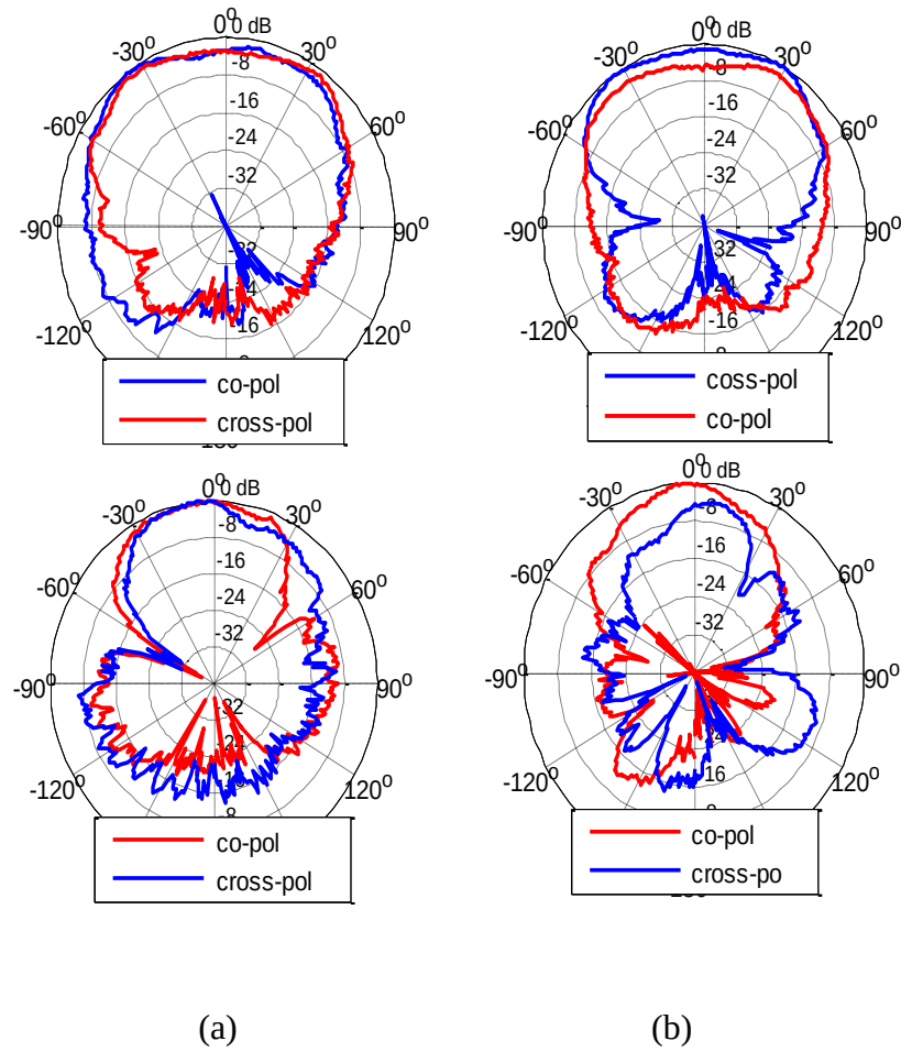
Figure 3.19. Diagramme de rayonnement de l'antenne réalisée dans les deux plan E (a) et H (b) à 4.3 et 5 GHz
