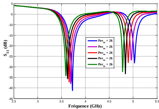
Figure 4.11. Variation du paramètre S_{11} en fonction de la permittivité du résonateur intérieur
