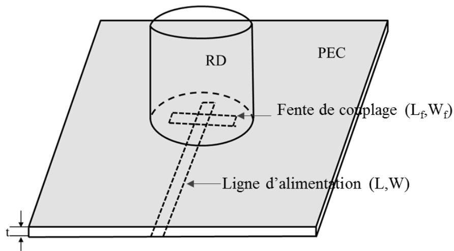
Figure 3.1. Antenne à résonateur diélectrique cylindrique
