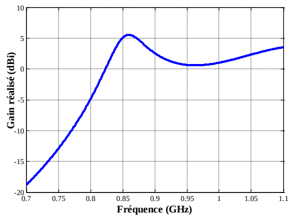
Figure 5.31. Variation du gain simulé en fonction de la fréquence
