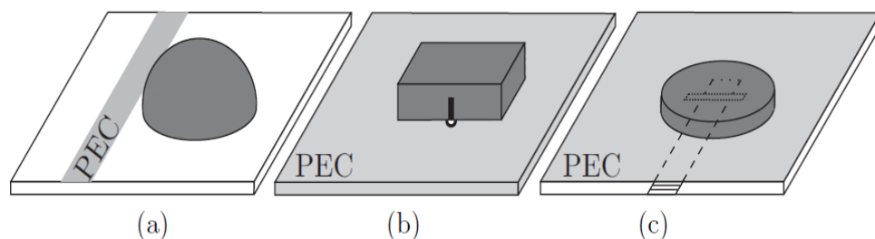
Figure 2.1. Configurations d'ARD les plus populaires : (a) ARDH couplée par une ligne microruban, (b) ARDR couplée par une sonde coaxiale et (c) ARDC couplée à travers une fente.
