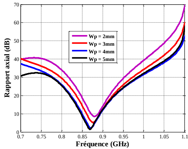
Figure 5.18. Variation du rapport axial en fonction de la largeur de ruban métallique W_p
