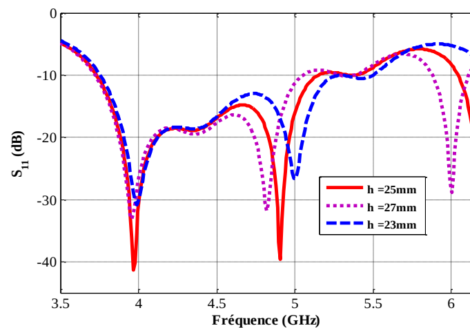
Figure 3.6. Coefficient de réflexion pour différentes valeurs de la hauteur du résonateur
