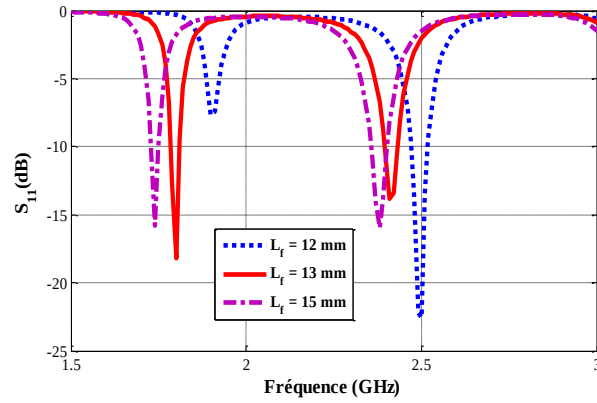
Figure 4.4. Variation du coefficient de réflexion de l'antenne en fonction de la longueur de la fente L_f
