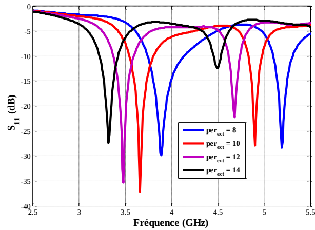
Figure 4.12. Variation du paramètre S_{11} en fonction de la permittivité du résonateur intérieur
