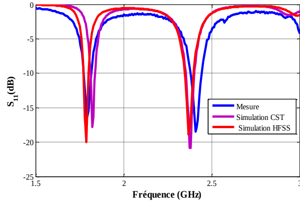
Figure 4.7. Comparaison entre la simulation et la mesure du coefficient de réflexion de l'antenne
