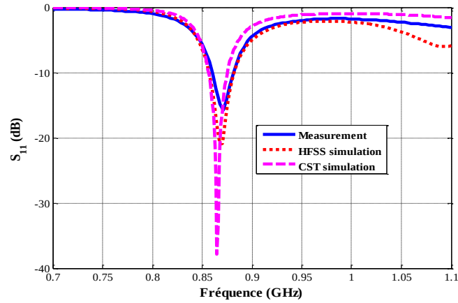
Figure 5.9. Coefficients de réflexion simulé et mesuré en fonction de la fréquence
