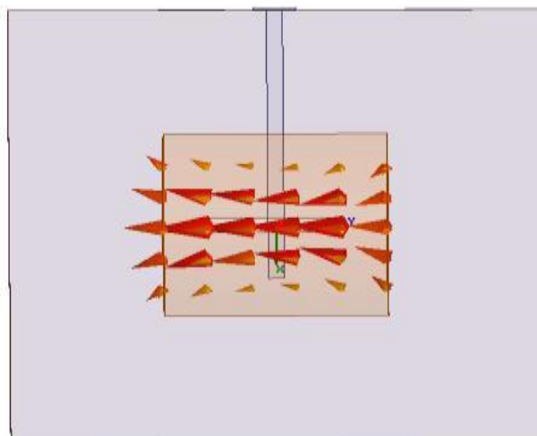
Figure 5.4. Distribution du champ magnétique dans le plan xy
