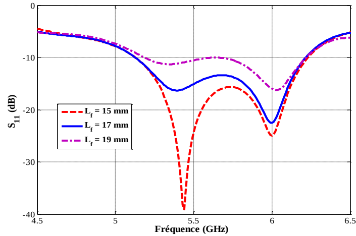
Figure 3.29. Variation du coefficient de réflexion pour différentes valeurs de L_f
