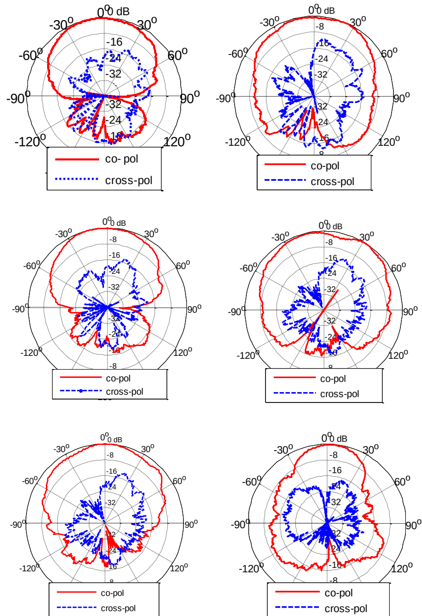
Figure 3.10. Composante principale et croisée du champ mesuré dans les plans E (à gauche) et H (à droite) à 3.7, 4.5 et 5.6 GHz
