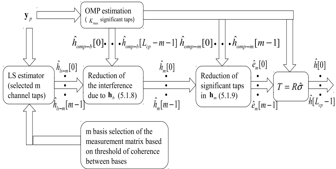
Figure C.5.1: Schéma de l'estimation de canal parcimonieux proposée
