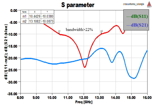
Figure 2.24: S parameters
