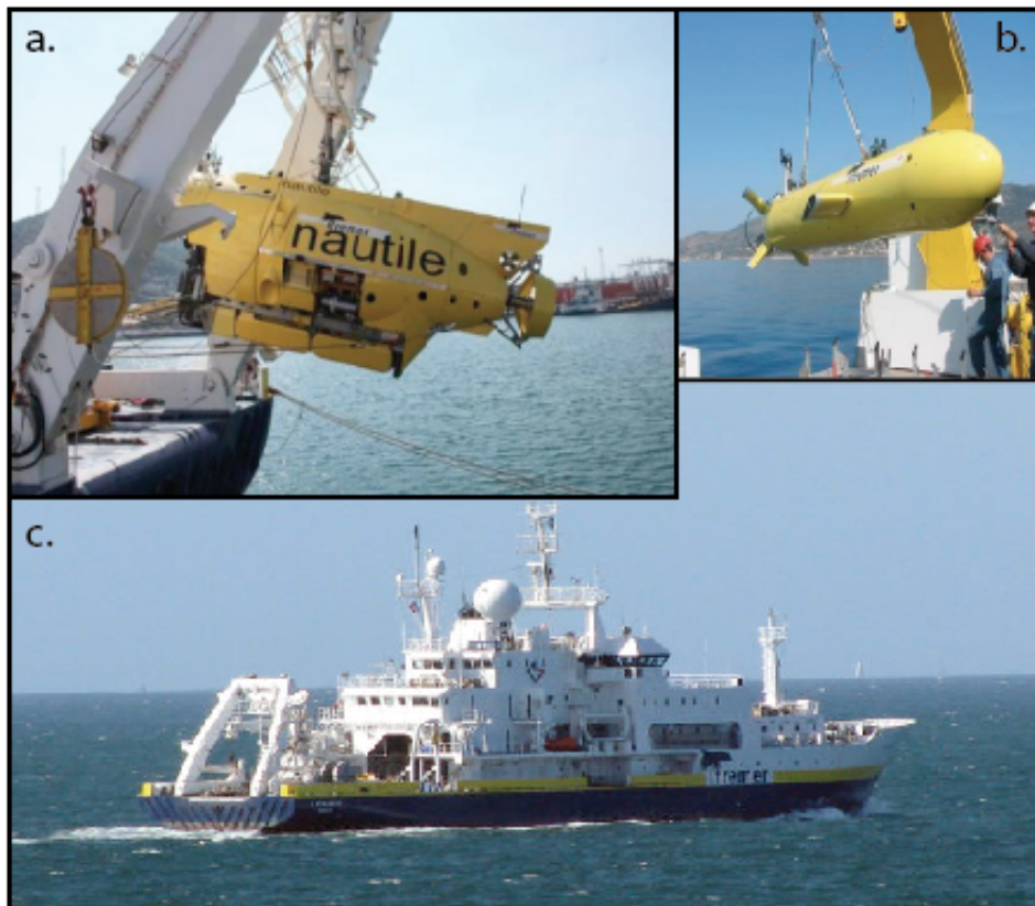
FIGURE 2.4 – Photographies des équipements utilisés lors de la campagne PaRiSub. a) le submersible Nautille, b) l'Autonomous Underwater Vehicle (AUV) AsterX, et c) le navire Océanographique (N/O) l'Atalante.
