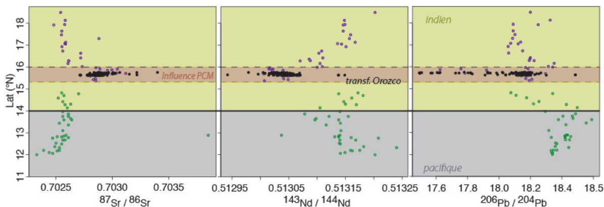
FIGURE 5.7 – Variations des rapports ^{87}\text{Sr}/^{86}\text{Sr} , ^{143}\text{Nd}/^{144}\text{Nd} , et ^{206}\text{Pb}/^{204}\text{Pb} le long de l'EPR entre 11 ° N et 18 ° N. On remarquera l'émergence d'une signature géochimique très singulière entre 15 ° et 16 ° N avec des valeurs de Sr très radiogéniques et des valeurs de Nd et Pb très peu radiogéniques, suggérant une influence du Point Chaud des Mathématiciens (PCM) sur cette portion de l'EPR. Les cercles noirs correspondent aux échantillons analysés dans cette étude ; les cercles verts sont les données de Castillo et al. (2000) ; et les cercles violets, les données extraites de Donnelly (2002).
