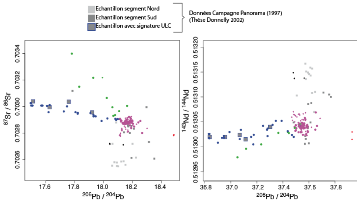
FIGURE 5.17 – Compositions isotopiques des basaltes de l'EPR entre 15^{\circ}20'N et 17^{\circ}40'N . Les ronds désignent les échantillons analysés au cours de cette étude, et les carrés correspondent aux données de la campagne Panorama Leg 1 (1997) (extraites de Donnelly, 2002).
