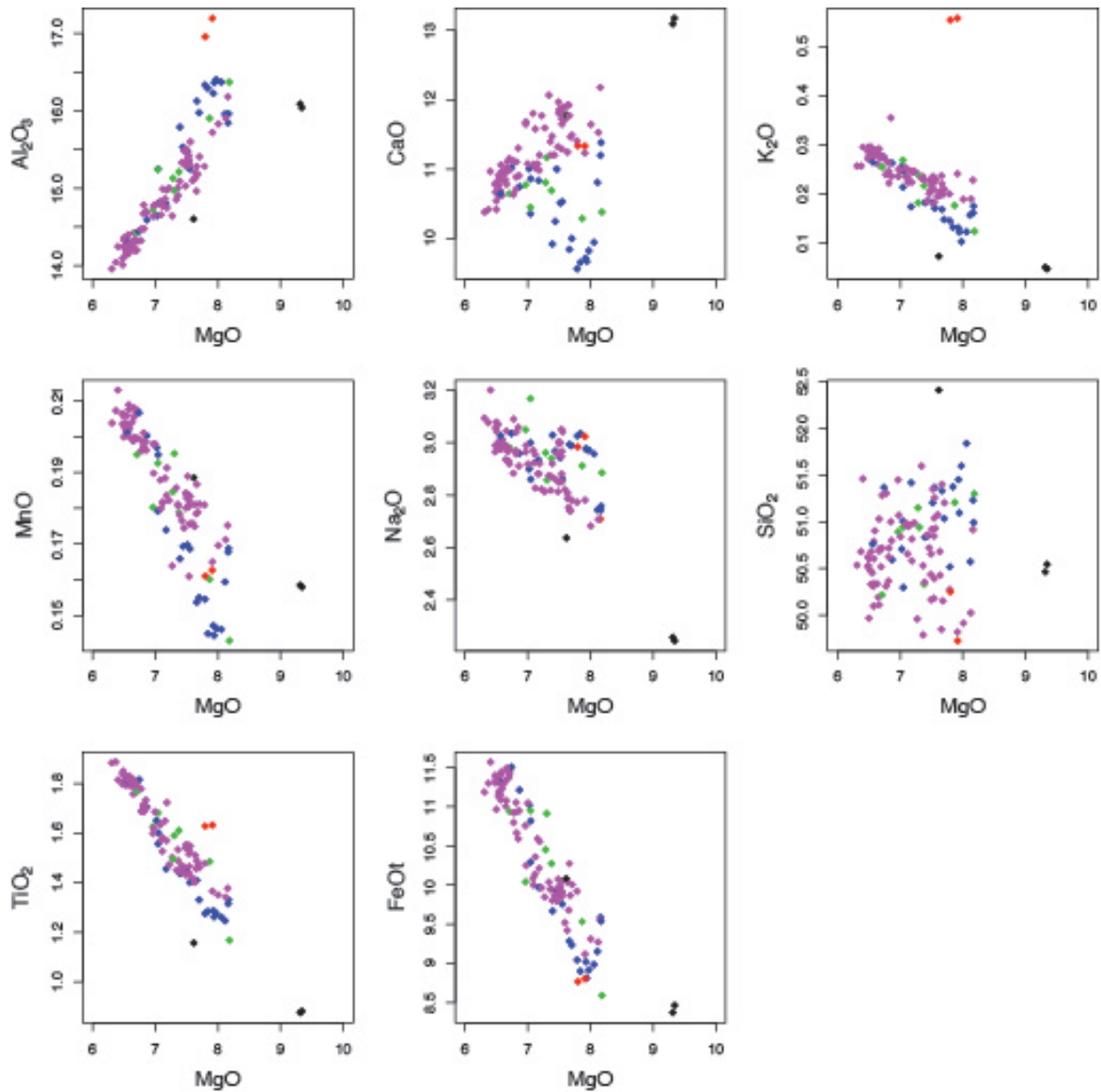
FIGURE 5.11 – Variations des teneurs en \text{Al}_2\text{O}_3 , \text{CaO} , \text{MnO} , \text{Na}_2\text{O} , \text{SiO}_2 , \text{TiO}_2 et \text{FeO} en fonction de \text{MgO} de l'ensemble des échantillons analysés, et identification de leur source mantellique d'après leur composition isotopique. En violet sont représentés les échantillons caractéristiques du manteau ambiant (AM). En vert, les échantillons caractéristiques du mélange entre les composants SMC (Secondary Mathematician Component) et AM, en bleu ceux caractéristiques du mélange entre les composants ULC (Unradiogenic Lead Component) et AM, et en rouge et noir les E-MORB et N-MORB respectivement, identifiés le long du profil transversal. On remarquera que ce sont plutôt les différences de source et les processus de mélange, plus que la cristallisation fractionnée qui semble définir les tendances et la répartition des échantillons dans les diagrammes.
