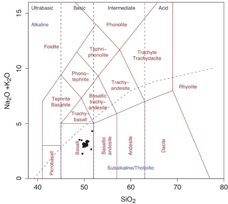
FIGURE 4.9 – Diagramme TAS (Total Alkalis vs Silica d’après Le Bas et Streckeisen, 1991) des échantillons du profil transversal.
