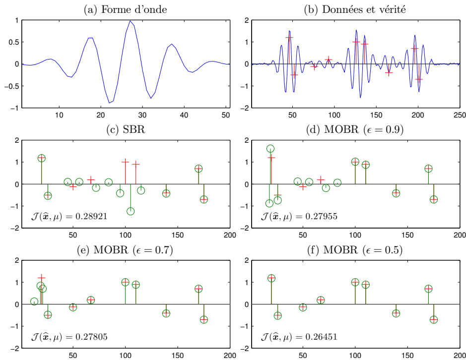
FIGURE 3.12 – Déconvolution par régularisation \ell_0 . (a) : Réponse impulsionnelle instrumentale avec f_0 = 5 MHz, \text{BWR}_{-3} = 0.3 , \phi = -\pi/4 , (b) : données avec \text{RSB} = 25 dB (–) et vérité (+), (c) : vérité (+) et estimation par SBR (○), (d) vérité (+) et estimation par MOBR pour \epsilon = 0.9 (○), (e) : vérité (+) et estimation par MOBR pour \epsilon = 0.7 (○), (f) : vérité (+) et estimation par MOBR pour \epsilon = 0.5 (○).
