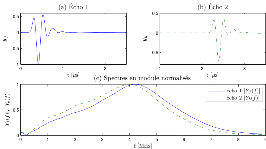
FIGURE 2.20 – Signaux temporels et fréquentiels acquis à partir d'une épaisseur d'huile de ricin de 3 mm avec un transducteur à 5 MHz. (a) : Écho 1 acquis avec la première position du transducteur, (b) : écho 2 acquis avec la deuxième position du transducteur, (c) : spectres en module des deux échos.
