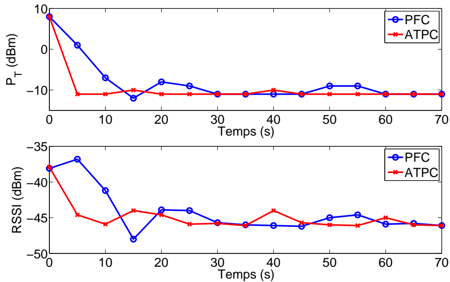
FIGURE 4.14 – Evolution de la puissance émise et du RSSI pour le capteur WS_2 avec la condition initiale de 8dBm
