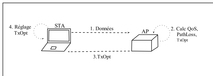
FIGURE 2.2 – L'algorithme TPC pour les WLAN
