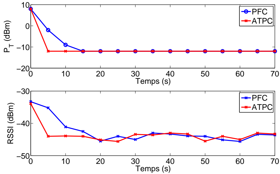
FIGURE 4.13 – Evolution de la puissance émise et du RSSI pour le capteur WS_1 avec la condition initiale de 8dBm
