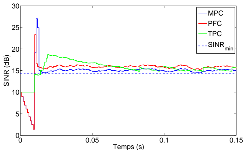
FIGURE 4.3 – Le SINR d’UE avec une vitesse de déplacement de 260\text{km.h}^{-1}
