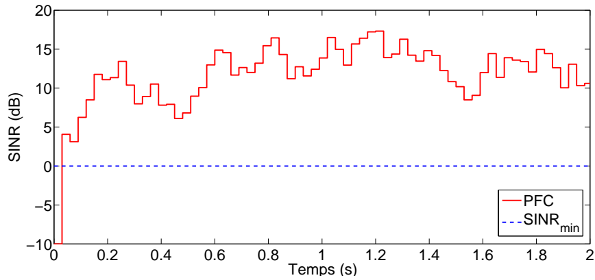
FIGURE 4.8 – SINR avec la commande PFC, k_1 = -0.05
