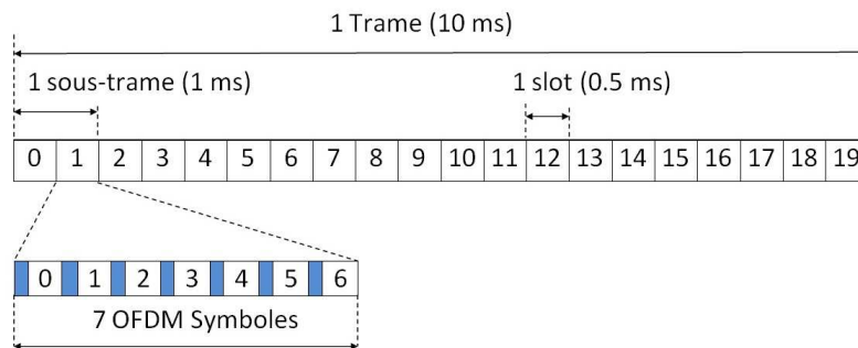
FIGURE 1.2 – Structure d'une trame en LTE
