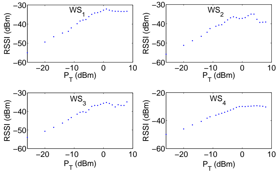
FIGURE 4.12 – RSSI vs puissance de transmission
