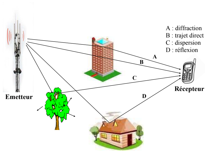
FIGURE 1.10 – Phénomènes de propagation de l'onde radio
