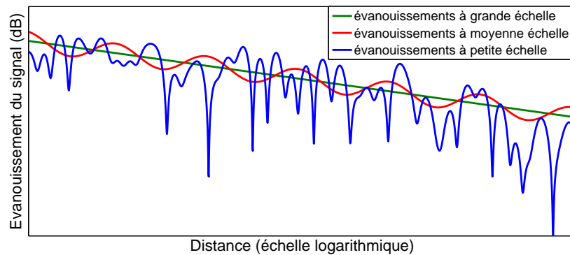
FIGURE 1.11 – Evanouissement du signal reçu dans un canal radio mobile
